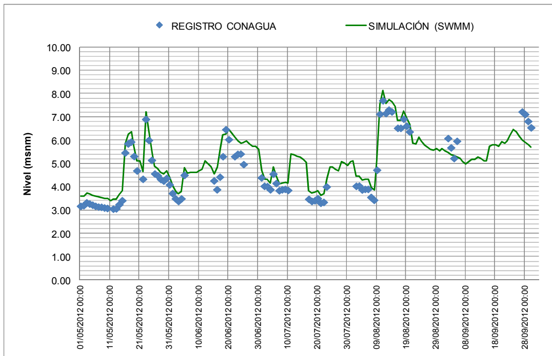
Figura 5.16 Hidrograma medido vs calculado (SWMM) -Estación Hidrométrica PUEBLO NUEVO
