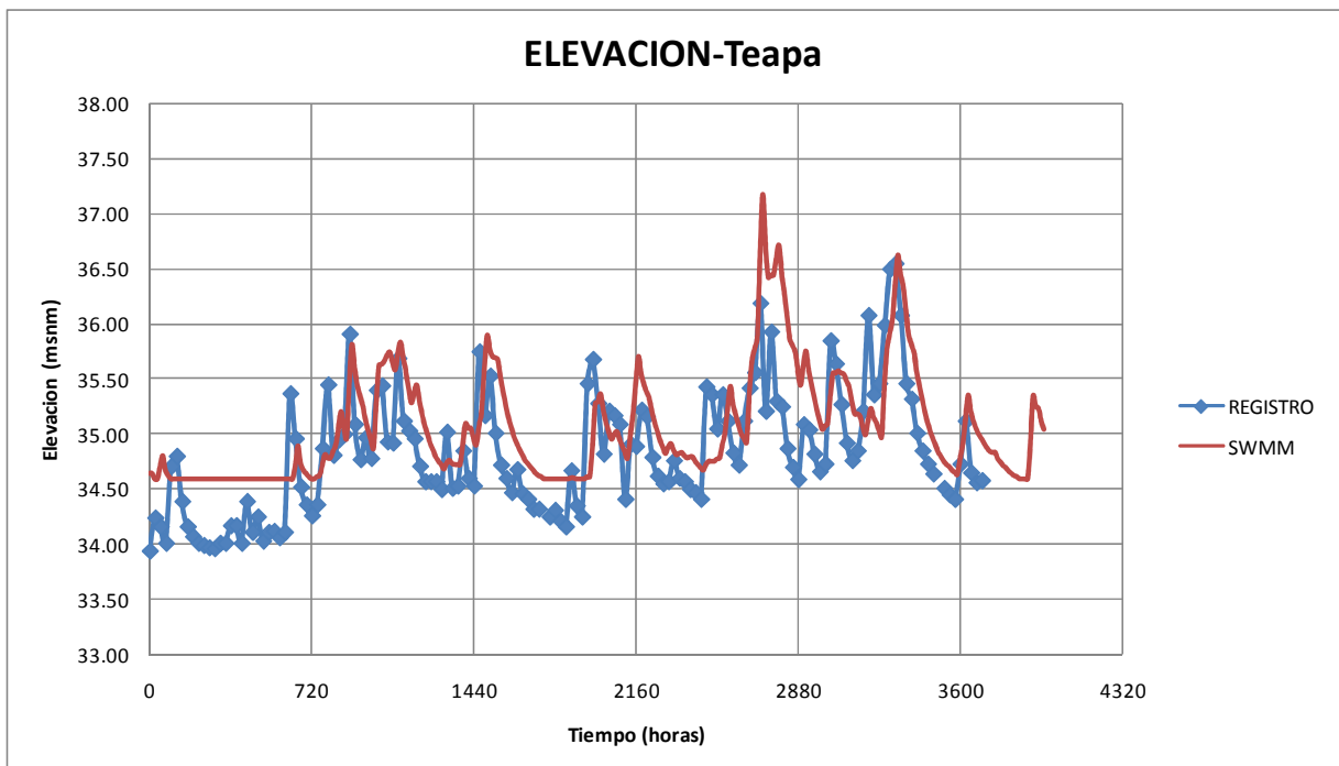
Figura 4.11 Limnigramas medido y calculado en la estación hidrométrica Teapa
