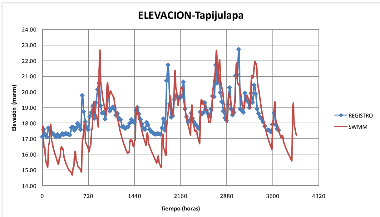
Figura 4.7 Limnigramas medido y calculado en la estación hidrométrica Tapijulapa
