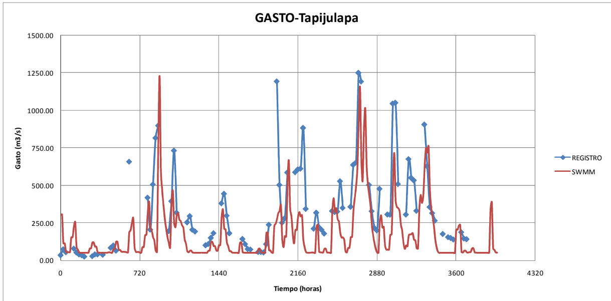
Figura 4.14 Resultados de la calibración del año 2011 Variable: Gasto Punto de control: EH Tapijulapa
