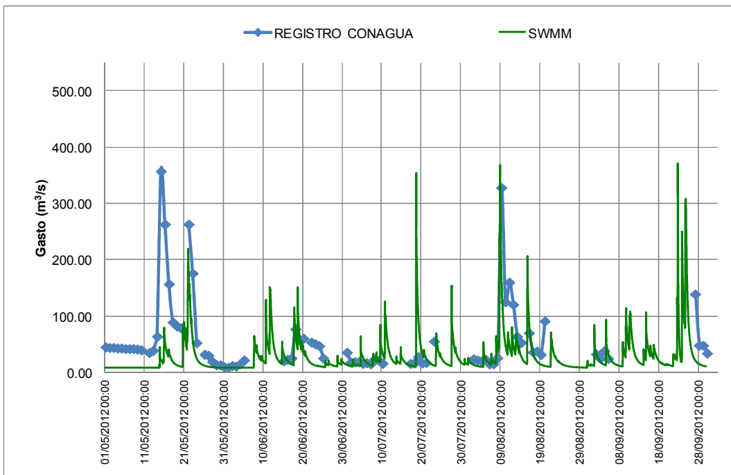
Figura 5.14 Hidrograma medido vs calculado (SWMM) -Estación Hidrométrica PICHUCALCO
