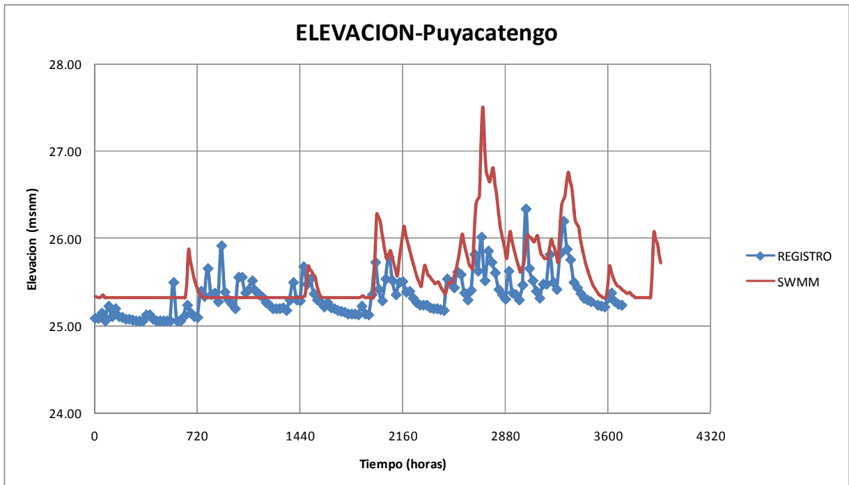
Figura 4.9 Limnigramas medido y calculado en la estación hidrométrica Puyacatengo
