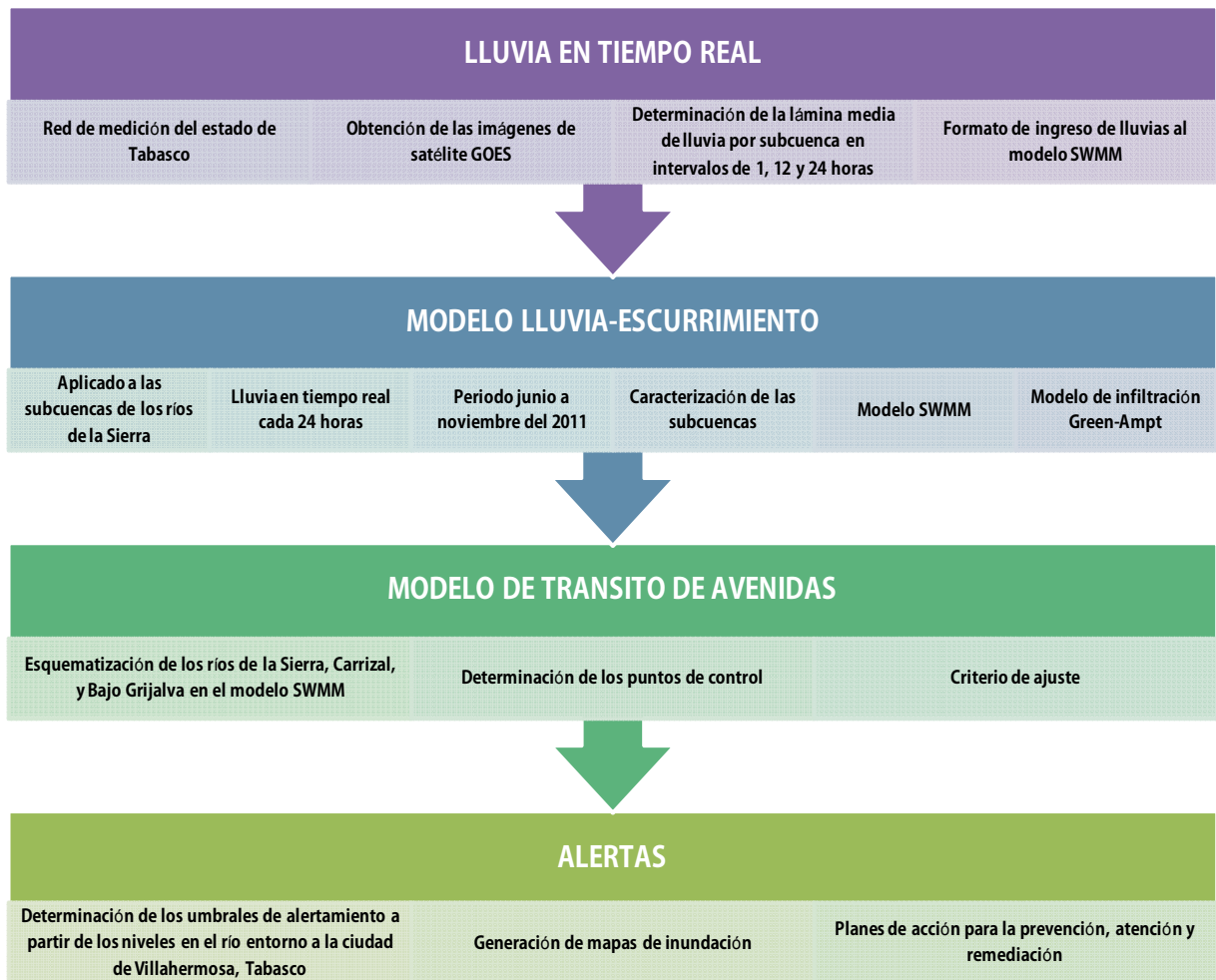
Figura 3.10 Diseño conceptual propuesto del SAT para la ciudad de Villahermosa
