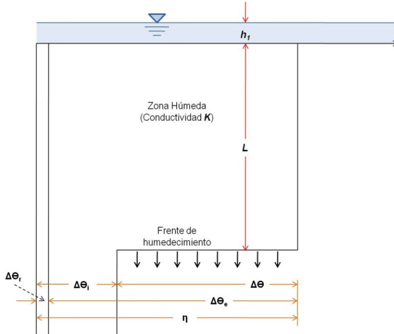
Figura 4.2 Modelo de infiltración de Green - Ampt
