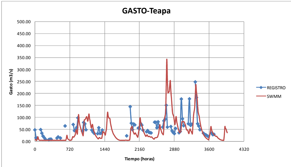
Figura 10. Hidrogramas medido y calculado en la estación hidrométrica Teapa
