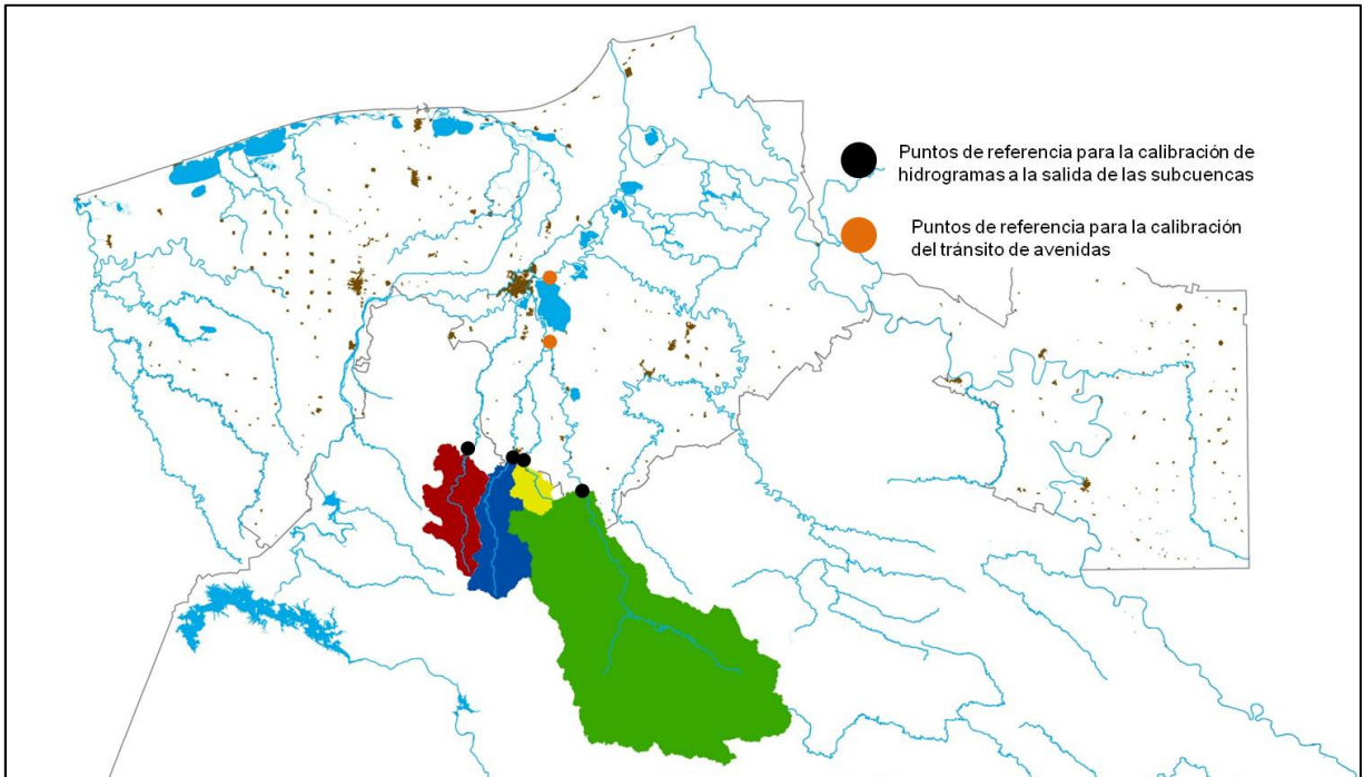
Figura 4.5 Puntos de medición de hidrogramas a la salida de las subcuencas
