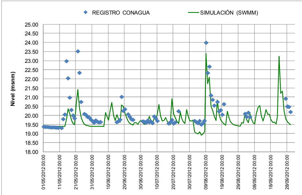
Figura 5.13 Limnigrama medido vs calculado (SWMM) -Estación Hidrométrica PICHUCALCO
