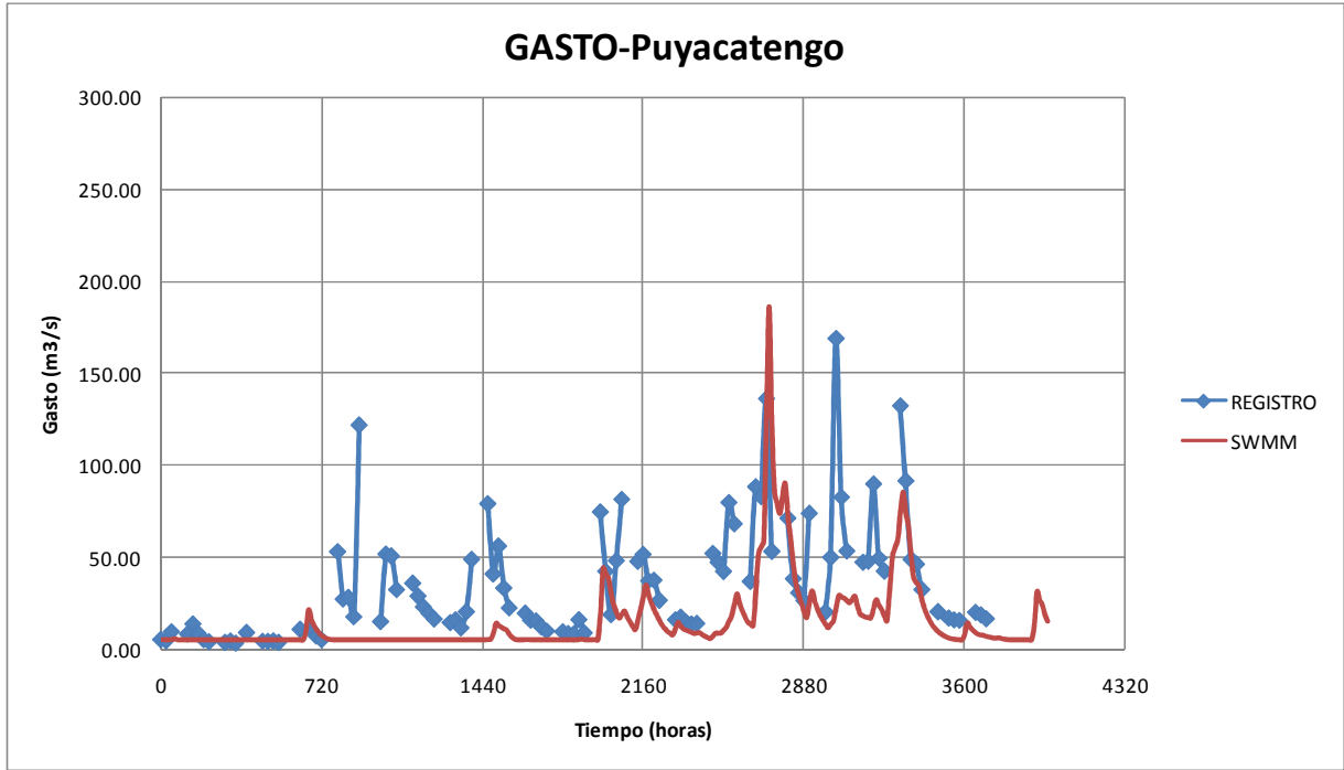
Figura 4.8 Hidrogramas medido y calculado en la estación hidrométrica Puyacatengo
