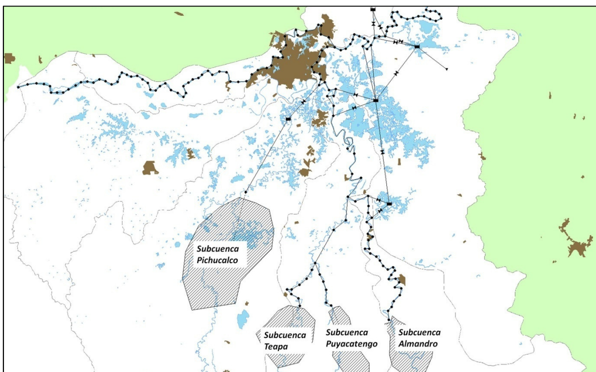
Figura 3.16 Ubicación de las subcuencas dentro del esquema
