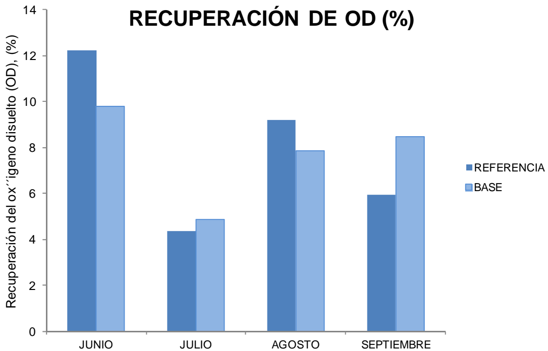
Figura 4.8. Recuperación de OD durante la época de lluvias para los escenarios de referencia y base para el 2020.
