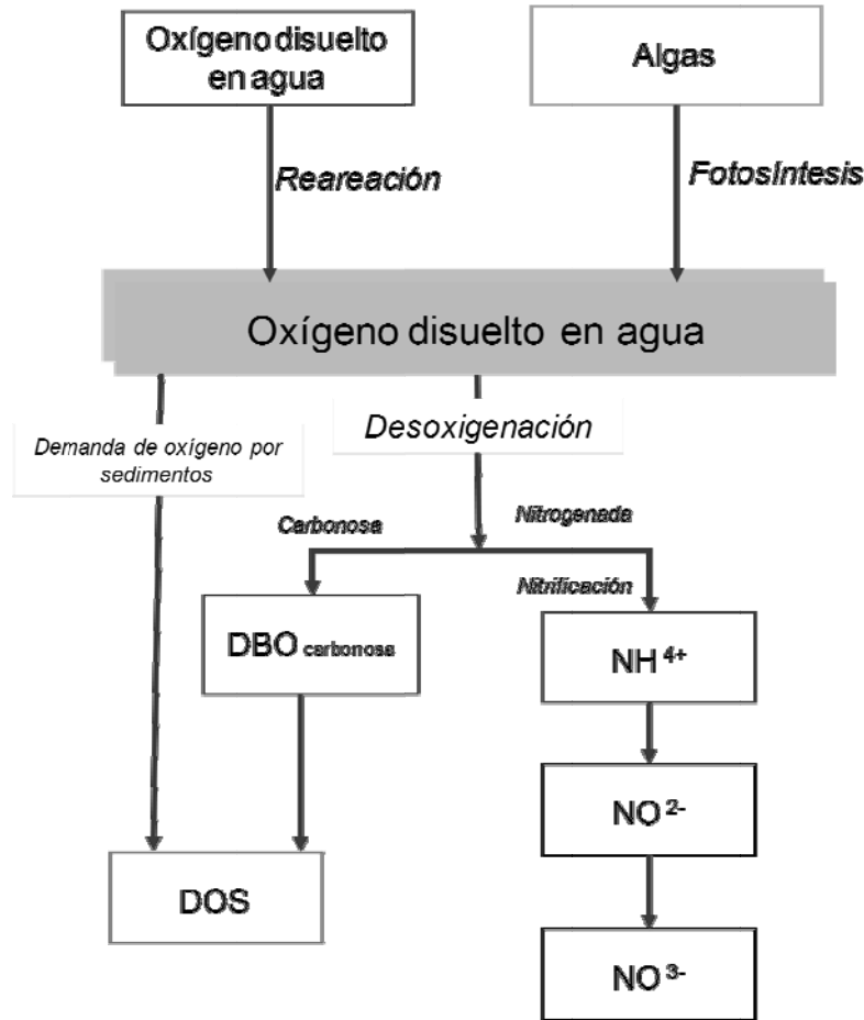
Figura 2.2. Representación conceptual del flujo de oxígeno en un volumen de control.
