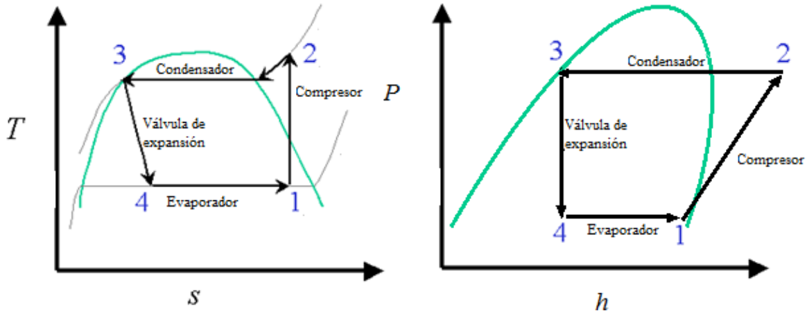
Figura 3-4 Diagrama T-s y P-h de bomba de calor simple
