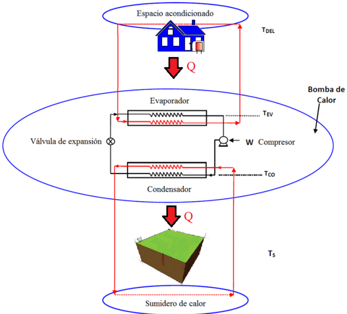
Figura 2-3 Configuración de Bomba de Calor para enfriamiento
