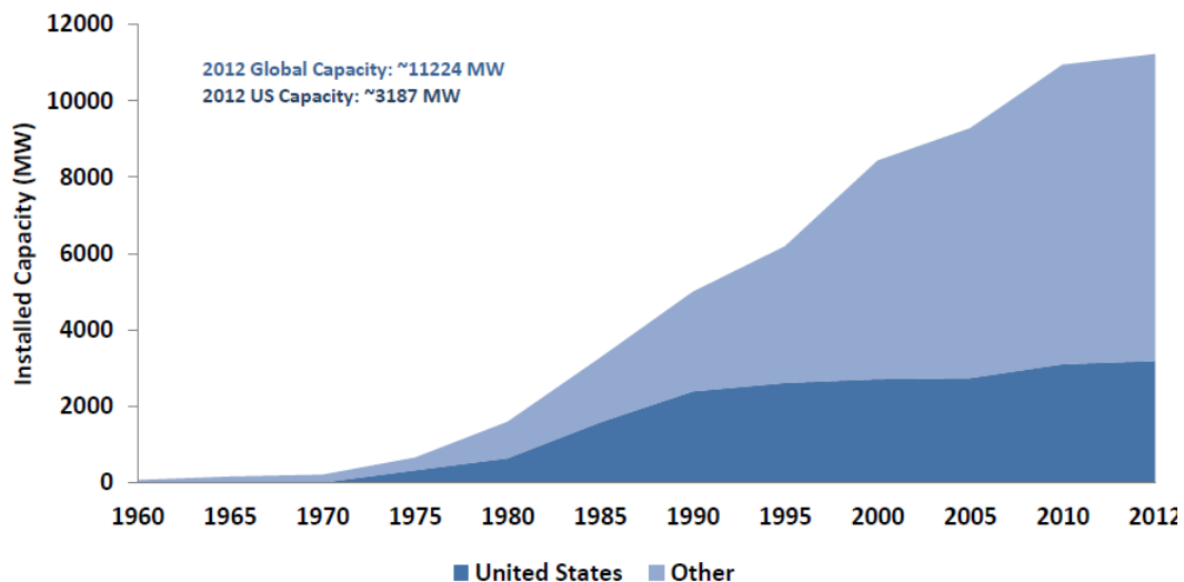
Figura 0-4 Capacidad Instalada Mundial de los años 1960 a 2012 11
