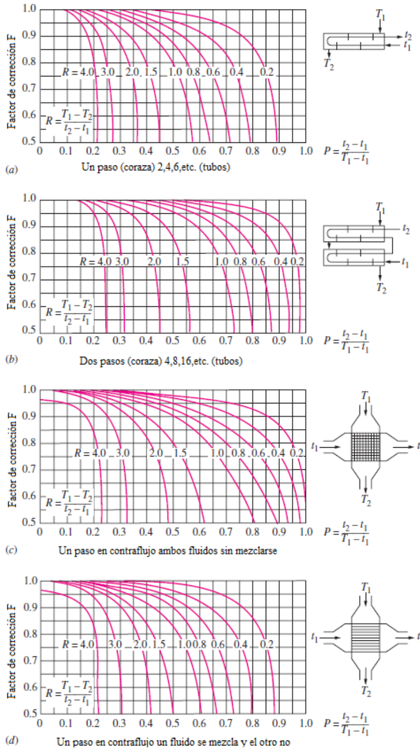
Anexo 8-3 Factores de corrección de diferencia de temperaturas media logarítmica para distintas configuraciones 74
