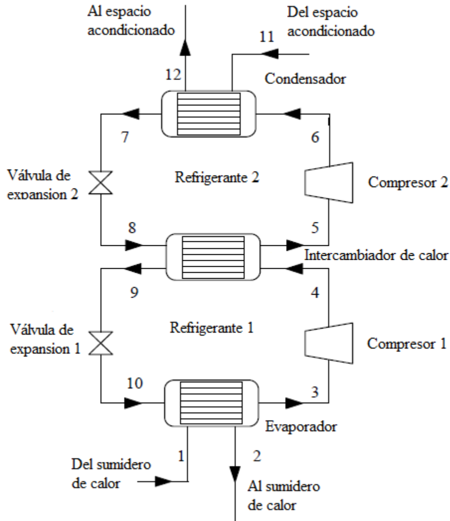
Figura 3-10 Esquema de bomba de calor de dos etapas con intercambiador de calor 41
