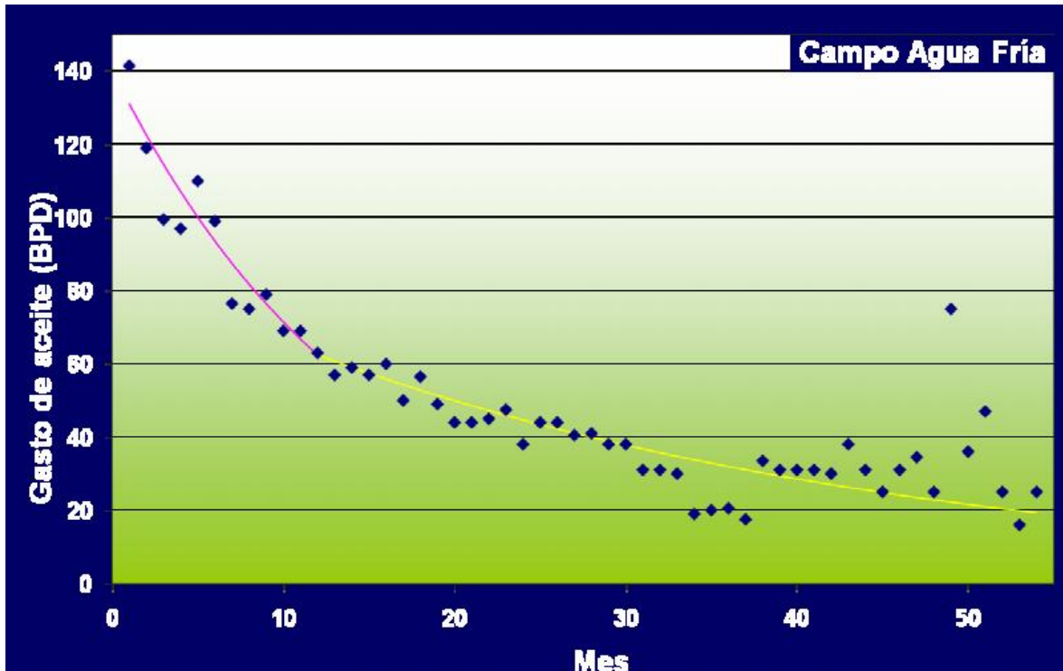
Figura 6.1. Grafica de producción típica de un pozo en el campo Agua Fría (Tomada de Camacho, 2009)
