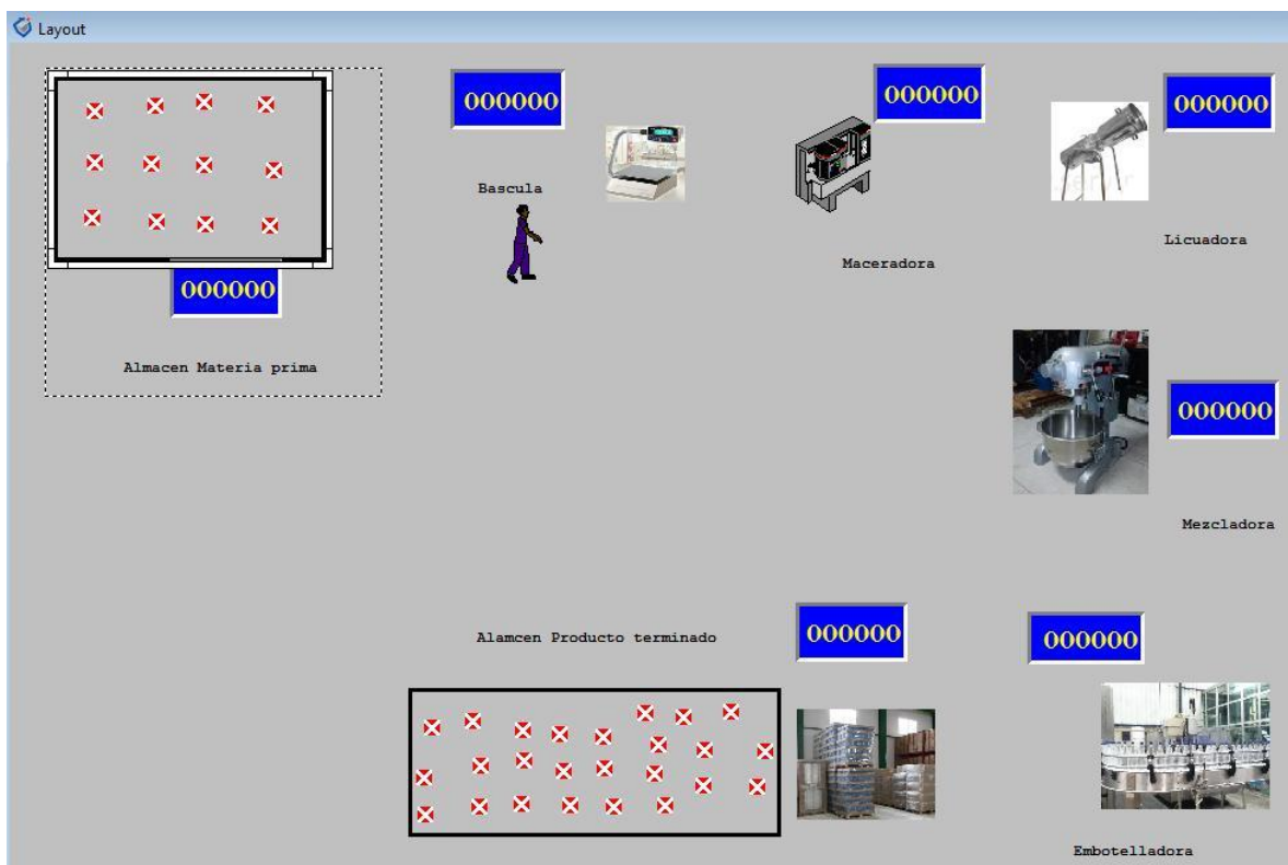
Figura 14. Distribución de locaciones para la simulación del proceso.
