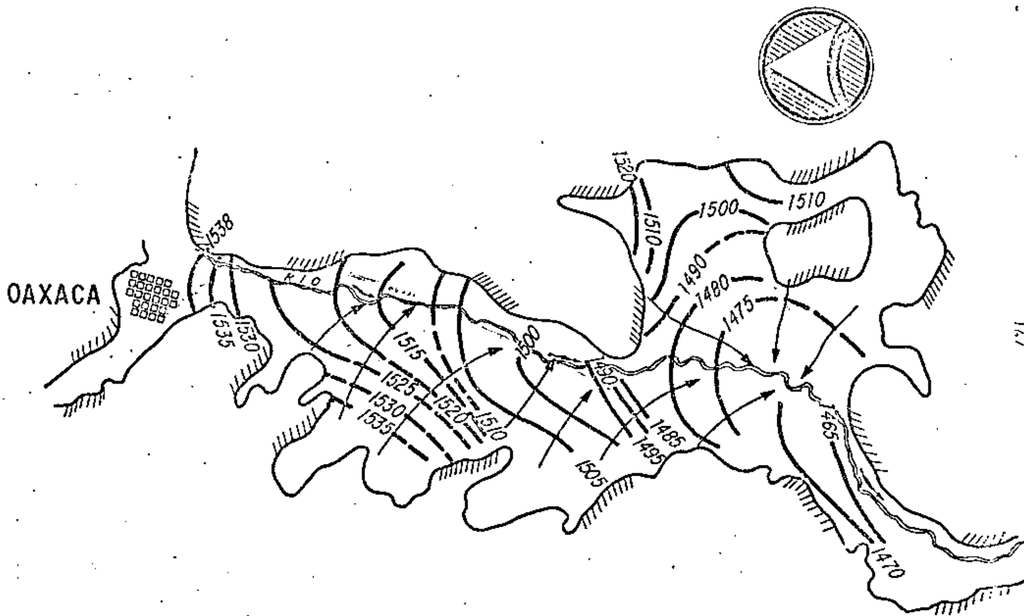
CONFIGURACION DE ELEVACION NIVEL ESTÁTICO MOSTRANDO LA INFLUENCIA QUE TIENEN LOS LIMITES GEOLOGICOS Y LOS ESCURRIMIENTOS SUPERFICIALES
