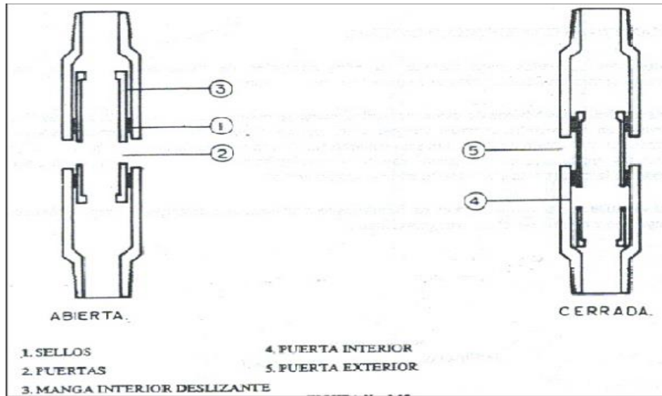
Figura 1.2 Camisa Deslizable
