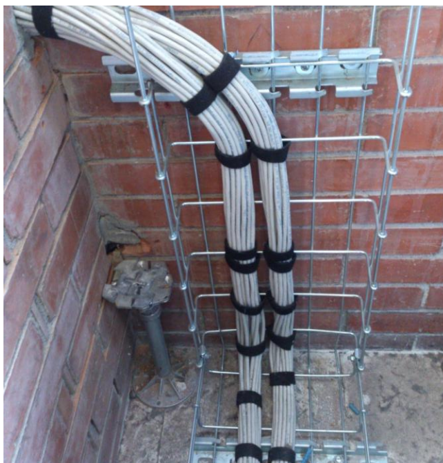
Figura 6.4.4 Instalación de escalerilla en Site de CTI
