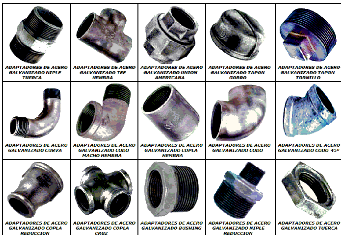
Figura 3.4.3 Adaptadores de tubo conduit metálico rígido de pared gruesa
