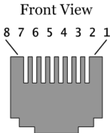
Figura 3.2.2 Vista frontal del conector RJ-45
