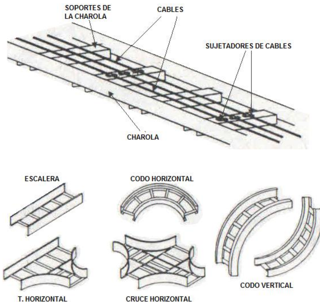
Figura 3.4.7 Charolas y algunos accesorios
