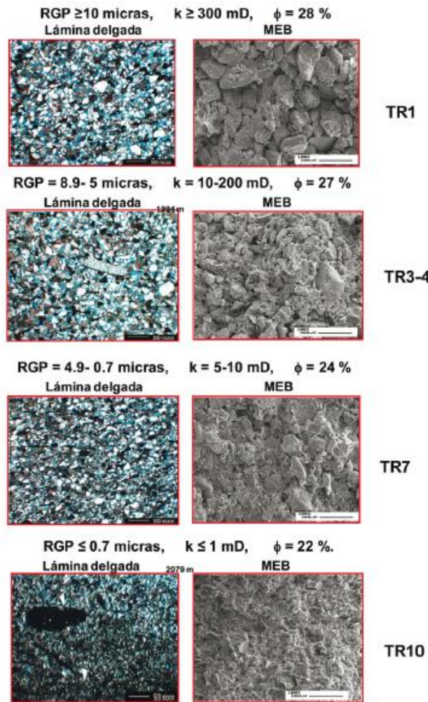
Figura 4.10 Fotomicrografías (nicoles cruzados) de los diferentes tipos de rocas petrofísicas presentes en el campo, además de una imagen de microscopio electrónico de barrido. Tomada de: Antonio Quinlantan P. 2012
