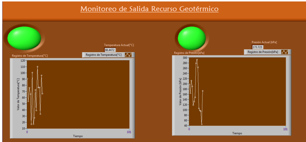
Figura 3.25 Gráficas de Temperatura y Presión de Salida Recurso Geotérmico
