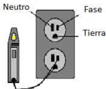
Figura 42. Identificación de la polaridad de tomacorriente
