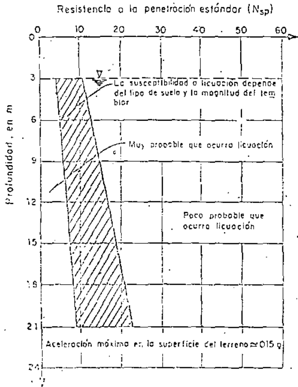
Fig 20 Gráficas para evaluar la susceptibilidad a licuación de arenos con el nivel freático a una profundidad aproximada de 3.0m
