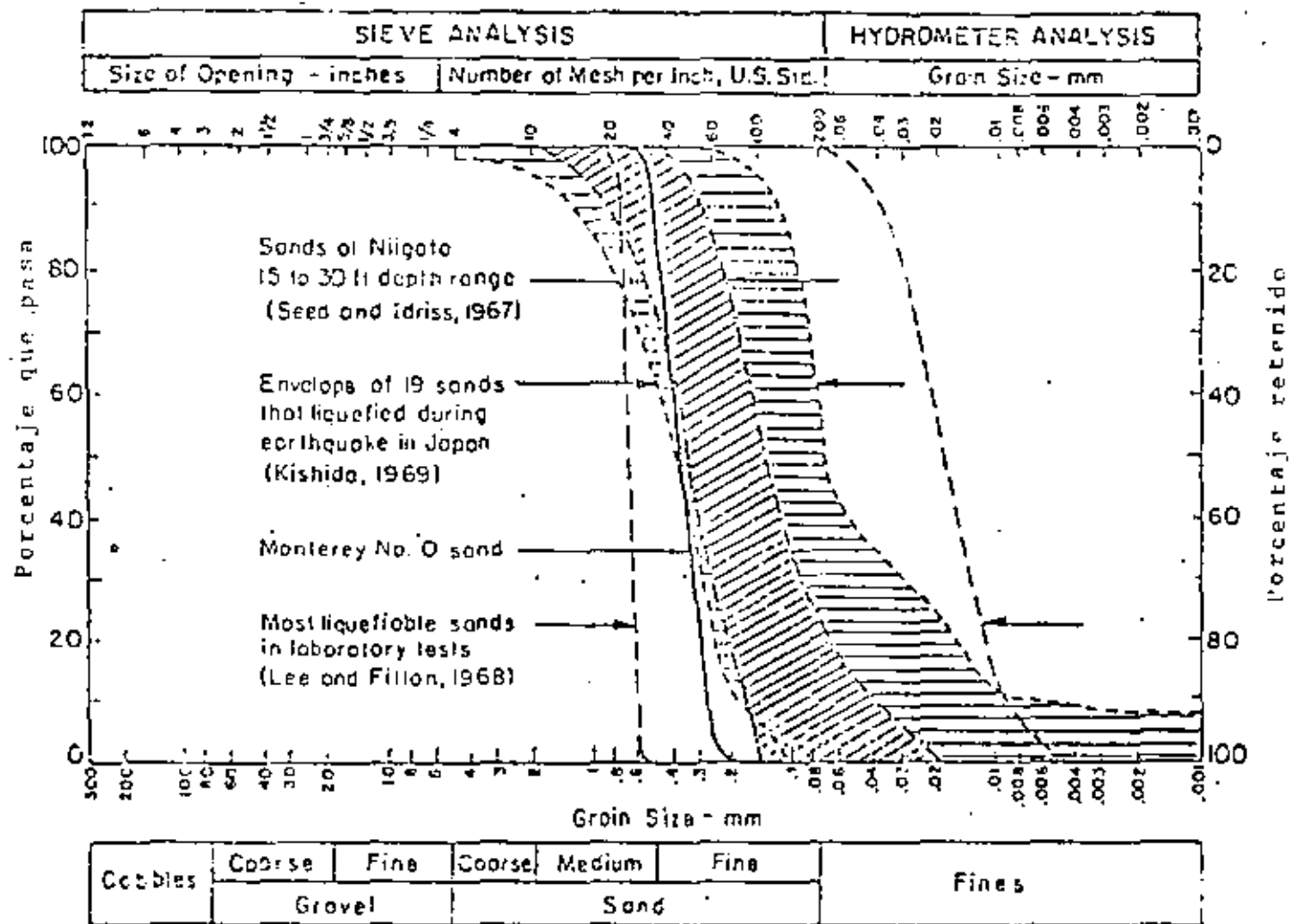
Fig 9 Suelos susceptibles a licuación.
