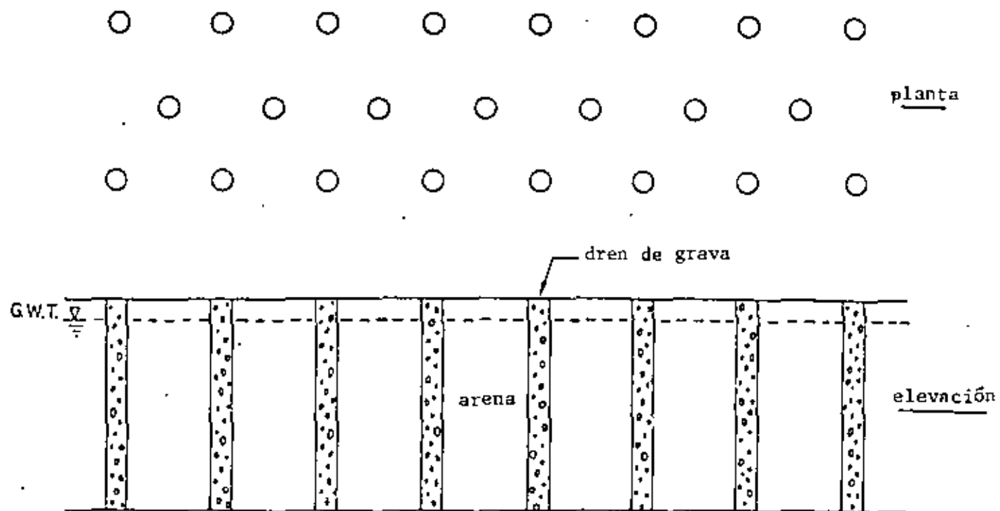
Fig 22(a). Sistema de drenes de grava
