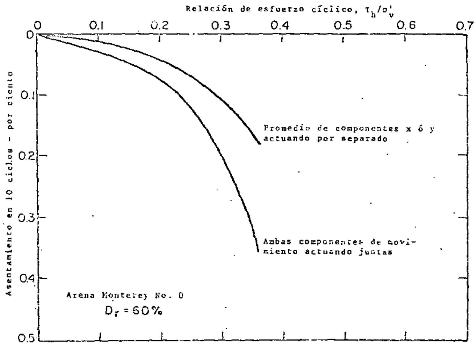
Fig 8 Asentamiento de arena seca bajo movimiento unidireccional y multidireccional, (Fyke et al, 1974).
