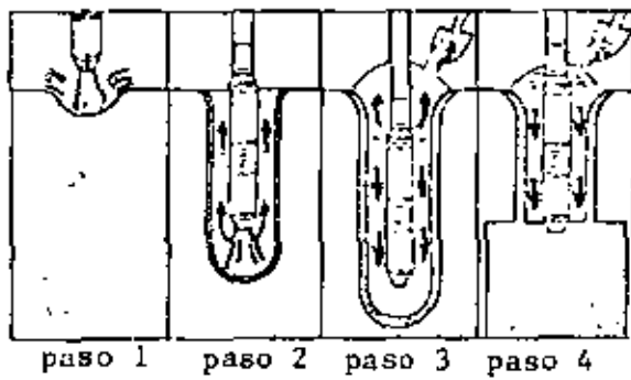
Fig 21(b) Proceso de compactación mediante vibroflotación
