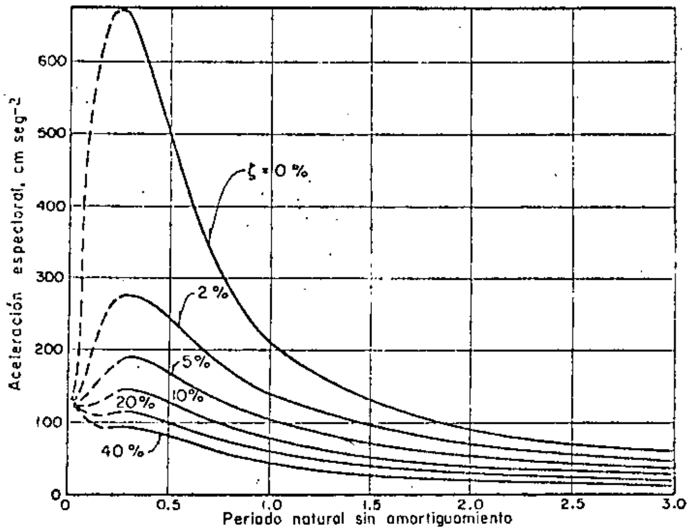
Fig. 16 Espectros de la aceleración media normalizada para los temblores de California (Según G.W. Housner)
