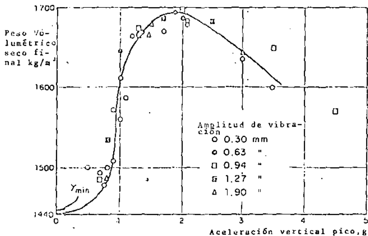
Fig 4 Efecto de la intensidad de aceleración sobre la densificación de la arena en pruebas de mesa vibratoria vertical
