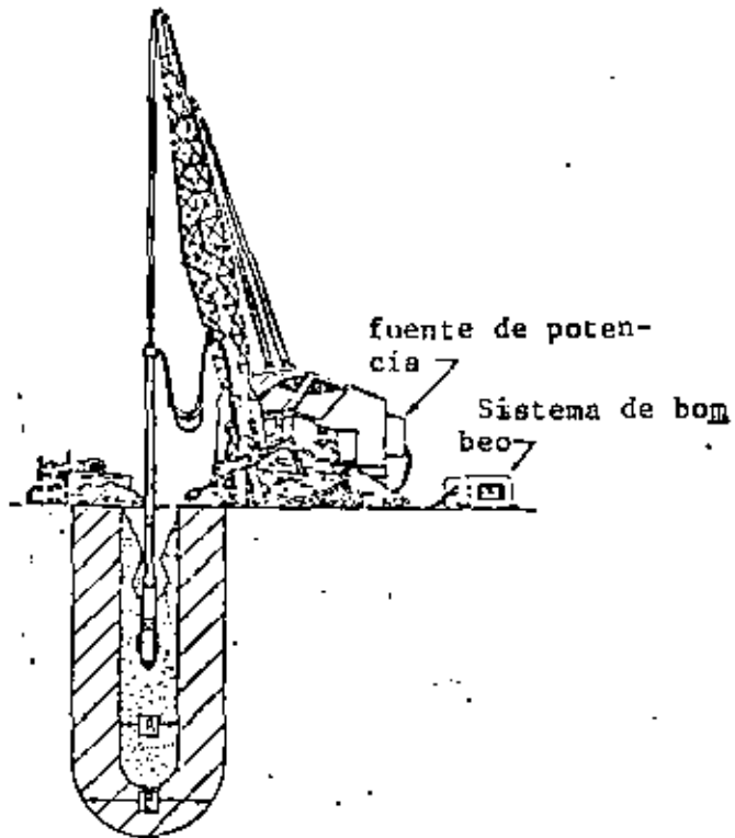
Fig 21(a) Equipo de vibroflotación
