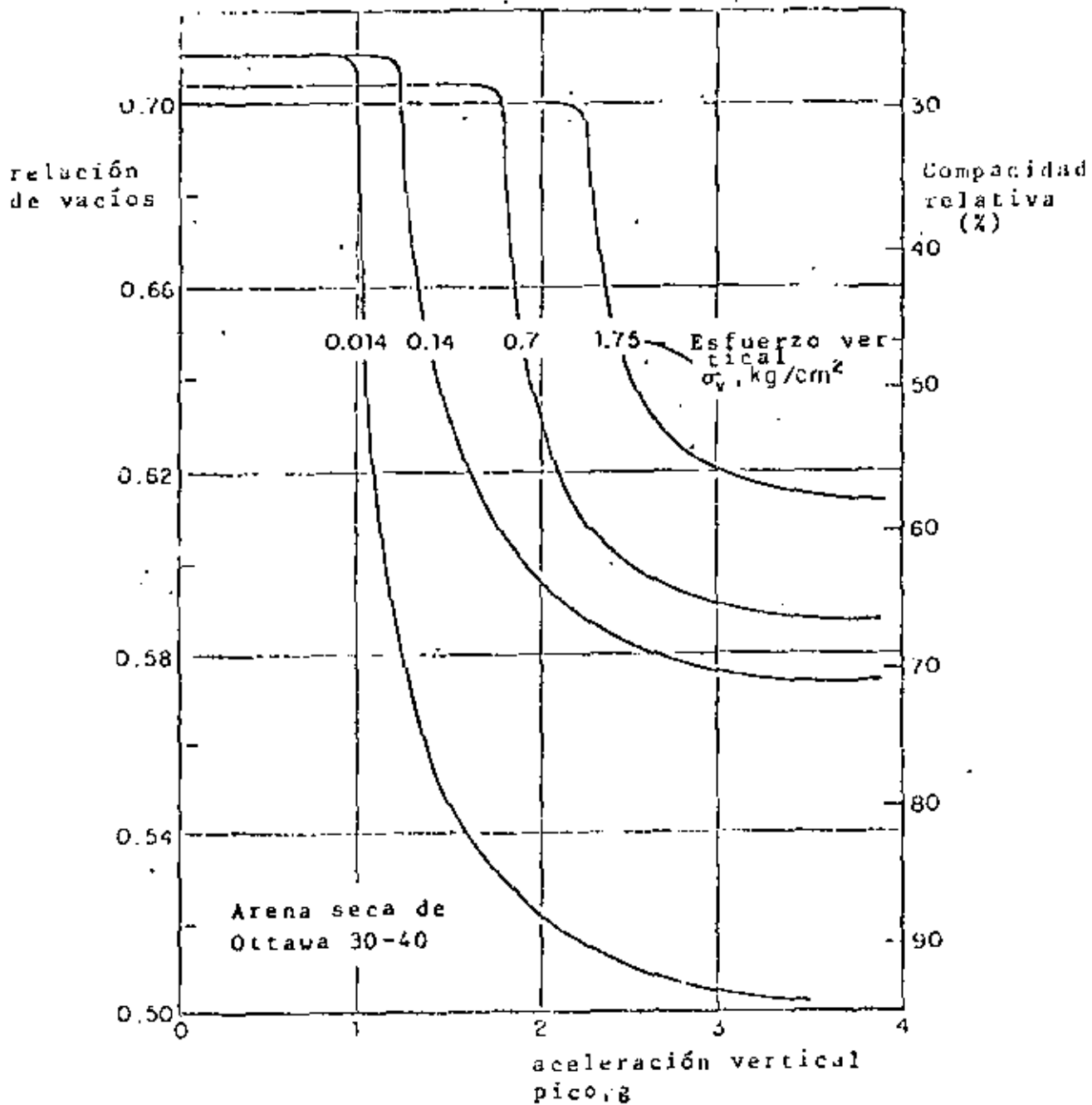
Fig 5 Efectos de la intensidad de aceleración y esfuerzo de confinamiento sobre la densificación de arena seca de Ottawa en pruebas de mesa vibratoria vertical.
