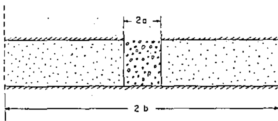
Fig 22(b) Dren de grava con drenaje radial únicamente
