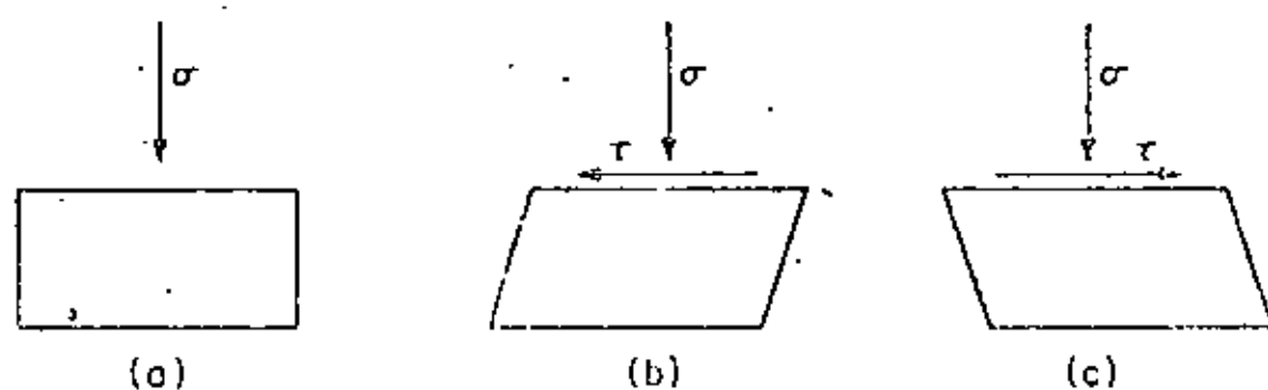
Fig 12. Condición idealizada de esfuerzos para un elemento de suelo en el interior de un depósito, durante un temblor
