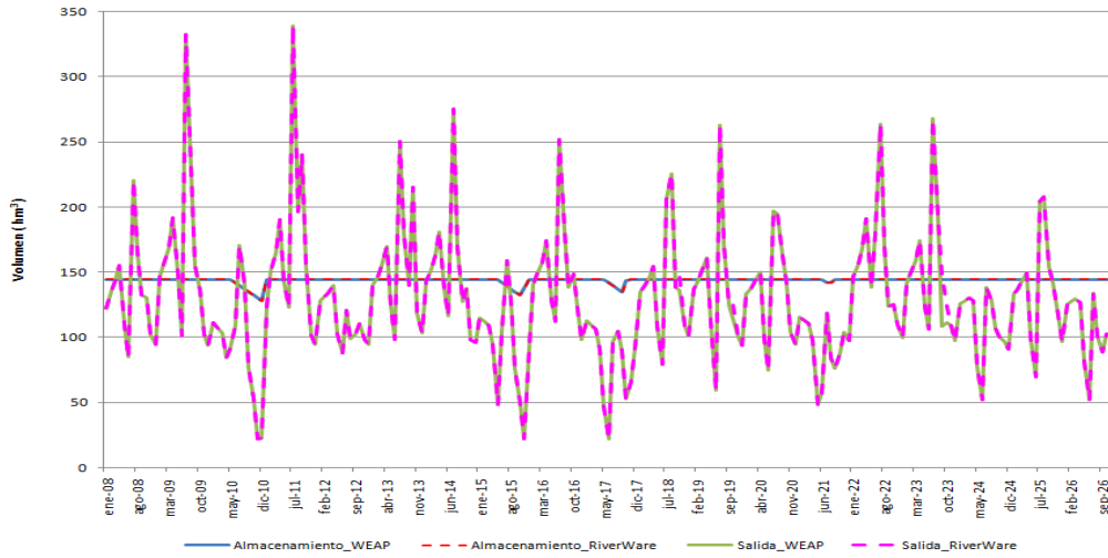
Figura 4.18 Almacenamiento y Salida de Morrow Point (2008-2026)
