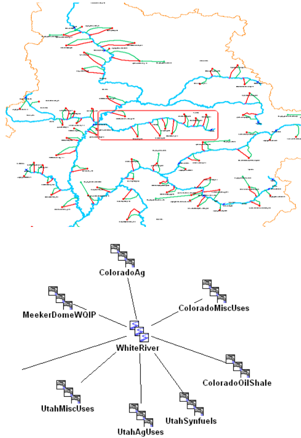
Figura 4.3 Esquema de tramo de río White del modelo WEAP y RiverWare
