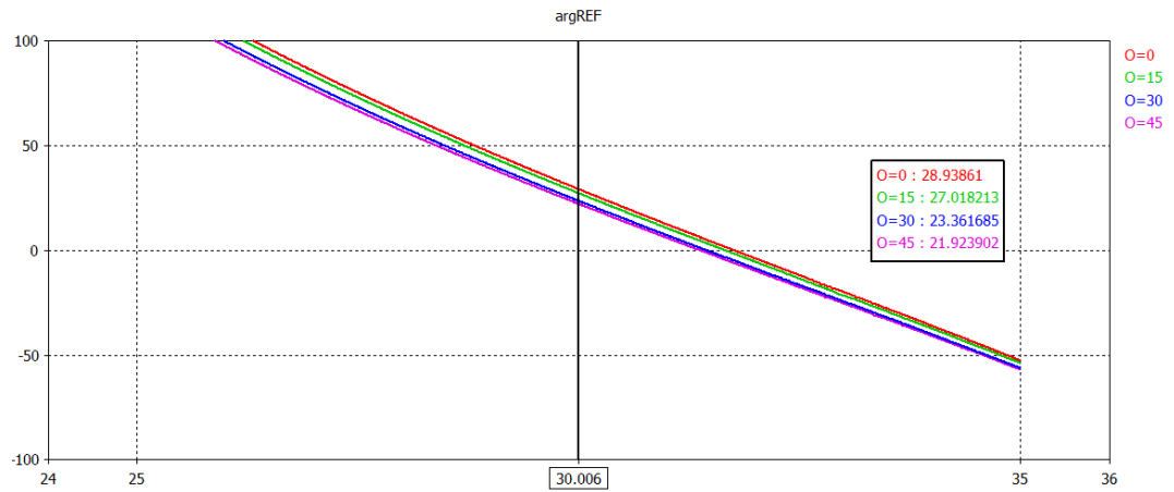
Figura 2.36 Fase del coeficiente de reflexión (intervalos de 15°, Onda Controlada, con pared PEC)
