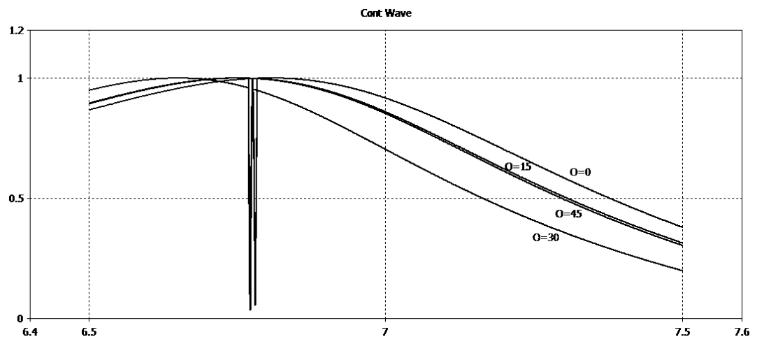
Figura 2.46: Magnitud de la Onda Controlada (intervalos de 15^\circ , con pared PEC)
