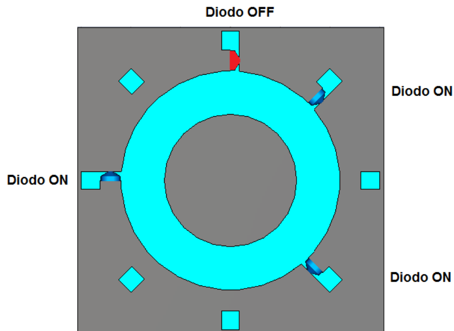
Figura 3.5: Elemento rediseñado con menor cantidad de PIN.
