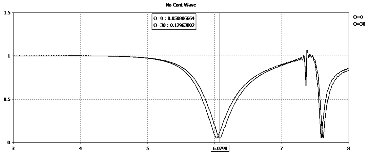
Figura 2.53: Magnitud de la Onda No Controlada (0° y 30°, con pared PEC)
