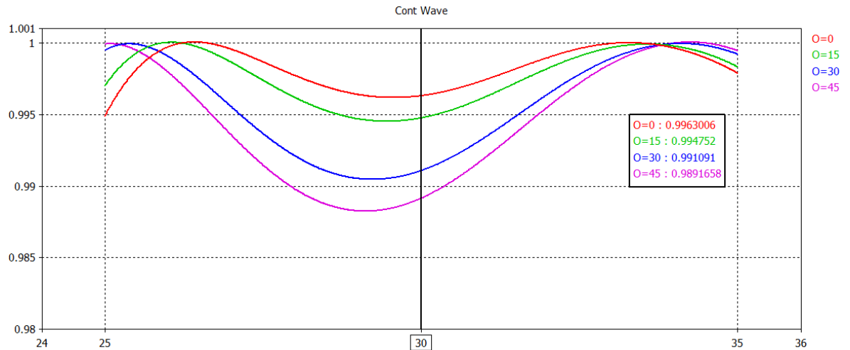
Figura 2.34 Magnitud de la Onda Controlada (intervalos de 15°, con pared PEC)
