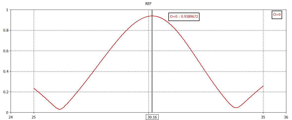
Figura 3.7: Respuesta en frecuencia ante una onda con polarización horizontal (Ortogonal). 0^\circ y 45^\circ
