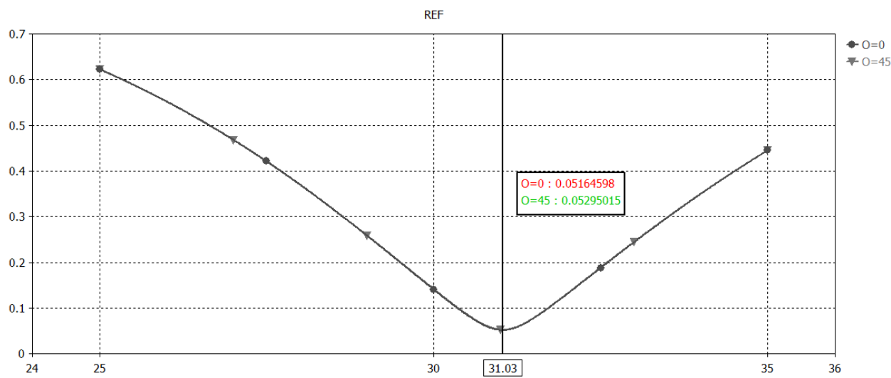
Figura 3.6: Respuesta en frecuencia ante una onda con polarización vertical (Paralela). 0° y 45°
