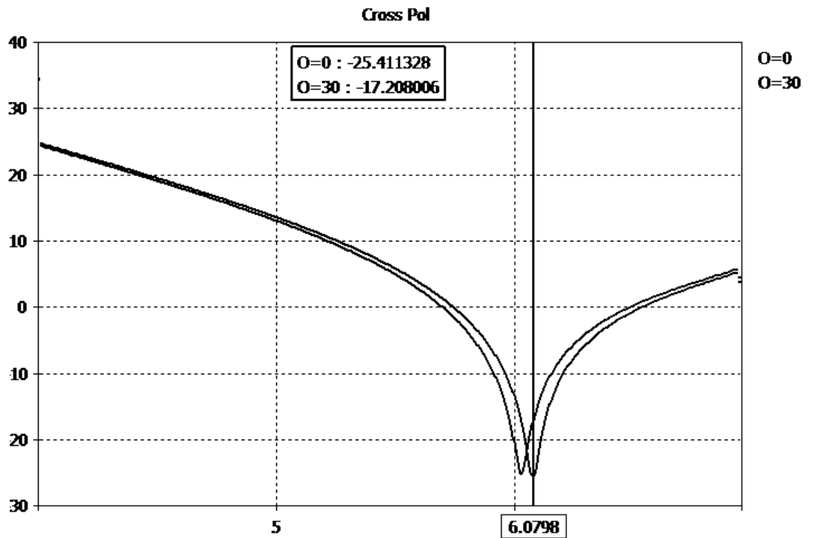
Figura 2.54: Polarización cruzada (0° y 30°)
