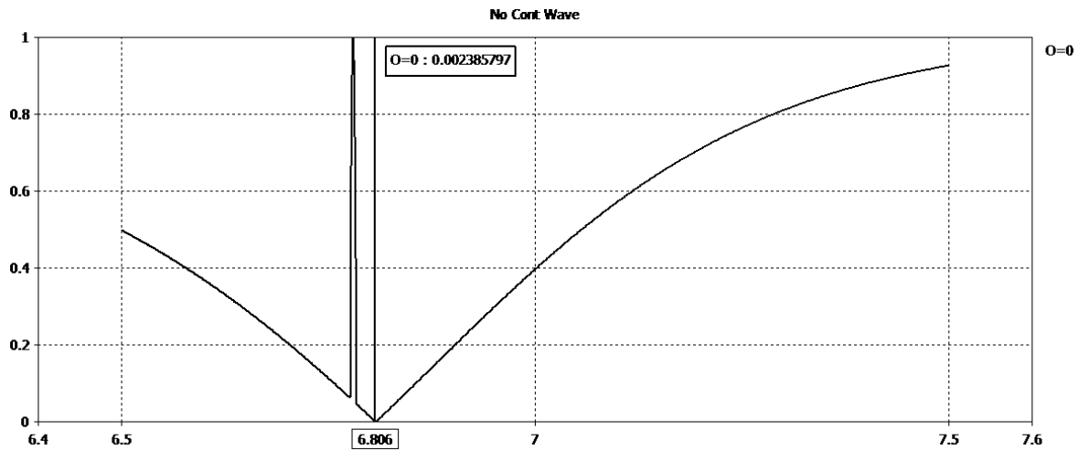
Figura 2.44: Magnitud de la Onda No Controlada (0°, con pared PEC)
