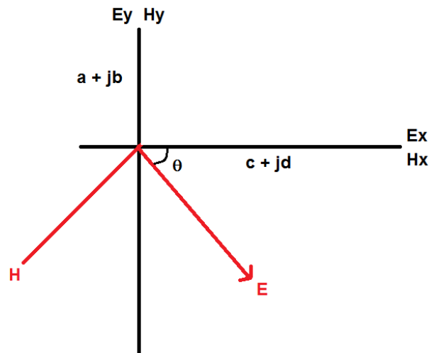
Figura 2.10: Diagrama del campo EM de la onda perpendicular respecto a las sondas . E_x y E_y indican la dirección en que se orientan las sondas que miden el campo eléctrico, mientras que H_y y E_x indican la dirección de las sondas que miden el campo magnético. E y Y representan la dirección de los campos eléctrico y magnético en la onda incidente.
