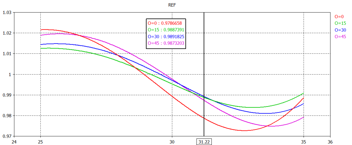
Figura 2.22: Coeficiente de reflexión, Onda controlada. (Intervalos de 15°, con pared PEC)
