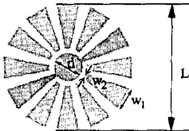
Figura 2.50: Dimensiones del elemento de Legay [8].
