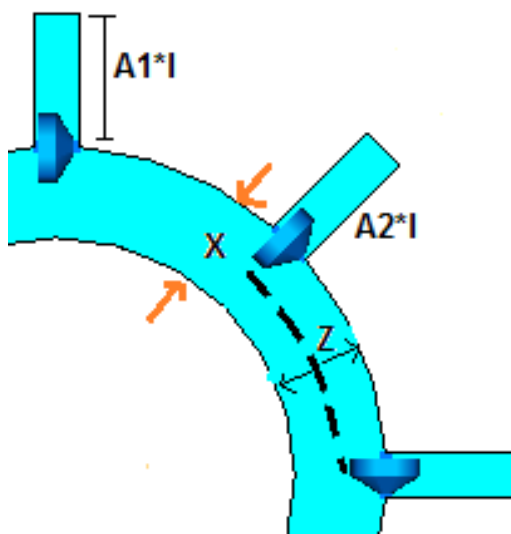
Figura 3.19: Constantes en la geometría del elemento.
