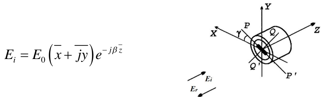
Figura 2.1. Elemento espirafase con onda RHCP incidente.
