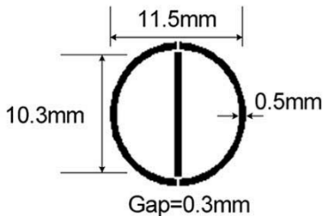
Figura 2.39: Geometría del Elemento espirafase basado en anillo y dipolo [7].
