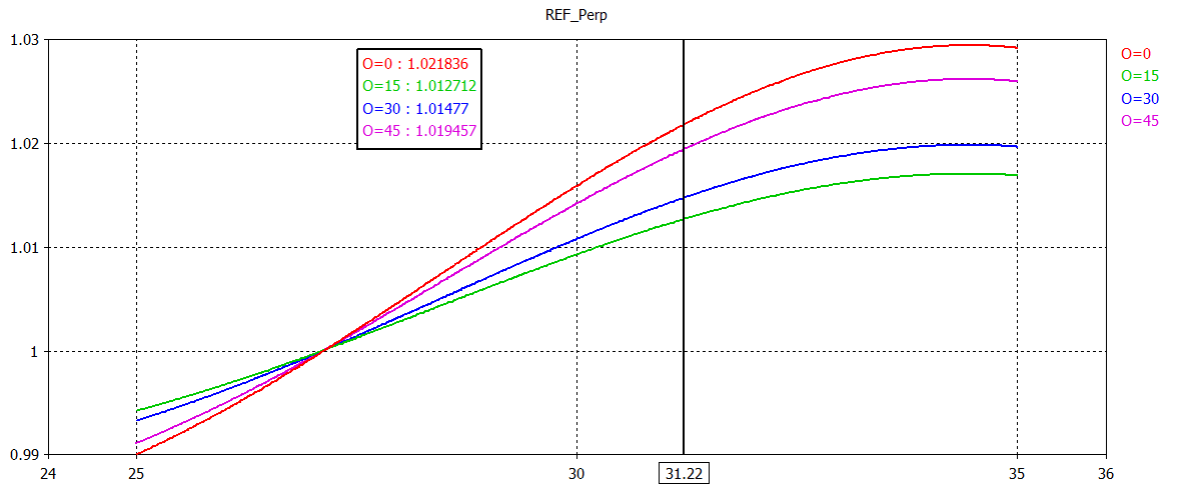
Figura 2.23: Coeficiente de reflexión, Onda No controlada. (Intervalos de 15°, con pared PEC)
