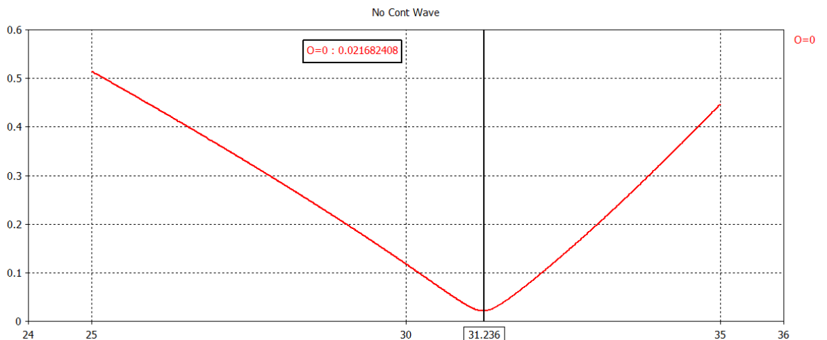
Figura 2.17 Respuesta en frecuencia del dipolo (0°, con pared PEC, Onda perpendicular al dipolo)
