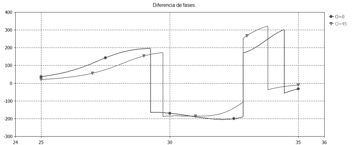
Figura 3.22: Diferencia de fases. 0° y 45°
