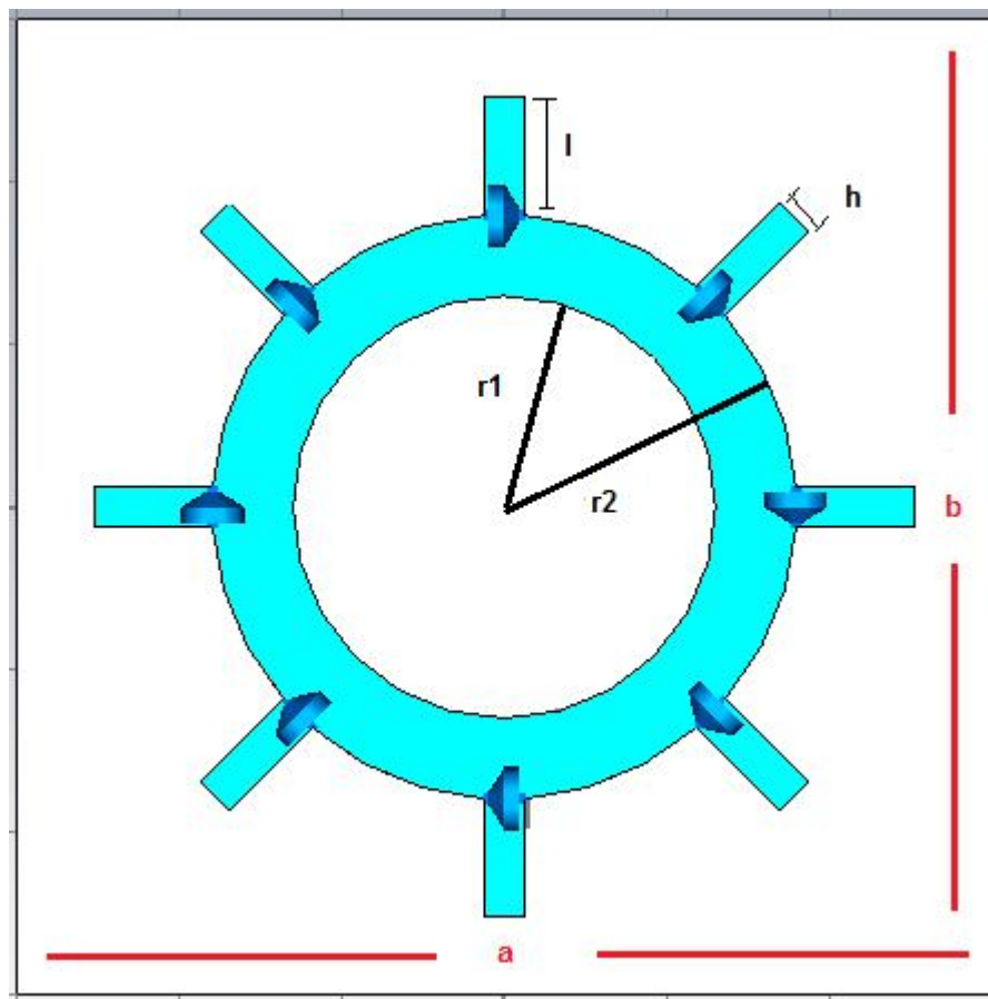
Figura 3.1 (b): Medidas del elemento propuesto en [2] (frente)
