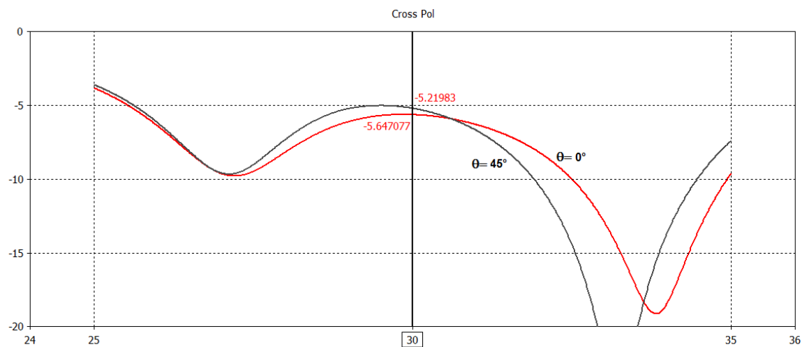
Figura 3.4: Polarización Cruzada en dB ( 0^\circ y 45^\circ )
