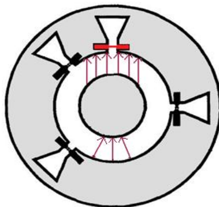
Figura 2.5: Elemento espirafase basado en ranuras girado electrónicamente [5].
