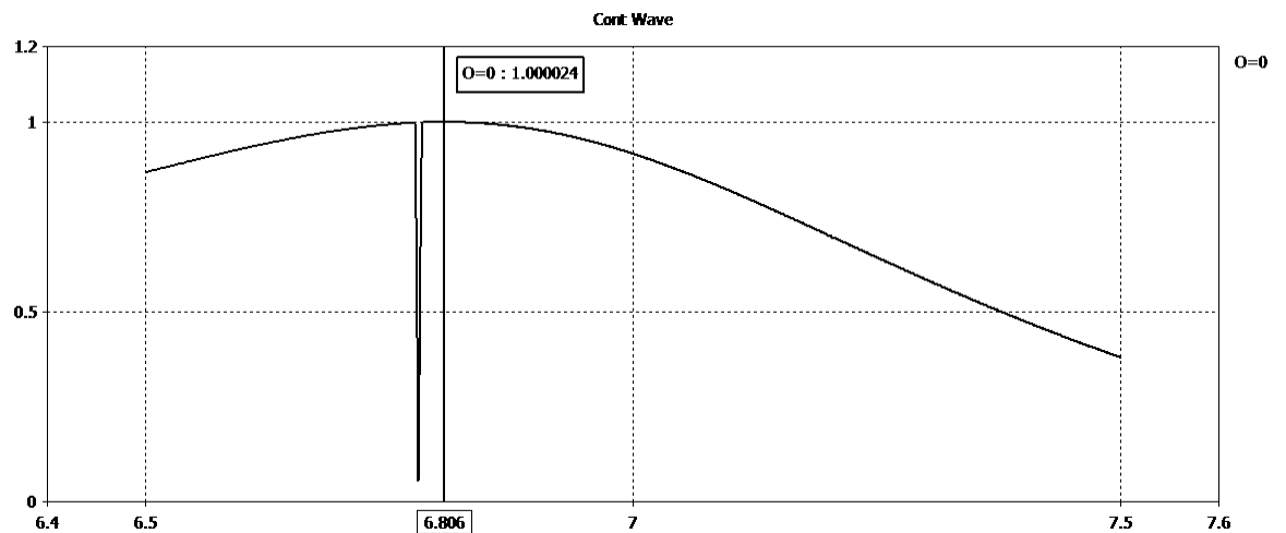
Figura 2.43: Magnitud de la Onda Controlada ( 0^\circ , con pared PEC)
