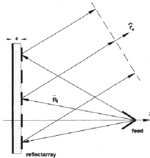
Figura 1.6: Geometría de la antena reflectora.
