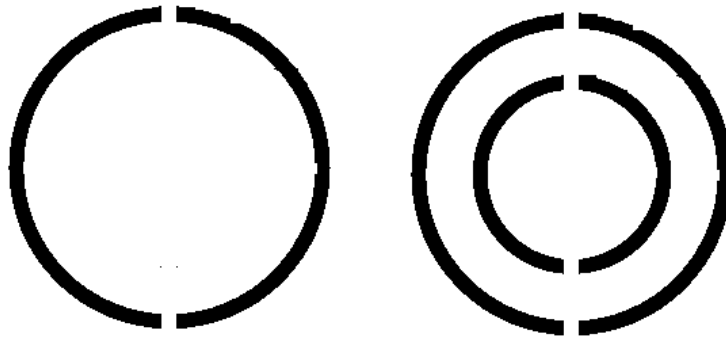
Figura 2.55: Elementos de anillo ranurado [9] y doble anillo ranurado [10]
