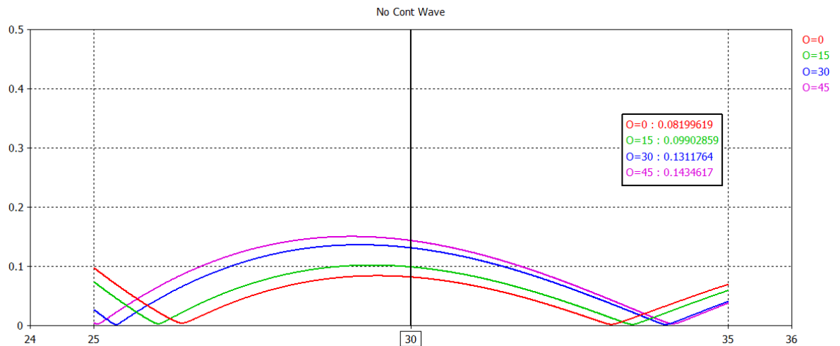
Figura 2.35 Magnitud de la Onda No Controlada (intervalos de 15°, con pared PEC)
