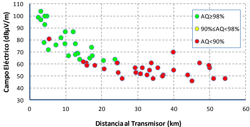
Figura 5.4. Resultados de recepción del modo Day 16 en función de la distancia al transmisor.
