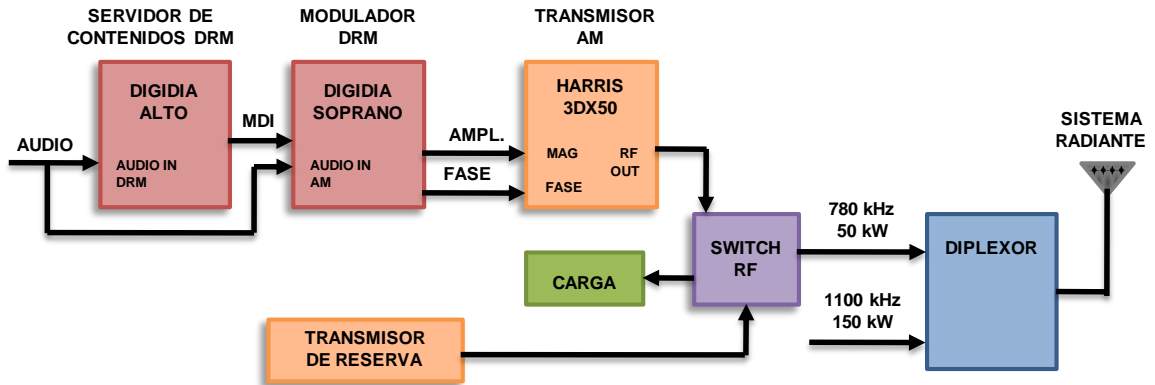
Figura 3.6. Esquema del transmisor en CBN.
