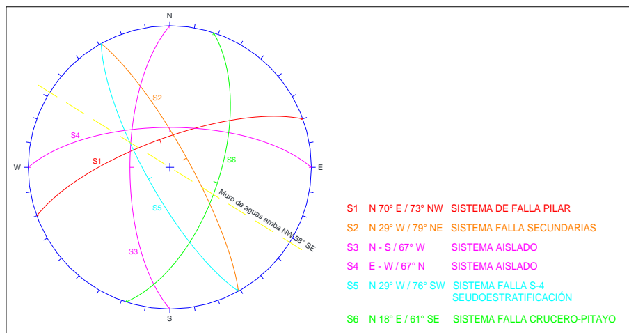
Figura 2.71.- Representación estereográfica de los sistemas de discontinuidades de la pared de aguas arriba de la casa de máquinas.
