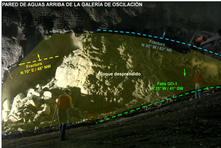
Figura 2.107.- Bloque desprendido en la pared de aguas arriba de la GO.
