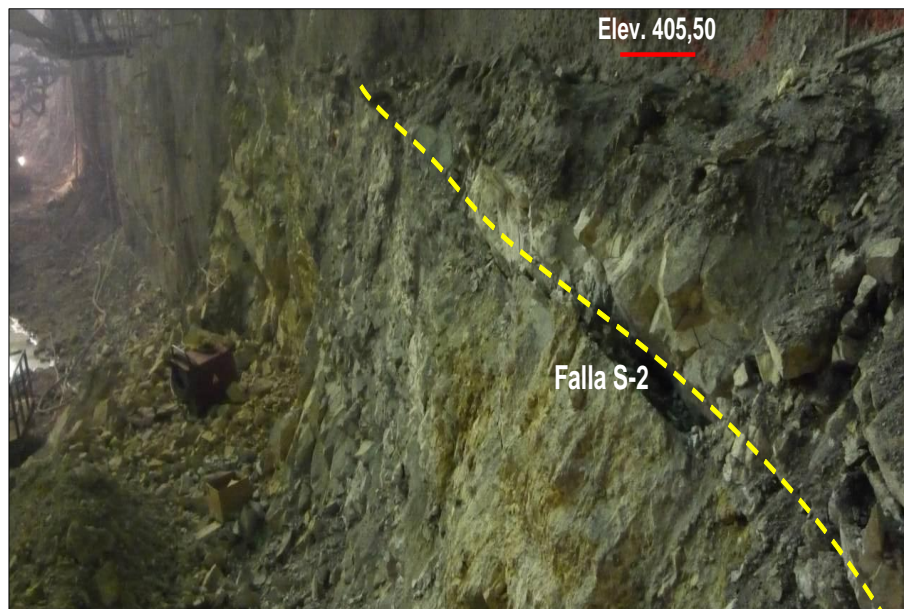
Figura 2.68.- Falla S-2.
