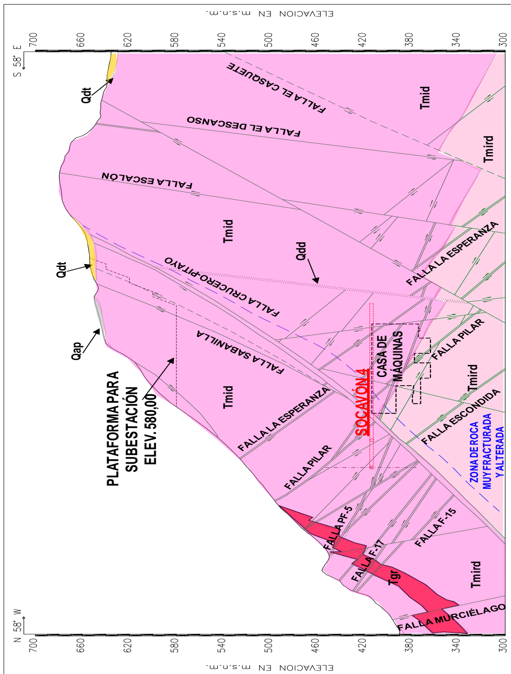
Figura 2.62.- Sección por el eje mayor de casa de máquinas.
