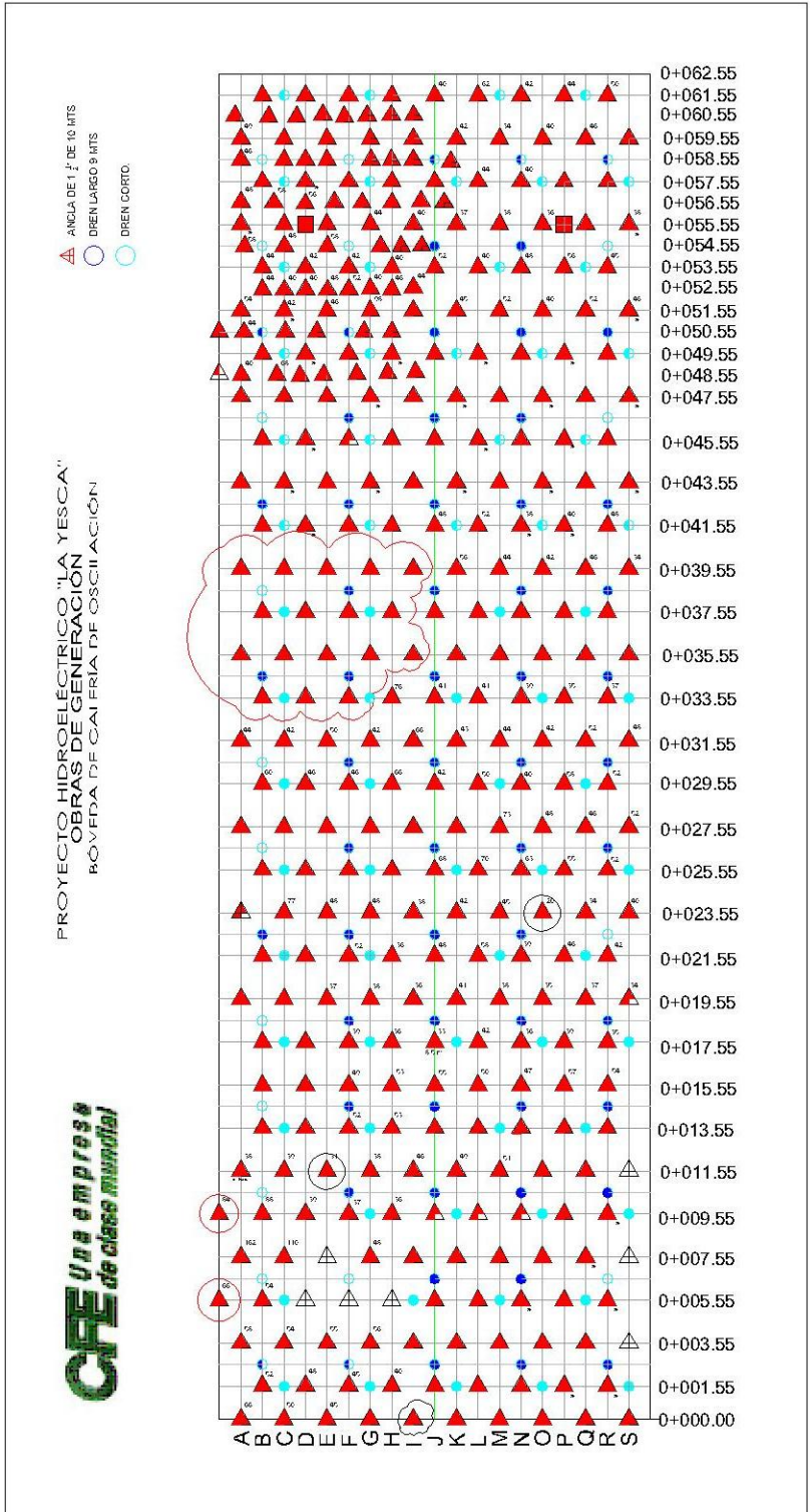
Figura 2.115.- Anclaje final en bóveda de galería de oscilación
