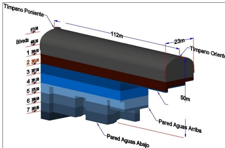
Figura 2.36.- Segundo banqueo de la casa de máquinas.
