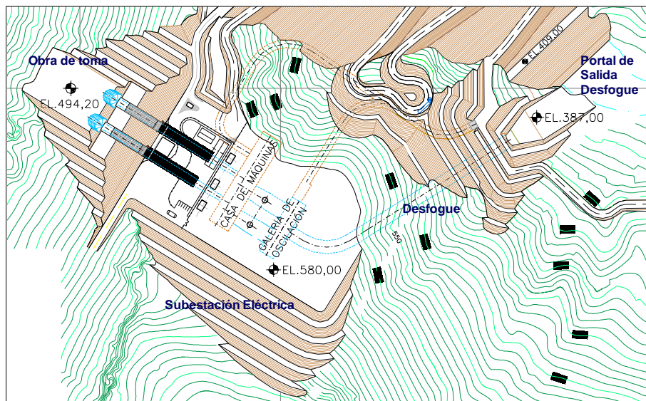
Figura 2.7.- Esquema general en planta de las obras de generación.
