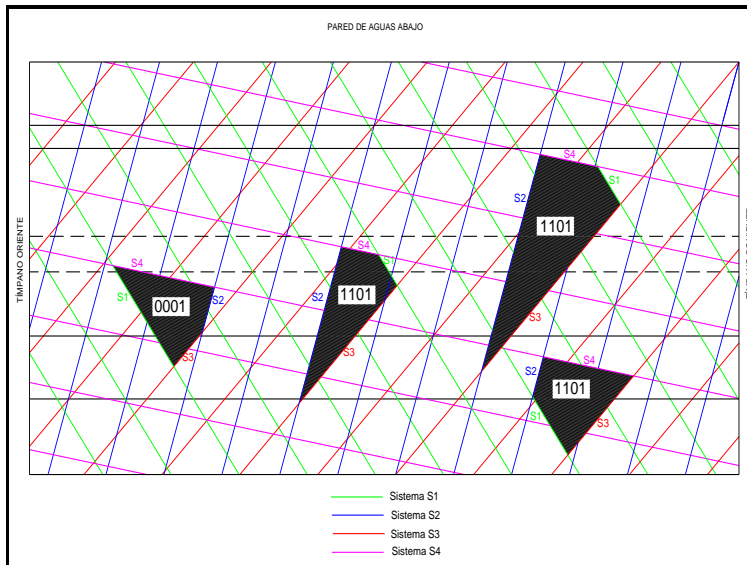
Figura 2.19.- Sección esquemática de la pared de aguas abajo, mostrando los bloques que se formaran, con salida hacia la excavación.
