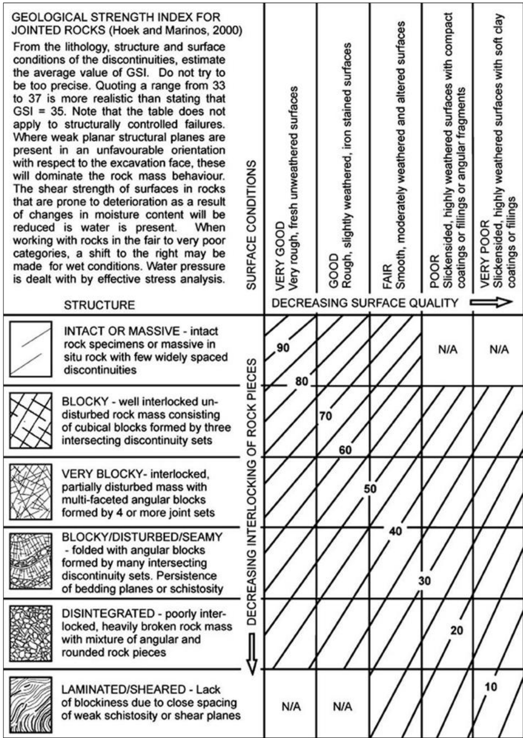
Figura 4.11 C. Clasificación en función del GSI (Hoek y Marinos, 2000).
