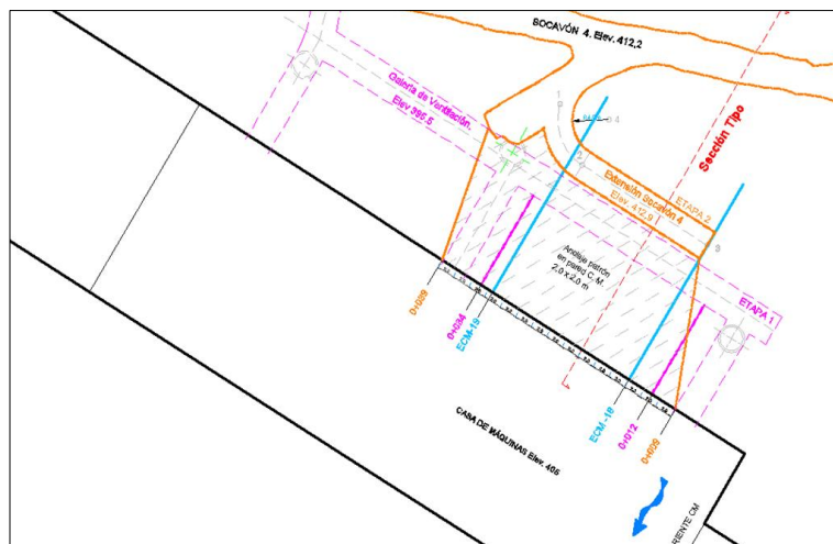
Figura 2.88.- Localización de los socavones para la instalación del anclaje de refuerzo
