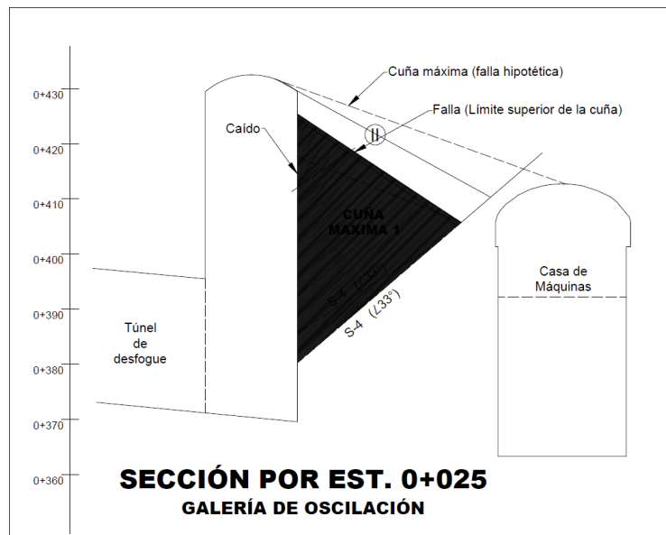
Figura 2.112.- Esquema de cuña máxima tipo 1.
