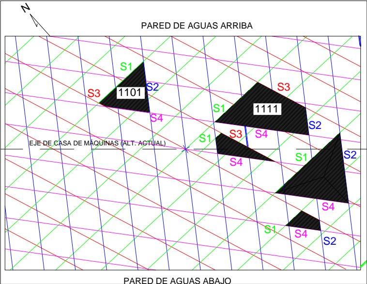
Figura 2.17.- Planta esquemática, que indica la geometría de los bloques que se formarán en la bóveda de la caverna de casa de máquinas.
