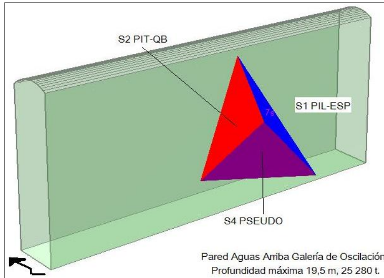
Figura 2.31.- Cuña tipo en pared aguas arriba de galería de oscilación.
