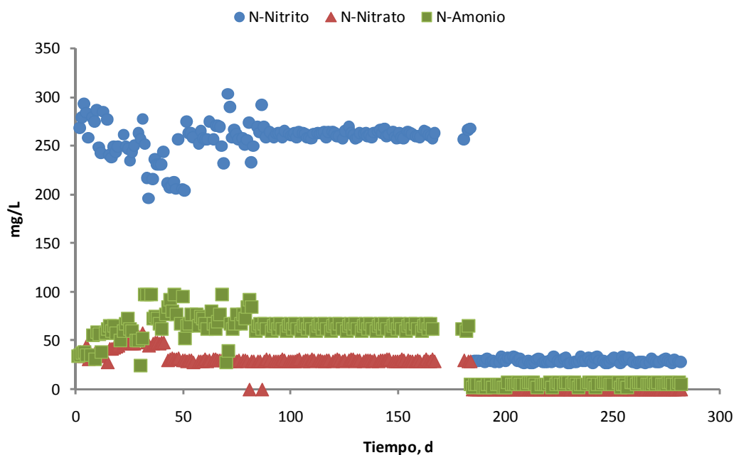
Figura IV.16. Concentración de compuestos nitrogenados en el efluente durante la operación del MSBR.
