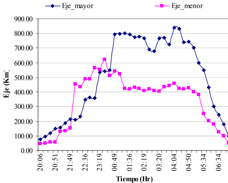
Figura 3.8.- Longitudes de los ejes mayor y menos trazados para la tormenta 07/07/04
