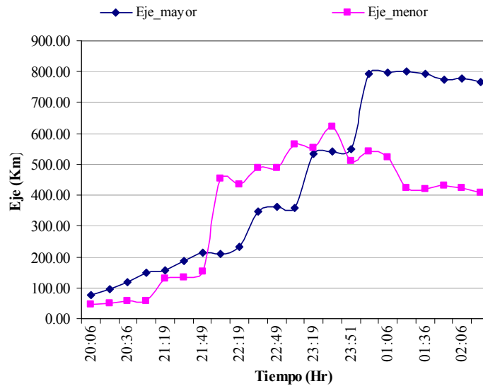
Figura 2.- Longitudes de los ejes mayor y menos trazados para la tormenta 07/07/04. Periodo cercano a la ocurrencia de lluvia
