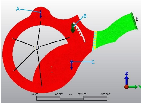
Figura 3.2 Cargas y Restricciones para el análisis del Cuadro (Caso de carga 1)
