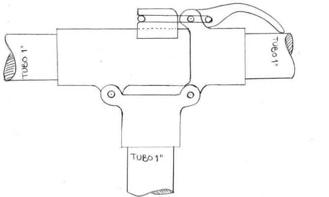
Figura 2.29 Mecanismo de Plegado para barra vertical del Manubrio
