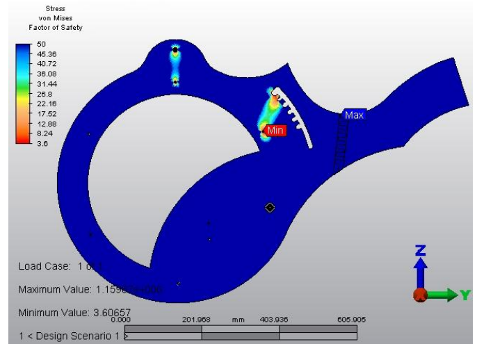
Figura 3.4 Factor de Seguridad en el Cuadro acotado (Caso de carga 1)
