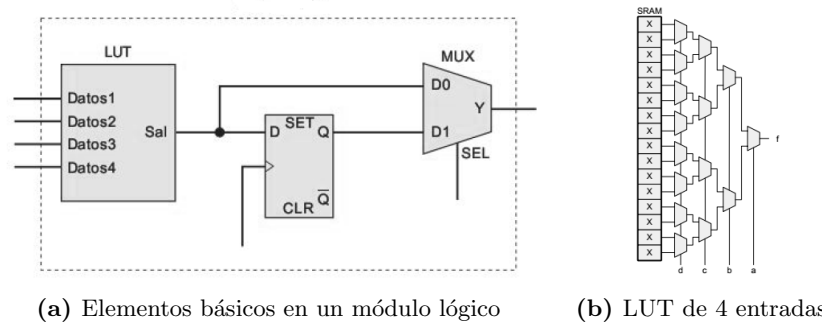
Figura 4.4: Elementos internos de un bloque lógico.
