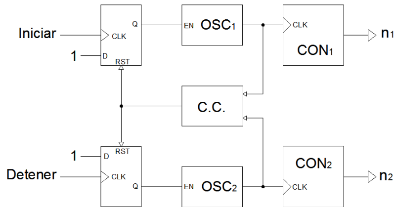
Figura 3.9: Método de Vernier con dos osciladores.
