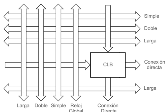
Figura 4.5: Estructura de las interconexiones programables globales.
