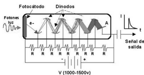
Figura 2.7: Funcionamiento del fotomultiplicador.
