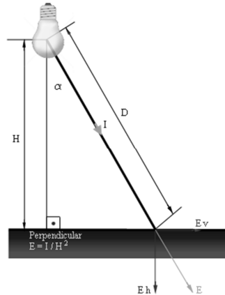
Ilustración 9: Iluminancia horizontal 12
