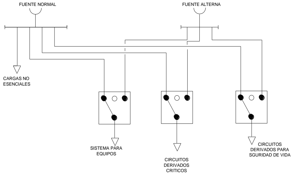
Figura 28. Tal como se indica, el sistema eléctrico puede incluir 3 desconectores de transferencia cuando exceda 150 [kVA], se colocará en este caso un disconector de transferencia para cada circuito derivado.
