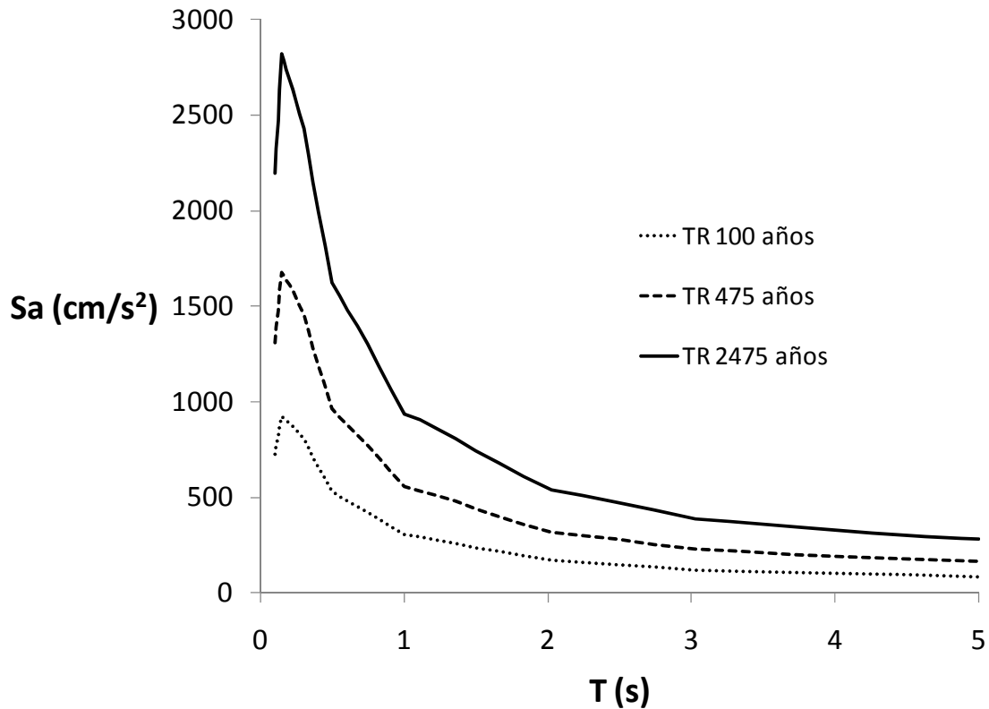
Figura 2.12.- Espectros de peligro uniforme en roca del sitio B.
