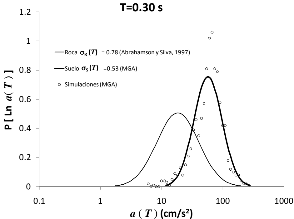
Figura 4.7.- Distribución de probabilidad para un periodo de 0.3 s del sitio A con la relación de atenuación en roca de Abrahamson y Silva (1997) y un sismo de magnitud M igual a 6 a una distancia R de 150 km.
