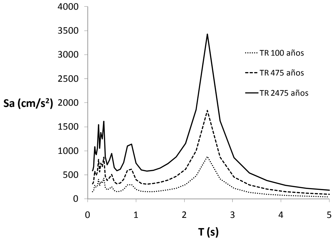
Figura 3.7.- Espectros de respuesta calculados con |H(f)| lineal para el sitio A.
