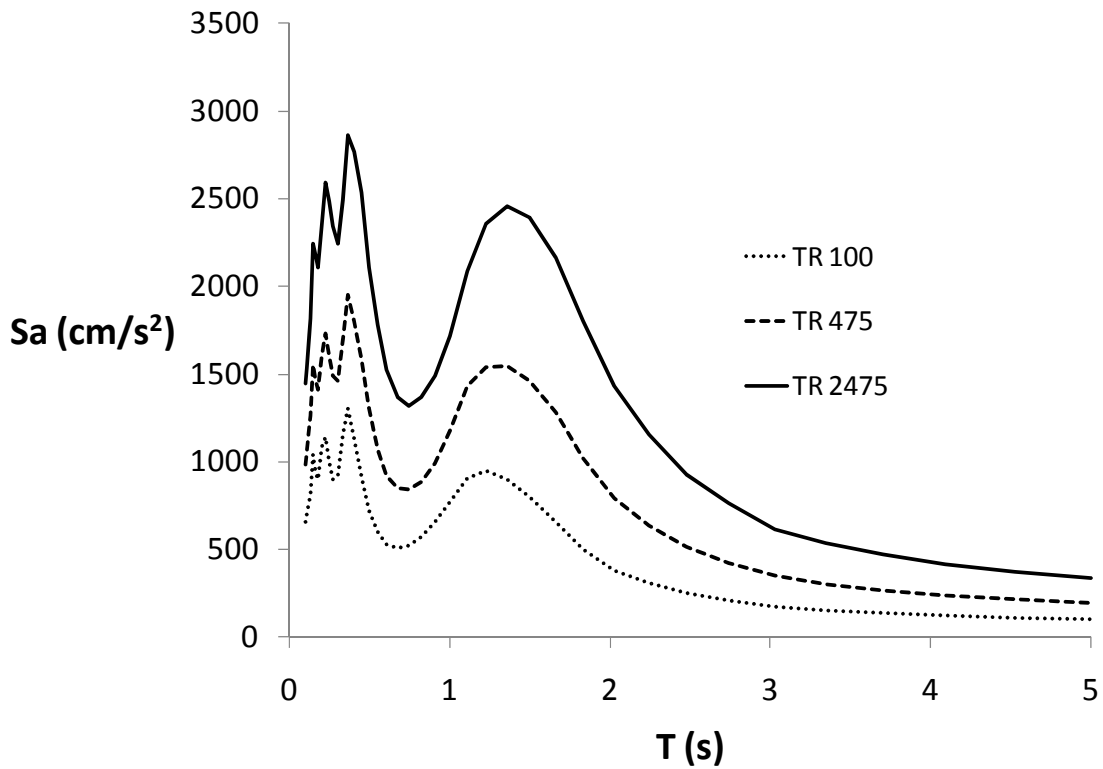
Figura 3.10.- Espectros de respuesta calculados con |H(f)| no-lineal para el sitio B.
