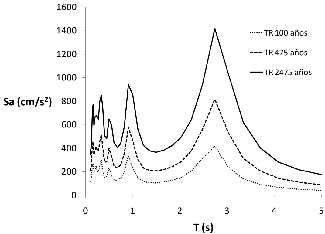
Figura 3.8.- Espectros de respuesta calculados con |H(f)| no-lineal para el sitio A.
