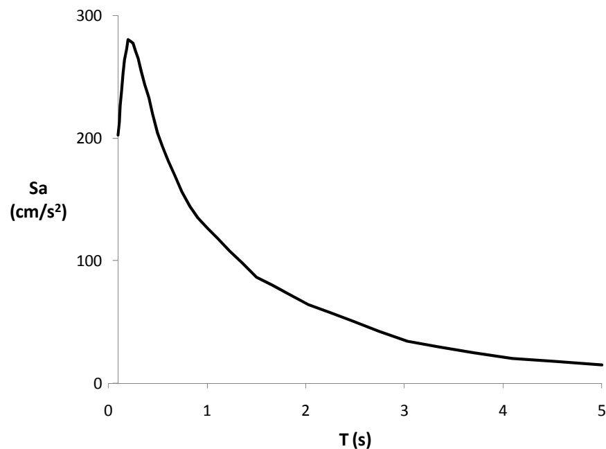
Figura 3.3.- Espectros de respuesta para un sismo de magnitud M igual a 7.5 a una distancia de 50 Km.
