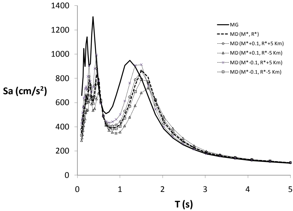
Figura 4.12.- EPU del sitio B para un periodo de retorno de 100 años con base en los resultados del MD y M^* \pm 0.1 y distancias R^* \pm 5 Km.
