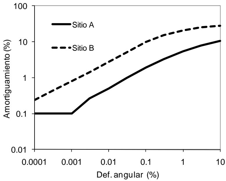
Figura 2.5.- Amortiguamiento vs deformación angular.
