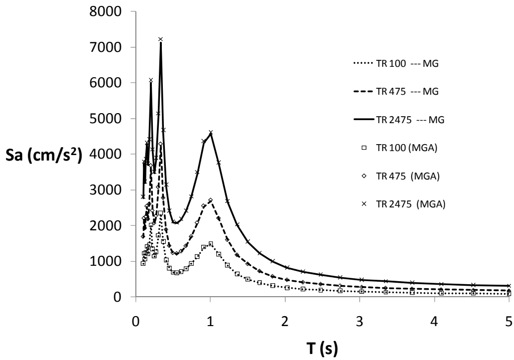
Figura 3.14.- Comparación de los espectros de respuesta del sitio B calculados con la función de transferencia |H(f)| lineal para el MG y el MGA.
