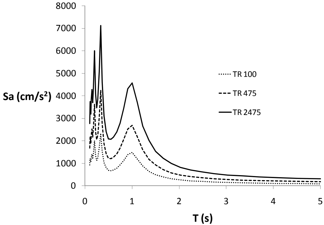
Figura 3.9.- Espectros de respuesta calculados con |H(f)| lineal para el sitio B.
