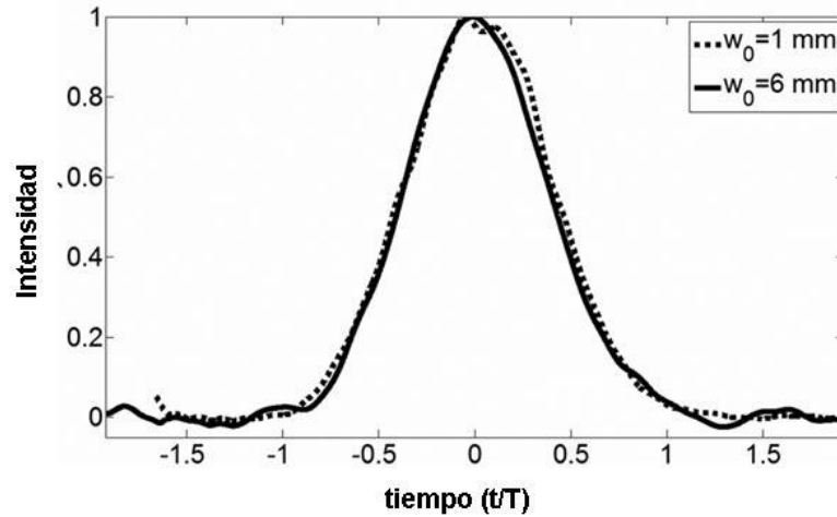
Figura 4.24. Resultados experimentales de la autocorrelacion para un doblete acromático
