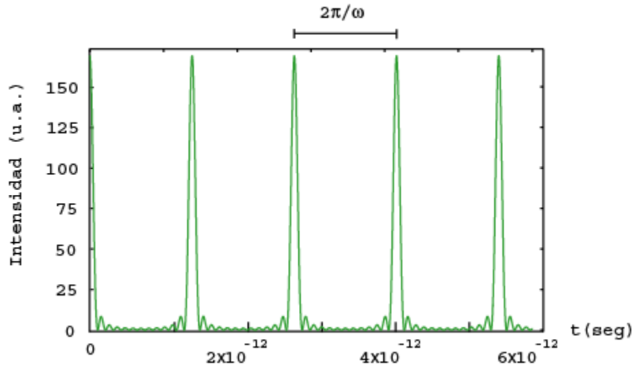
Figura 1.4 Intensidad de salida de un láser de pulsos, ecuación 1.6.
