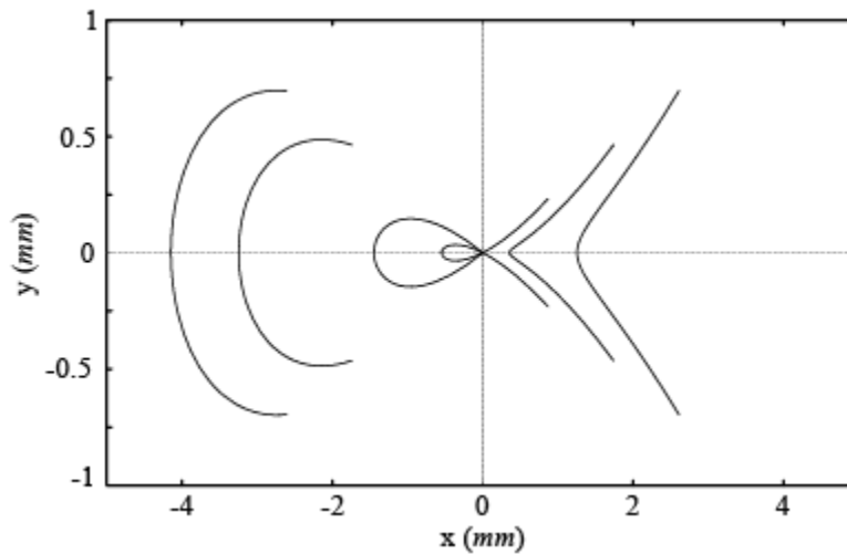
Figura 2.11 Frente del pulso cerca del foco para 249\text{nm} .
