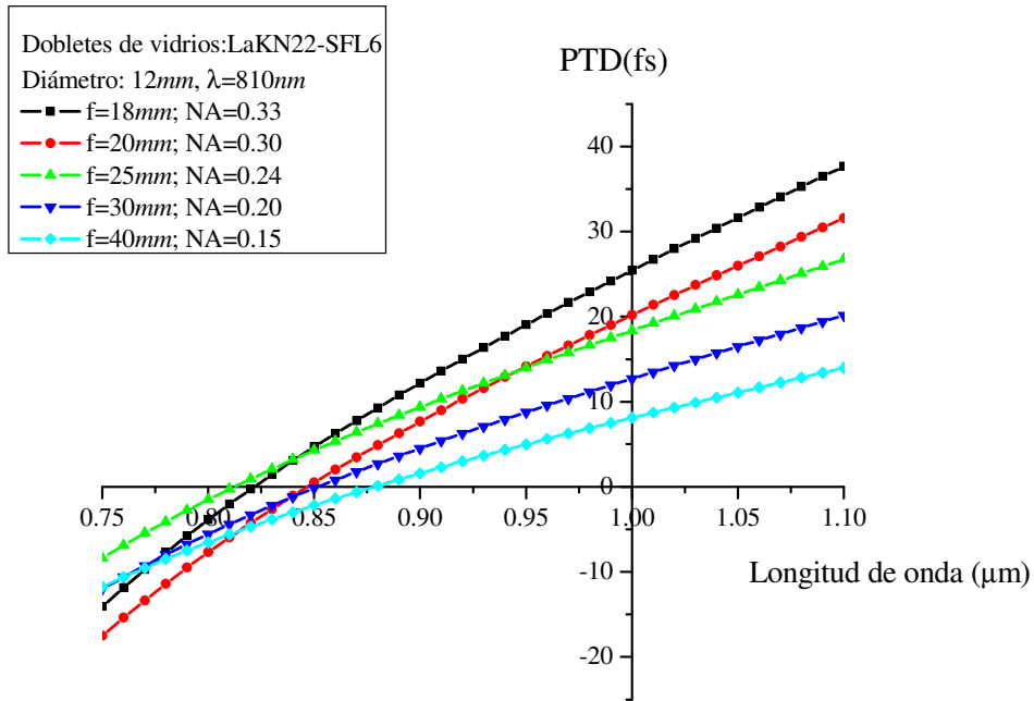
Figura 2.5 Diferencia en el tiempo de propagación, PTD, en función de la longitud de onda para cinco dobletes acromáticos
