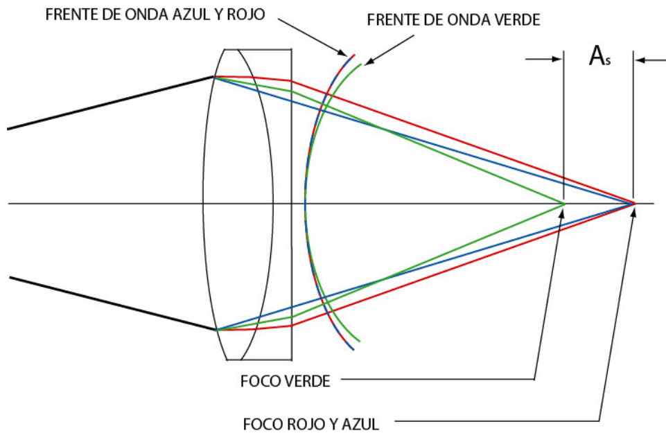
Figura 2.4 Diseño de un doblete acromático real.
