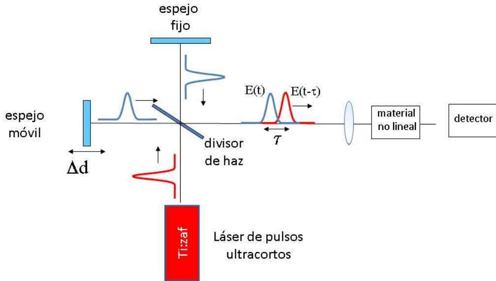
Figura 4.22. Arreglo experimental para la caracterización de pulsos con la técnica SHG.
