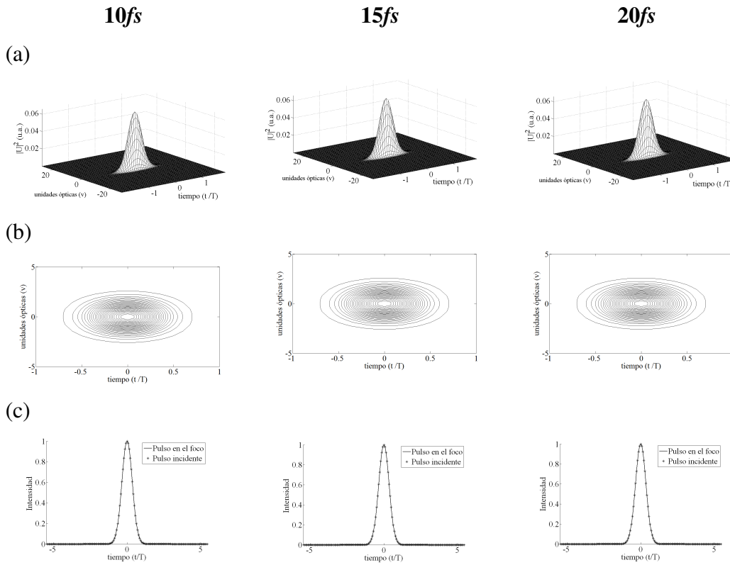
Figura 3.10. Pulsos en el foco paraxial de un doblete acromático ideal, f=18mm . Iluminación Uniforme.
