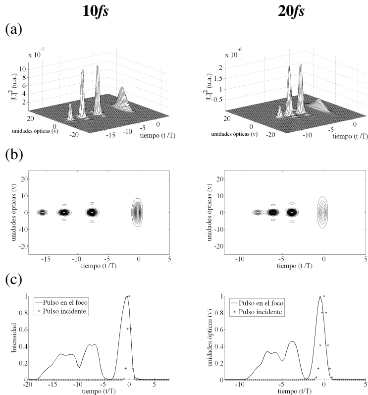
Figura 4.3 Pulso en el foco paraxial de una lente simple, con PTD, aberración esférica y tercer orden, f=18mm . Iluminación uniforme y pulsos incidentes de 10fs y 20fs.
