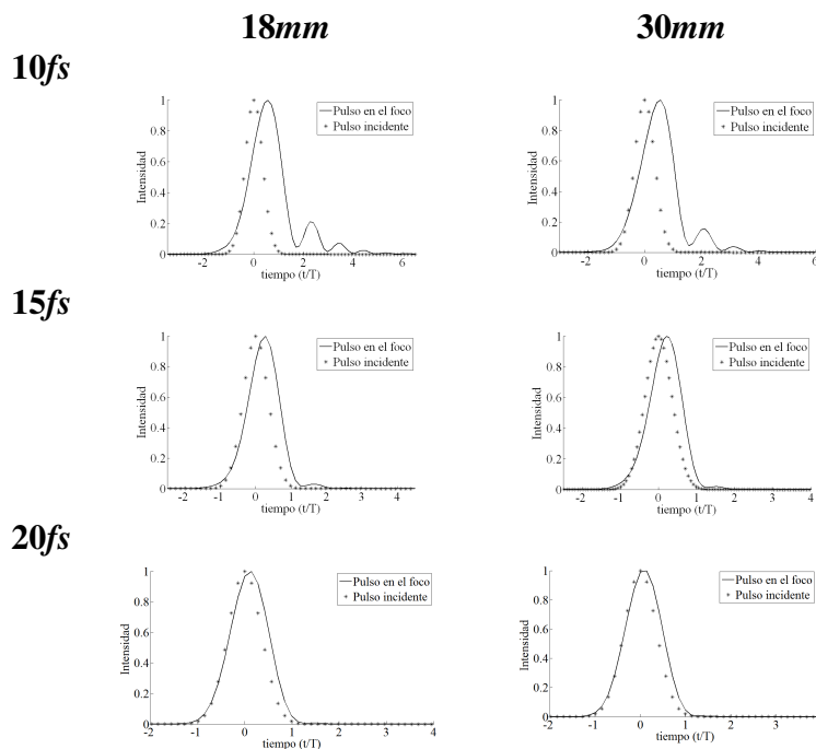
Figura 4.4 Efecto de tercer orden para un dobletes acromáticos, f=18mm y f=30mm . Iluminación uniforme y pulsos incidentes de 10fs , 15fs y 20fs .
