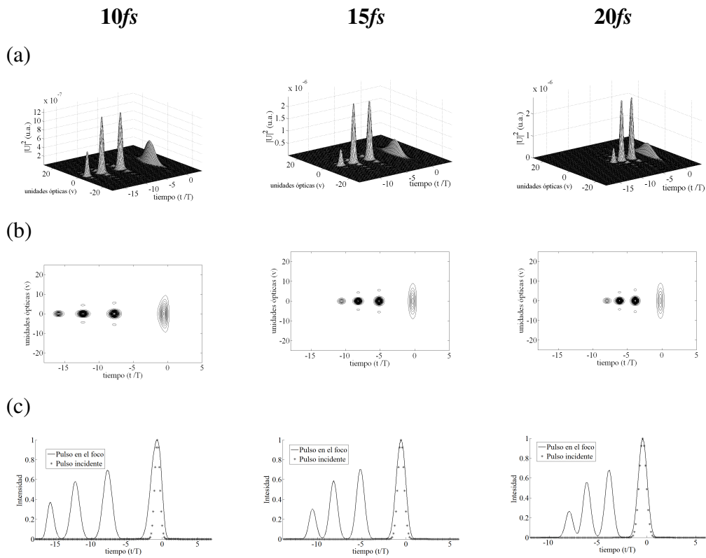
Figura 3.8. Pulsos en el foco paraxial de una lente simple real f=18mm , Iluminación uniforme.
