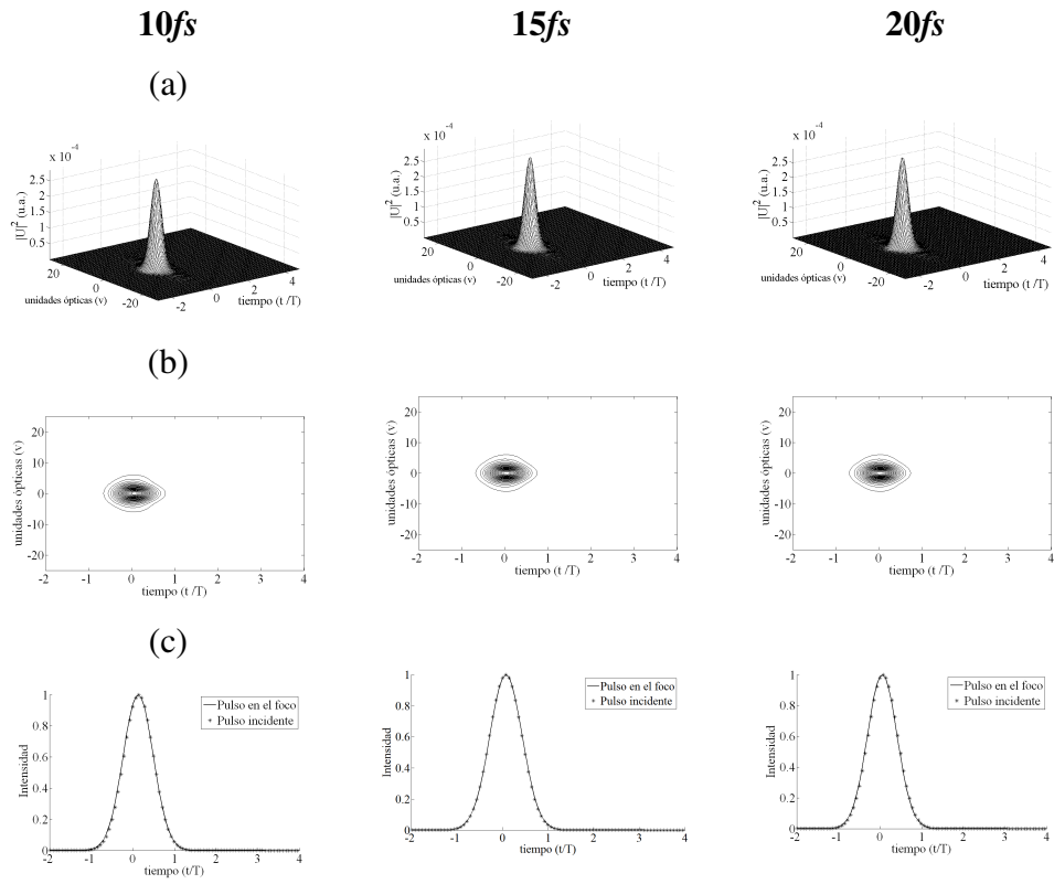
Figura 3.12. Pulsos en el foco paraxial de un doblete acromático real, f= 18mm . Iluminación uniforme.
