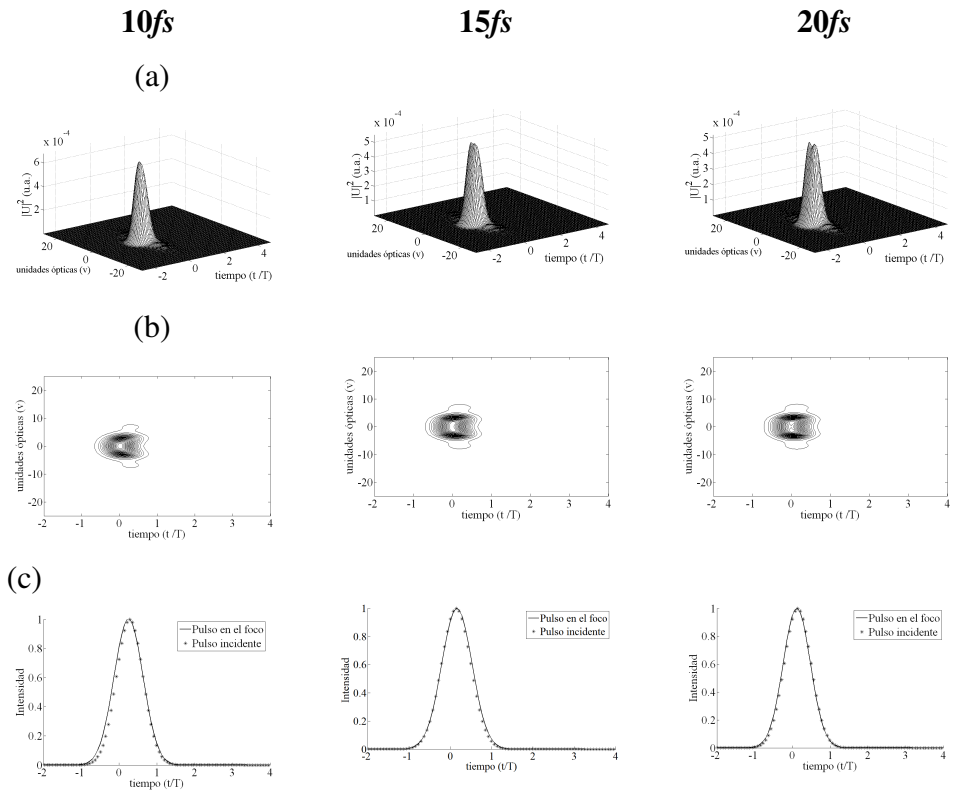
Figura 3.13. Pulsos en el foco paraxial de un doblete acromático real, f= 30mm . Iluminación uniforme.
