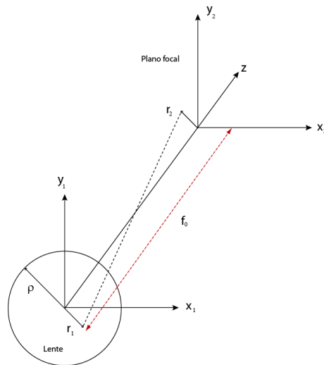
Figura 4.1 sistema de coordenadas en el plano de la lente y en el plano focal.
