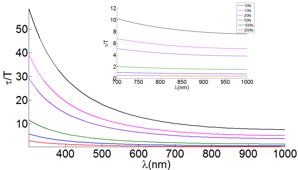
Figura 3.18. \tau/T vs \lambda , producida por una lente simple BK7 y f=30mm , para diferentes anchos temporales incidentes.
