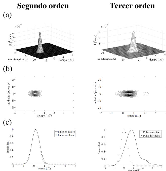
Figura 4.19 Pulsos en el foco paraxial de un doblete acromático real. Segundo y tercer orden, f=30mm . Iluminación Gaussiana y pulsos incidentes de 10fs .
