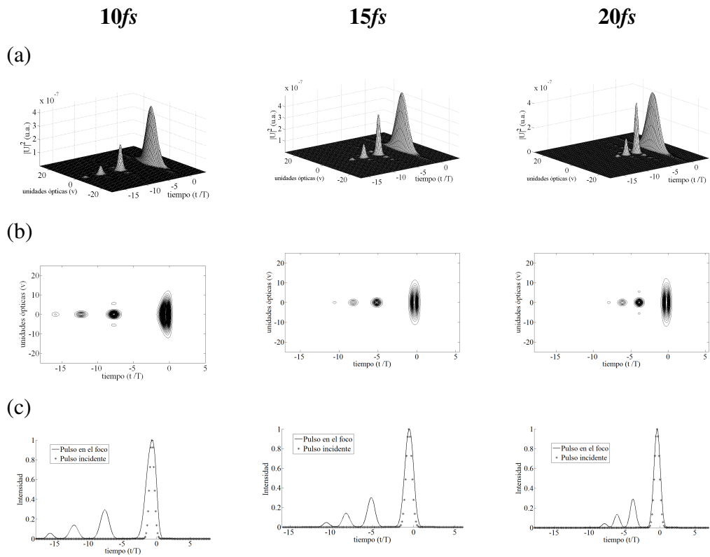
Figura 3.6. Pulsos en el foco paraxial de una lente simple real f=18mm . Iluminación Gaussiana.
