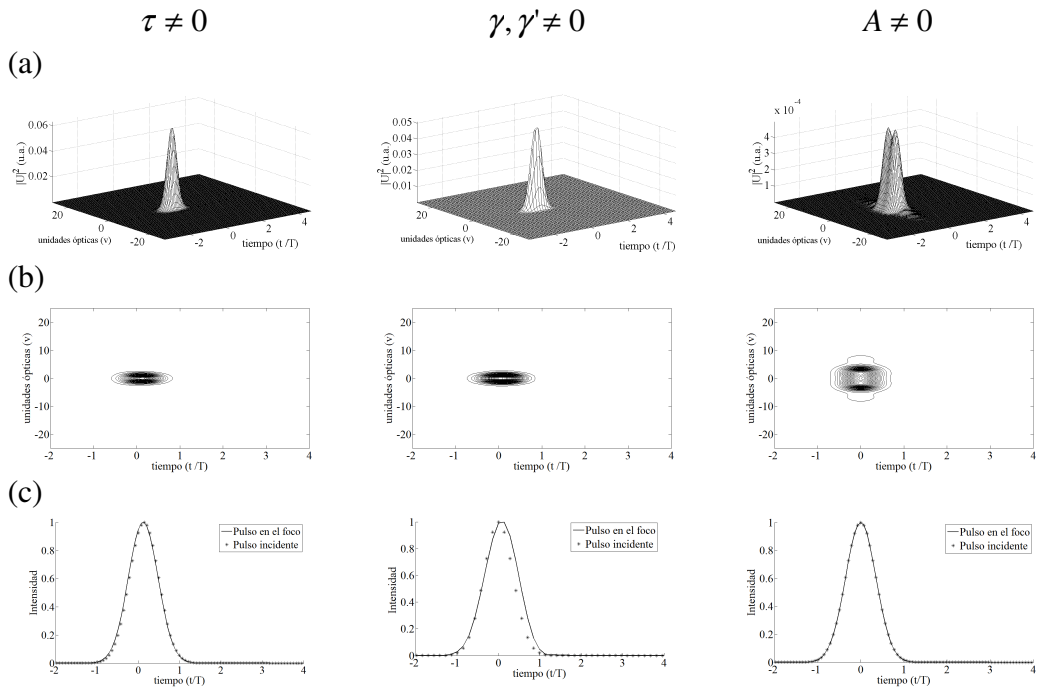
Figura4.8 PTD, tercer orden y aberración esférica para un doblete acromático, f = 30mm . Iluminación uniforme y un pulso incidente de 20fs
