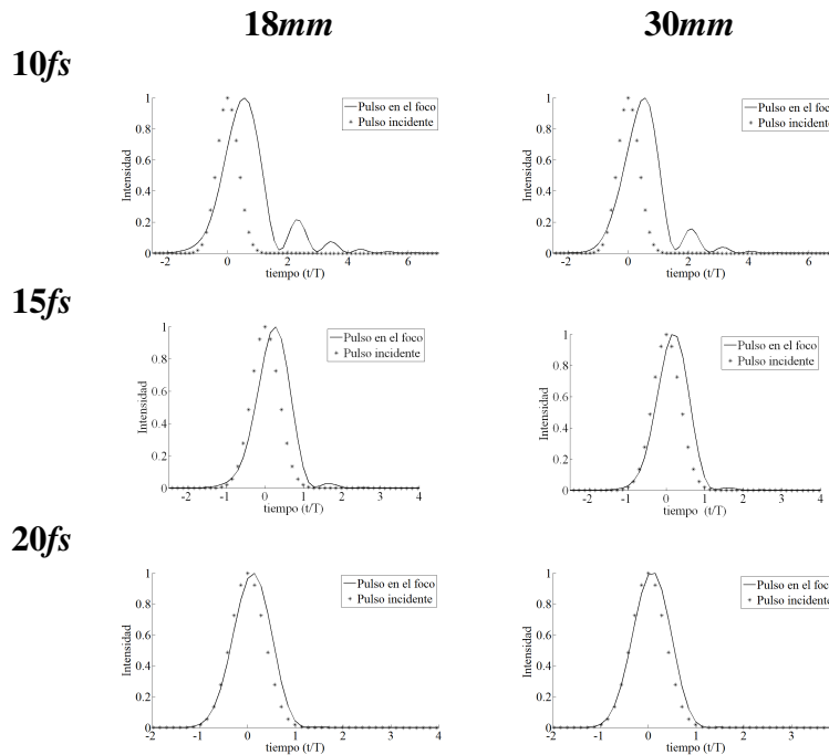
Figura 4.13 Efecto de tercer orden para un dobletes acromáticos, f=18mm y f=30mm . Iluminación Gaussiana y pulsos incidentes de 10fs , 15fs y 20fs .
