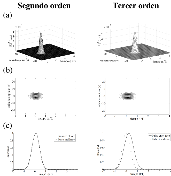
Figura 4.21 Pulsos en el foco paraxial de un doblete acromático real. Segundo y tercer orden, f=30mm . Iluminación Gaussiana y pulsos incidentes de 20fs .
