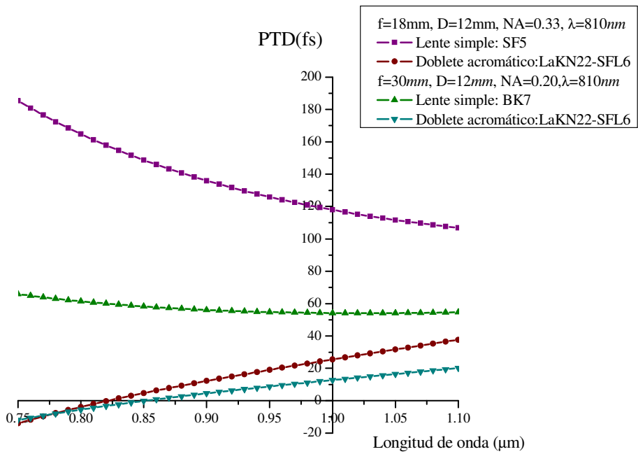
Figura 2.6 Comparación del efecto de PTD, para dos lentes simples y dos dobletes acromáticos que tienen las mismas aperturas numéricas que las lentes simples.
