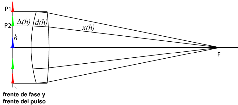
Figura 2.1 Lente simple en la cual incide sobre ella un haz de luz pulsada.
