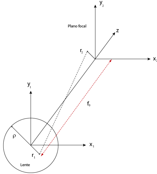
Figura 3.1. sistema de coordenadas en el plano de la lente y en el plano focal.
