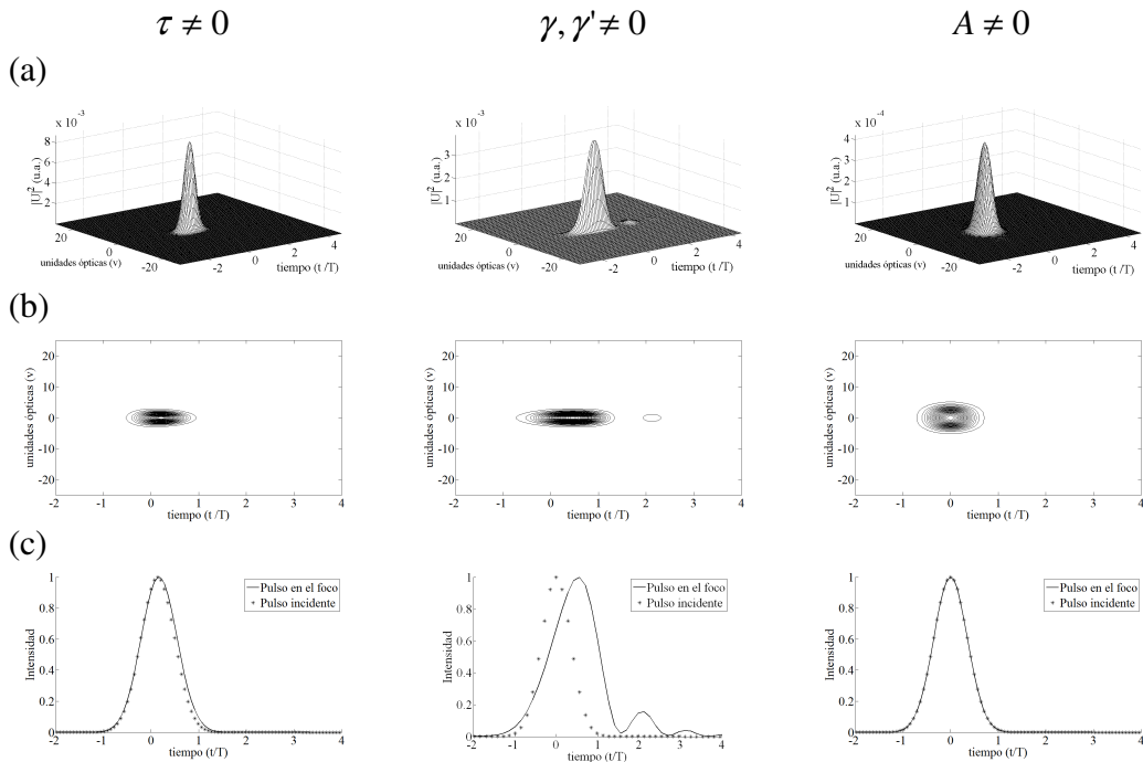
Figura 4.15 PTDT, tercer orden y aberración esférica para un doblete acromático, f= 30mm . Iluminación Gaussiana y un pulso incidente de 10fs
