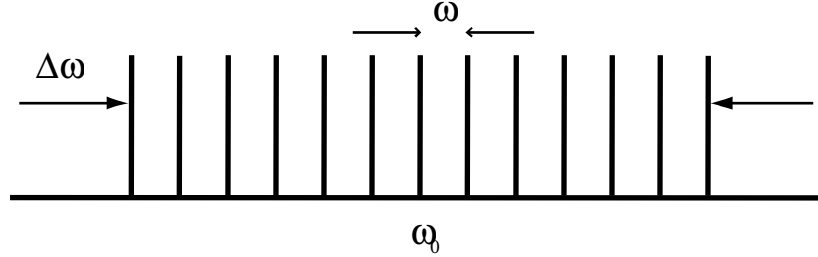
Figura 1.3. Modos de oscilación en un láser.
