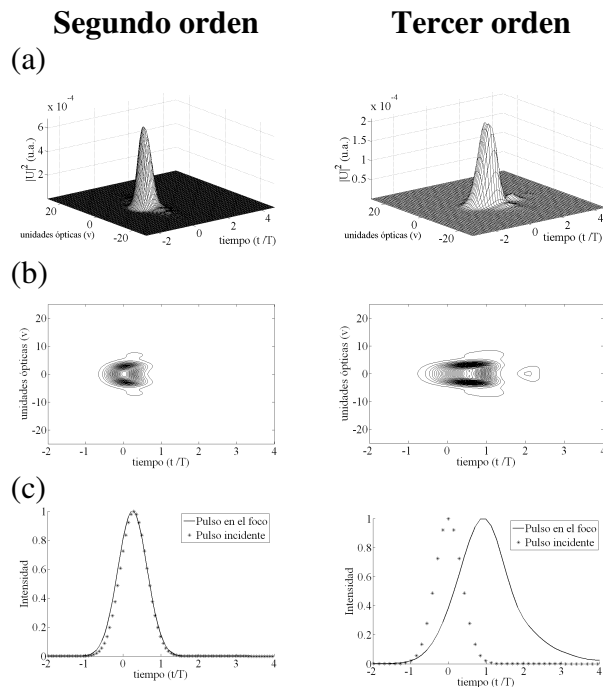
Figura 4.10. Pulsos en el foco paraxial de un doblete acromático real. Segundo y tercer orden, f=30mm . Iluminación uniforme y pulso incidente de 10fs .
