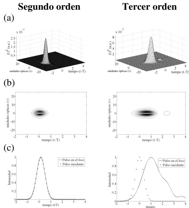
Figura 4.9. Pulsos en el foco paraxial de un doblete acromático real. segundo y tercer orden, f=18mm . Iluminación uniforme y pulso incidente de 10fs .
