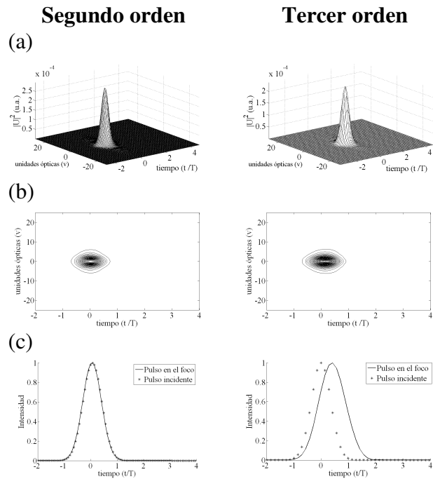
Figura 4.11 Pulsos en el foco paraxial de un doblete acromático real. Segundo y tercer orden, f=18mm . Iluminación uniforme y pulsos incidentes de 20fs .
