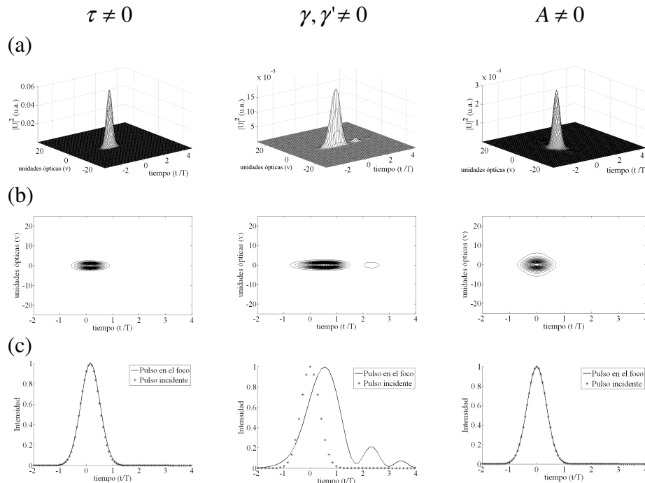
Figura 4.5 PTD, tercer orden y aberración esférica para un doblete acromático, f=18mm . Iluminación uniforme y un pulso incidente de 10fs
