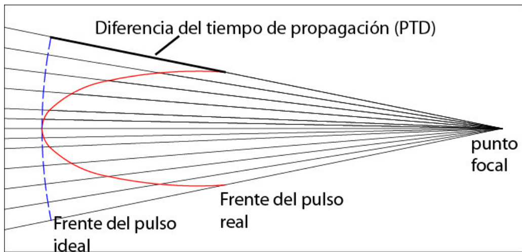
Figura 2.2 Ampliación de la zona focal para mostrar (a) el frente del pulso real, línea en color rojo y (b) el frente del pulso ideal, línea en color azul.
