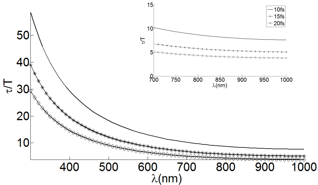
Figura 3.17. \tau/T producida por una lente simple de vidrio BK7 con distancia focal de 30mm como función de la longitud de onda de la portadora en el intervalo 300nm a 1100nm , para pulsos de 10fs , 15fs y 20fs .
