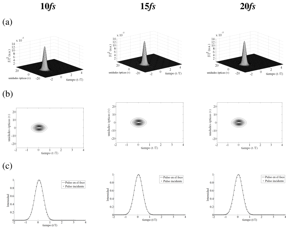
Figura 3.14. Pulsos en el foco paraxial de un doblete acromático real, f= 18mm . Iluminación Gaussiana.
