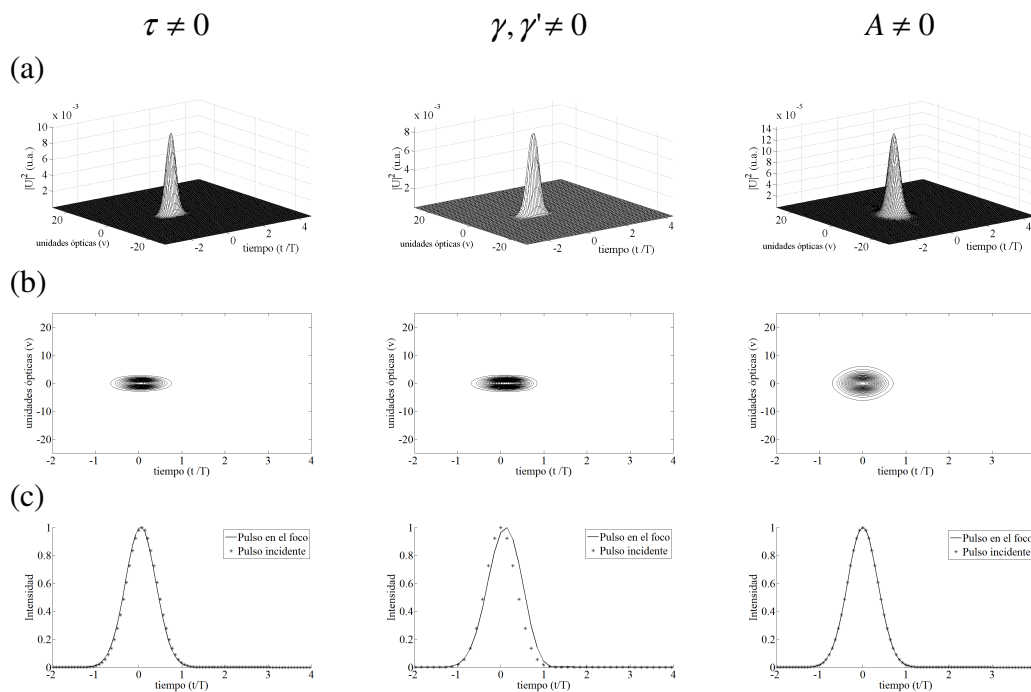
Figura 4.16 PTD, tercer orden y aberración esférica para un doblete acromático, f= 18mm . Iluminación Gaussiana y un pulso incidente de 20fs
