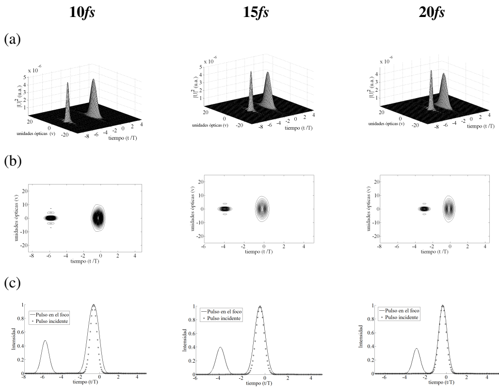
Figura 3.9. Pulsos en el foco paraxial de una lente simple real, f=30mm . Iluminación Uniforme.
