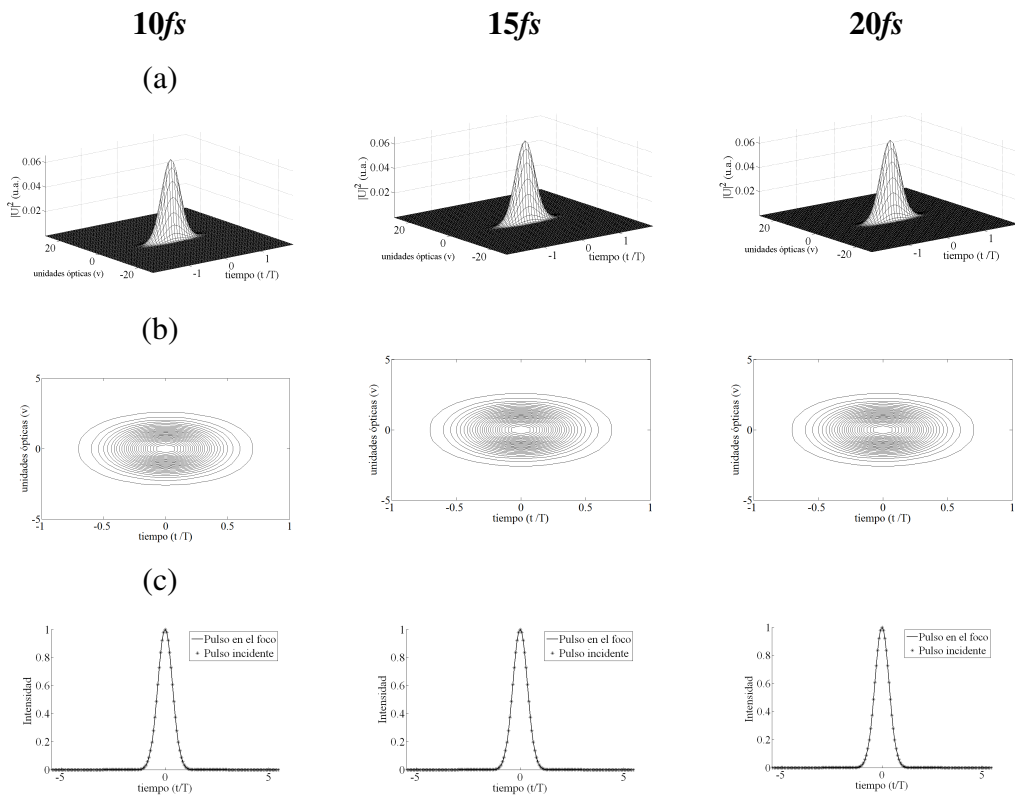
Figura 3.11. Pulsos en el foco paraxial de un doblete acromático ideal, f=30mm . Iluminación Uniforme.
