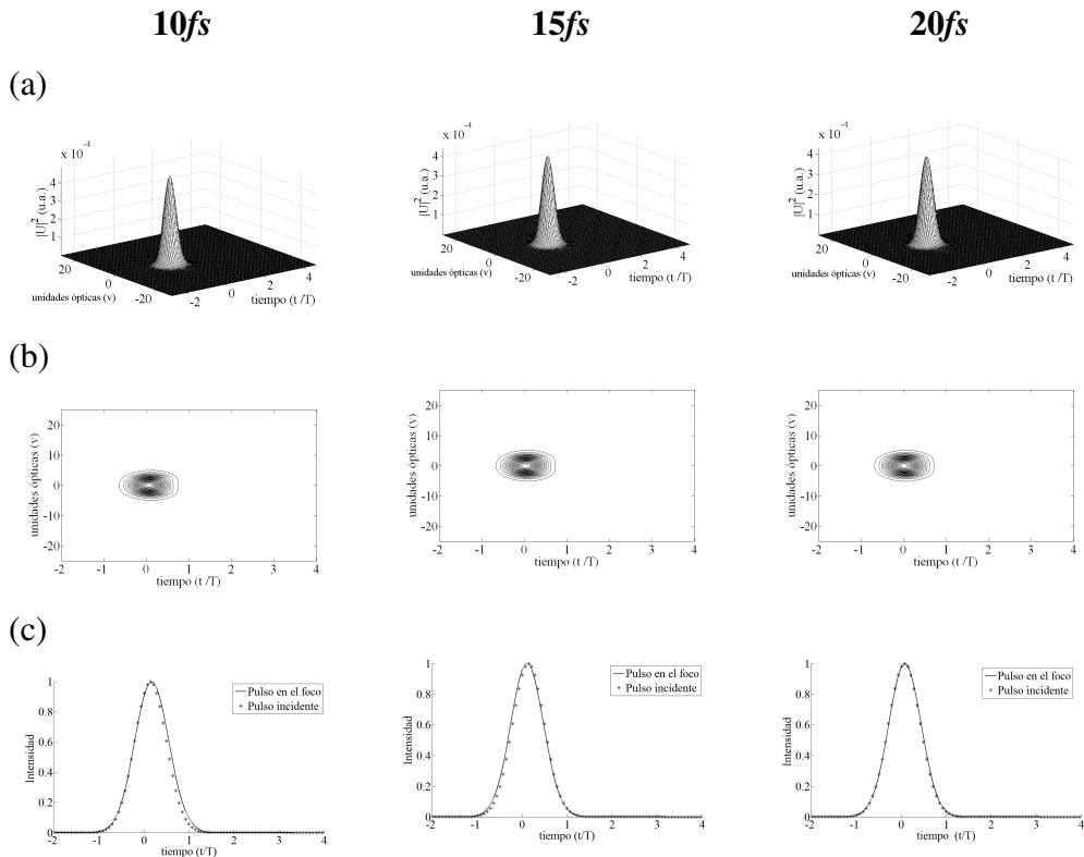
Figura 3.15. Pulsos en el foco paraxial de un doblete acromático real, f= 30mm . Iluminación Gaussiana.
