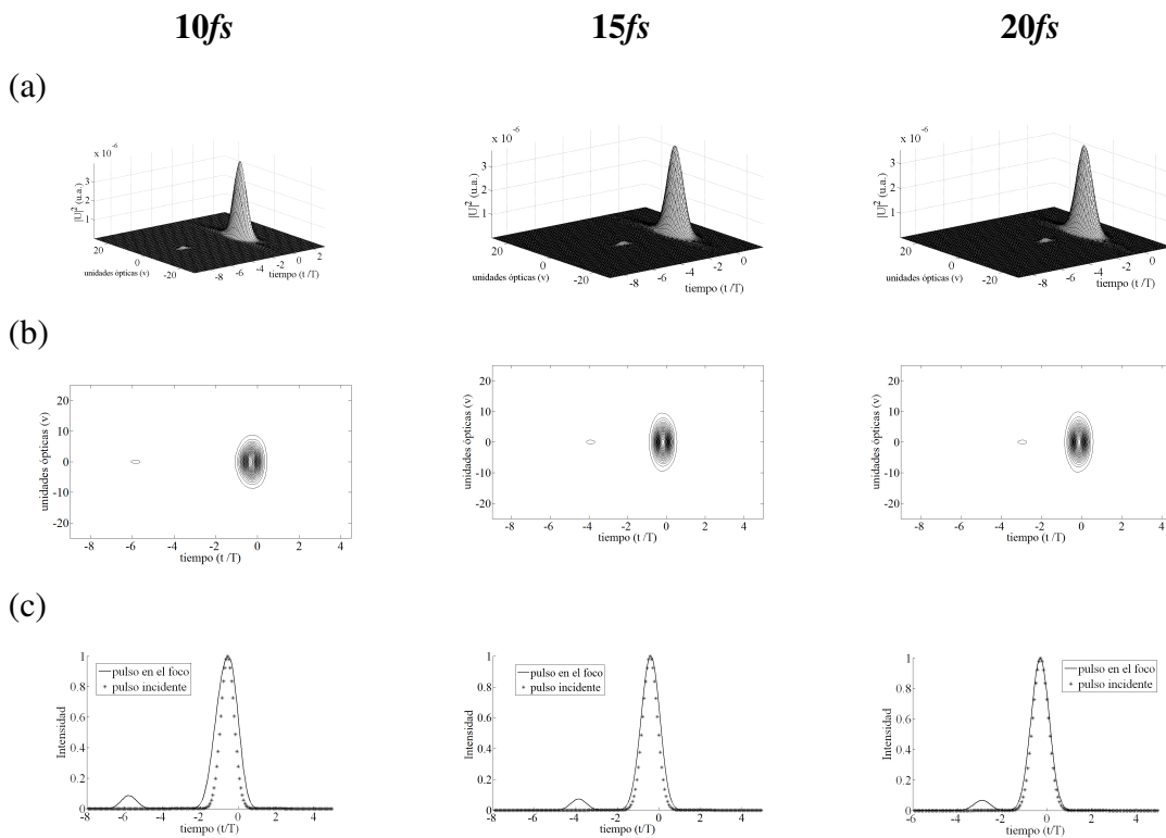
Figura 3.7. Pulsos en el foco paraxial de una lente simple real f=30mm . Iluminación Gaussiana.
