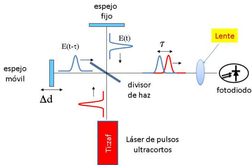
Figura 4.23. Arreglo experimental para la caracterización lentes y pulsos ultracortos con la técnica TPA.
