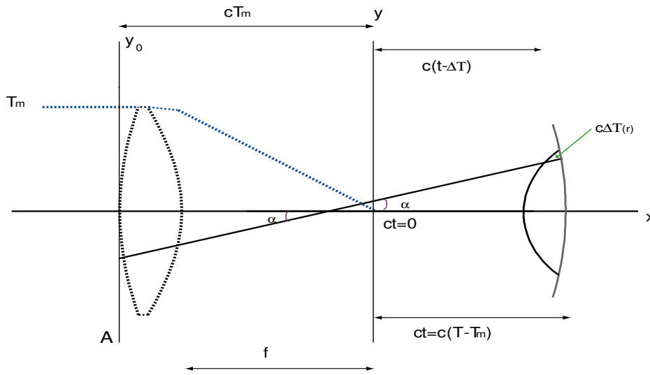
Figura 2.7 Deducción de las ecuaciones del frente del pulso y frente de fase.
