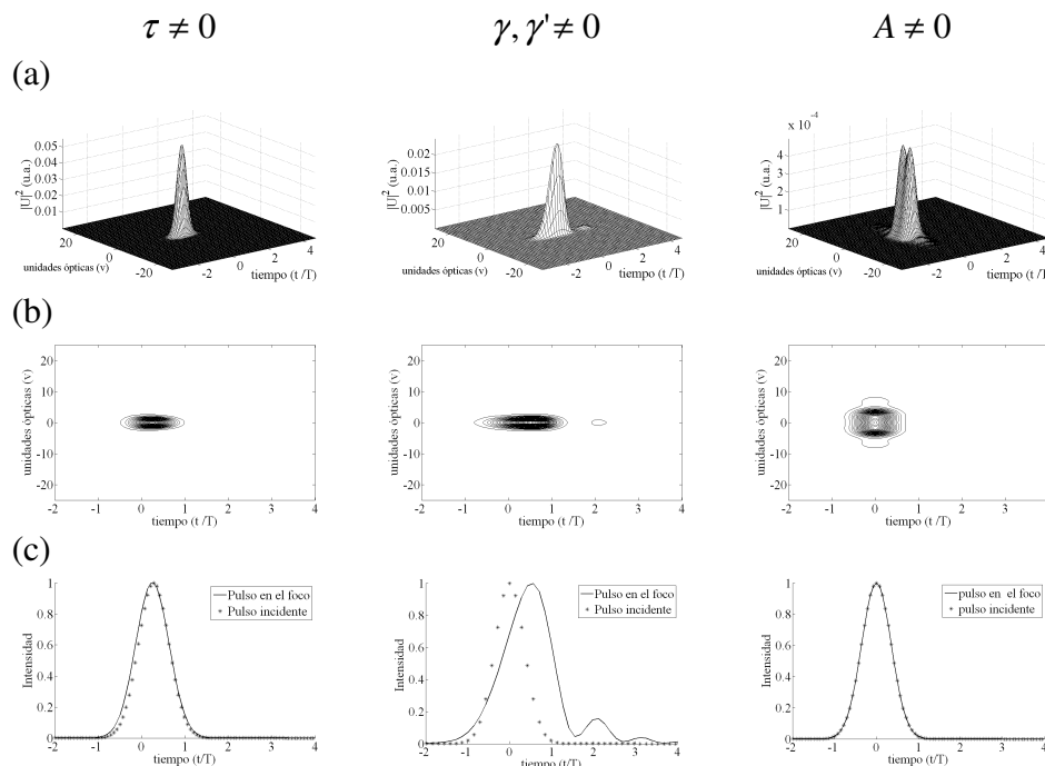
Figura 4.6 PTD, tercer orden y aberracion esférica para un doblete acromático, f= 30mm . Iluminación uniforme y un pulso incidente de 10fs
