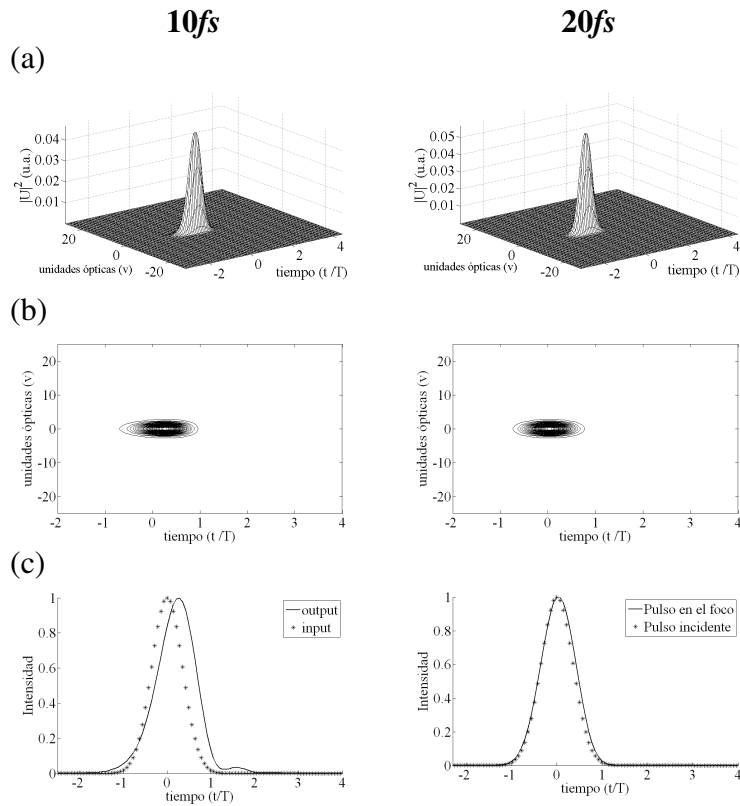
Figura 4.2 Efecto de tercer orden para una lente simple, f= 18mm . Iluminación uniforme y pulsos incidentes de 10fs y 20fs .
