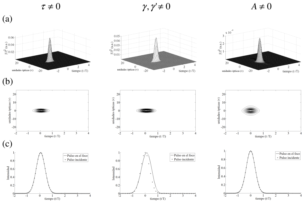
Figura4.7 PTD, tercer orden y aberración esférica para un doblete acromático, f = 18mm . Iluminación uniforme y un pulso incidente de 20fs
