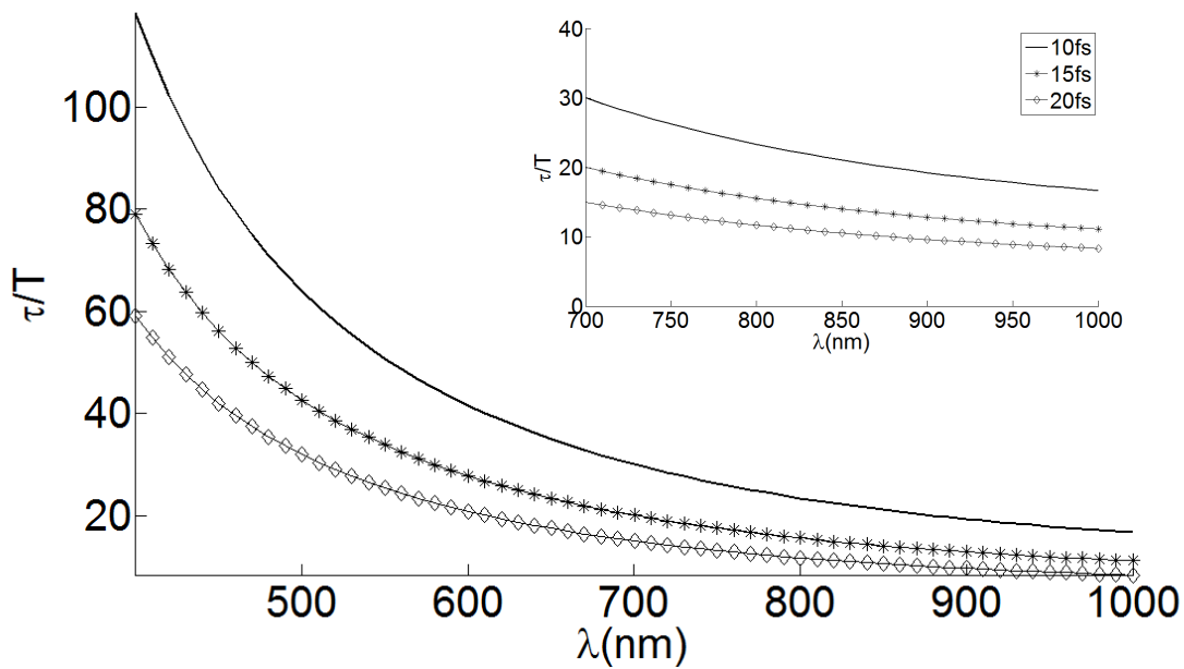
Figura 3.16. \tau/T producida por una lente simple de vidrio SF5 con distancia focal de 18\text{mm} como función de la longitud de onda de la portadora en el intervalo 300\text{nm} y 1100\text{nm} , para pulsos de 10\text{fs} , 15\text{fs} y 20\text{fs} .
