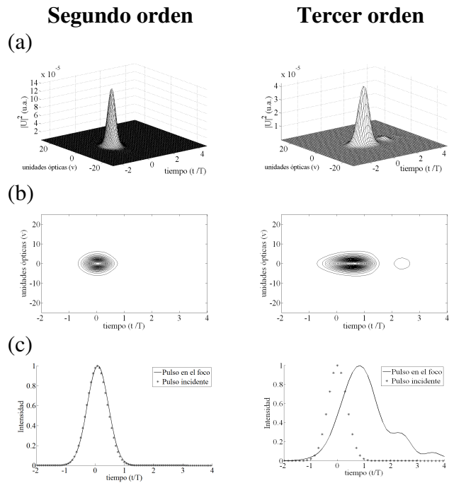
Figura 4.18 Pulsos en el foco paraxial de un doblete acromático real. Segundo y tercer orden, f=18mm . Iluminación Gaussiana y pulsos incidentes de 10fs .
