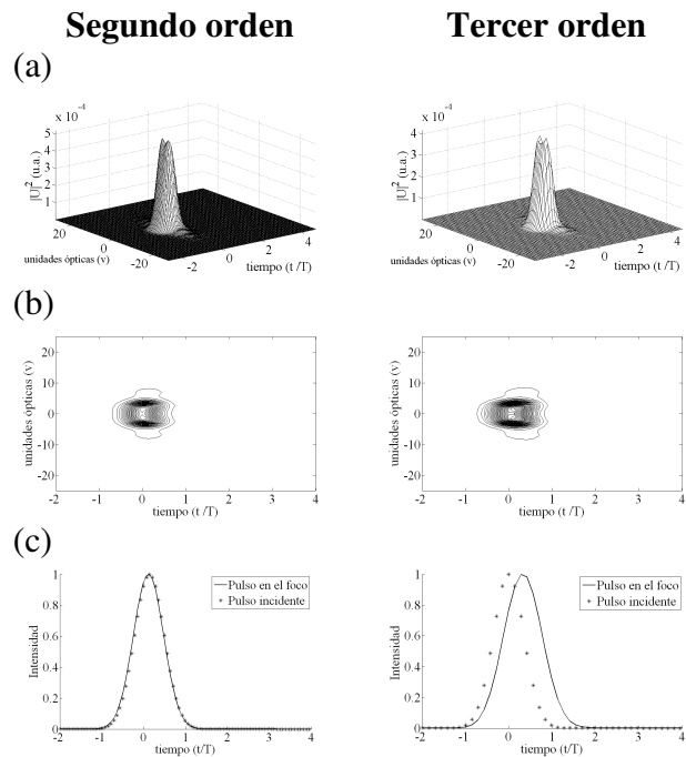
Figura 4.12 Pulsos en el foco paraxial de un doblete acromático real. Segundo y tercer orden, f=30mm . Iluminación uniforme y pulsos incidentes de 20fs .
