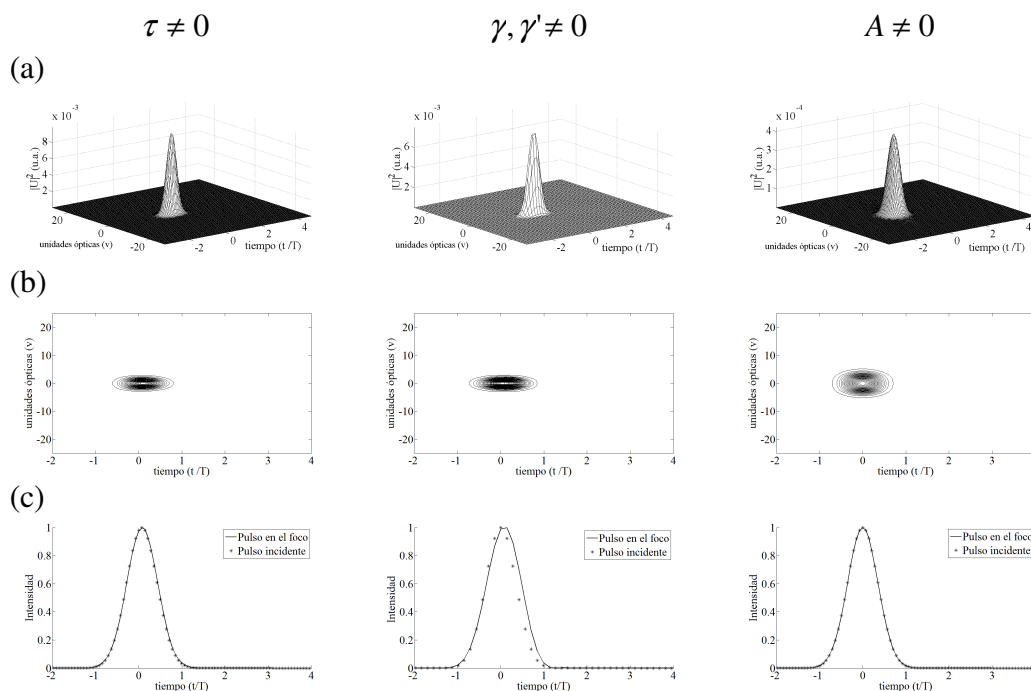
Figura 4.17 PTD, tercer orden y aberración esférica para un doblete acromático, f= 30mm . Iluminación Gaussiana y un pulso incidente de 20fs
