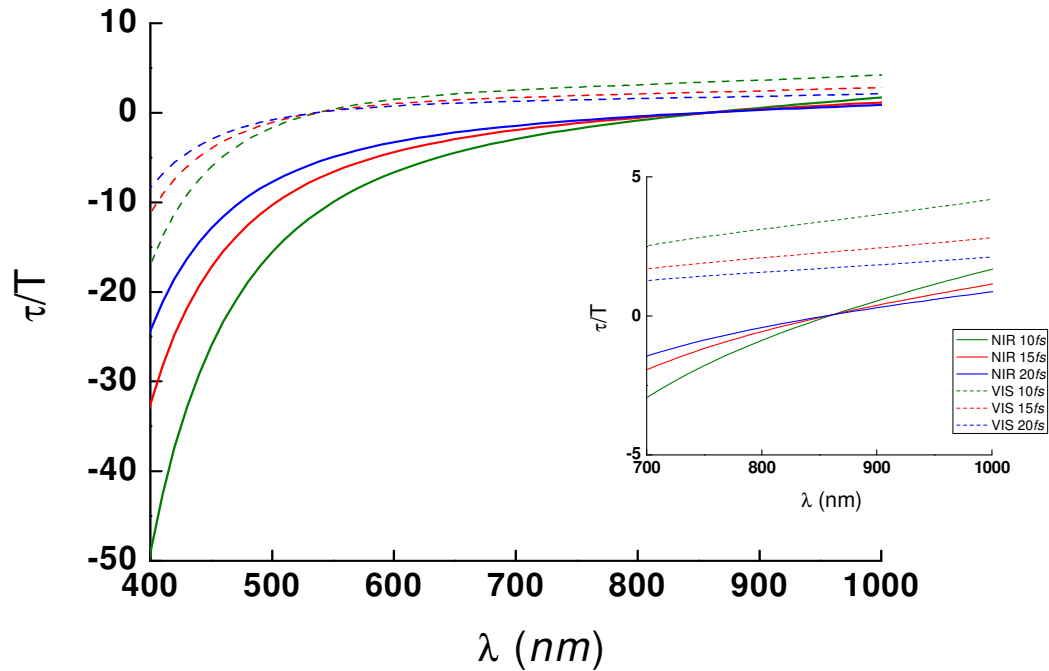
Figura 3.21. Comparación de \tau/T vs \lambda , para dos dobletes acromáticos de distancia focal f=30mm : uno diseñado en el VIS entre 486.1nm y 656.3nm y otro diseñado en el IR entre 700nm y 1100nm , para diferentes anchos temporales incidentes.
