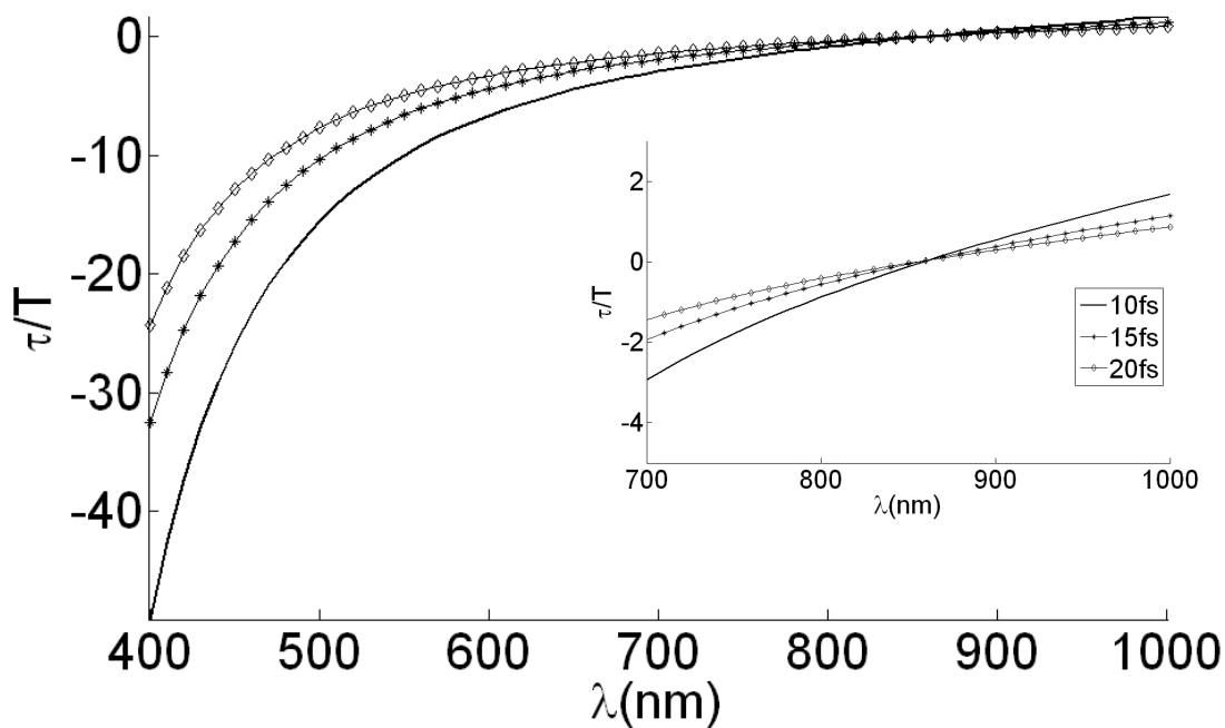
Figura 3.19. \tau/T vs \lambda , producida por un doblete acromático diseñado en el IR entre 700\text{nm} y 1100\text{nm} , f=30\text{mm} , para diferentes anchos temporales incidentes
