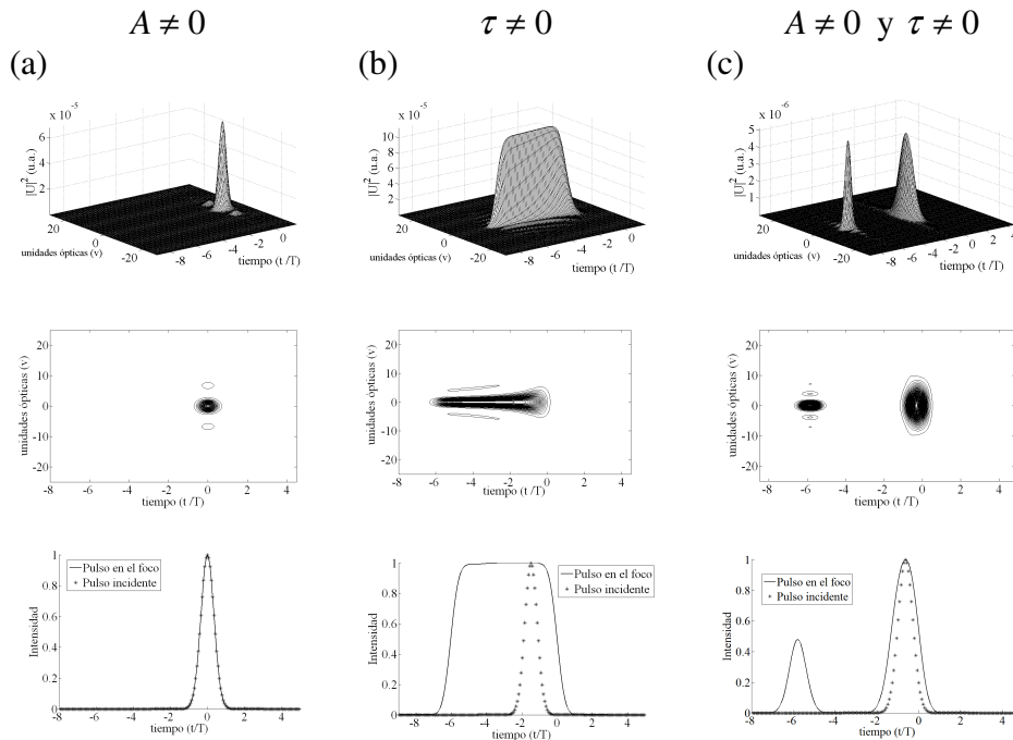
Figura 3.5. Pulso en el foco paraxial de una lente simple f=30mm . (a) PTD=0 , GVD=0 y aberración esférica diferente de cero, (b) GVD=0 y aberración esférica es cero, (c) GVD=0 y PTD aberración esférica son diferentes de cero. Iluminación Uniforme, para 10fs .
