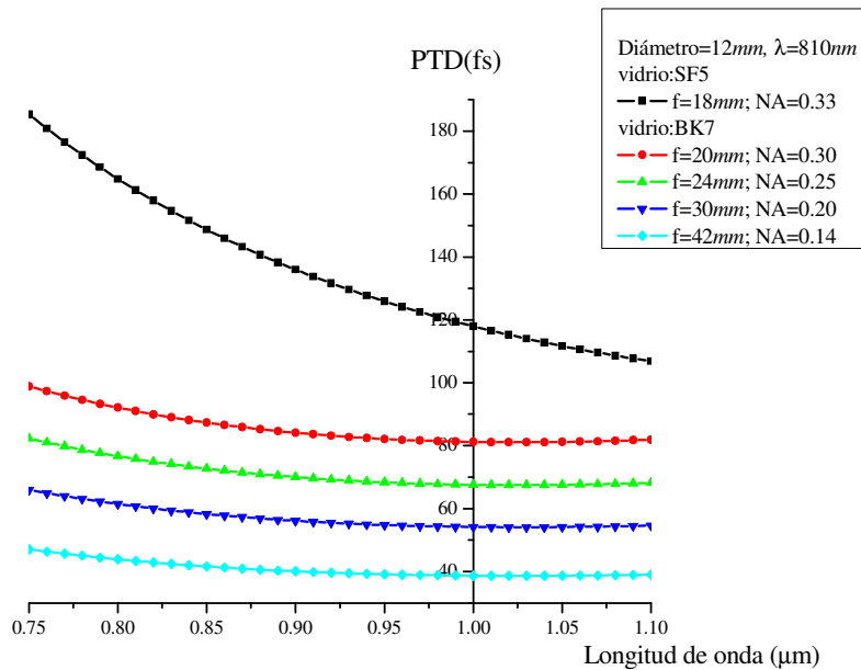
Figura 2.3 Diferencia en el tiempo de propagación, PTD, en función de la longitud de onda para cinco lentes simples.
