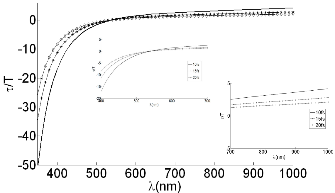
Figura 3.20. \tau/T vs \lambda , producida por un doblete acromático diseñado en el VIS entre 486.1nm y 656.3nm , f=30mm , para diferentes anchos temporales incidentes.
