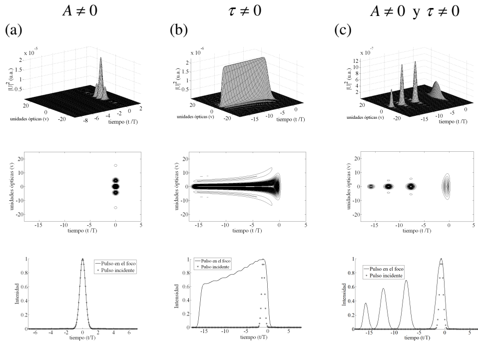
Figura 3.4. Pulso en el foco paraxial de una lente simple f=18mm . (a) PTD=0 , GVD=0 y Aberración esférica diferente de cero, (b) GVD=0 y aberración esférica es cero, (c) GVD=0 PTD y aberración esférica son diferentes de cero. Iluminación Uniforme, para 10fs .
