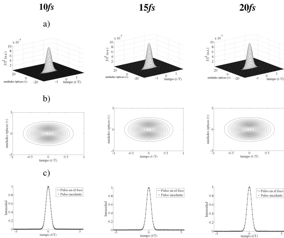
Figura 3.3. Pulsos en el foco paraxial de una lente simple ideal f=30mm . Iluminación Gaussiana.
