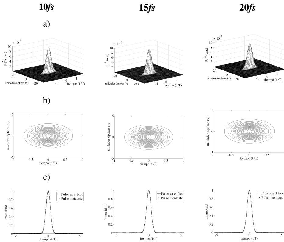
Figura 3.2. Pulsos en el foco paraxial de una lente simple ideal f=18mm . Iluminación Gaussiana.
