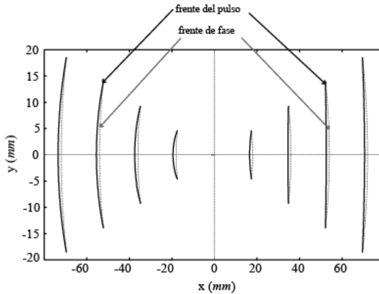
Figura 2.8 Frente de fase y frente del pulso en diferentes momentos para una longitud de onda de 249nm .
