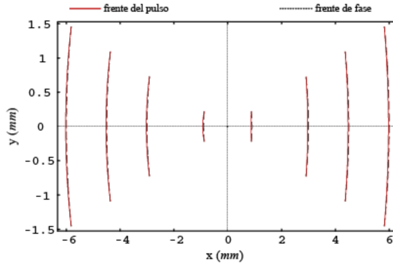
Figura 2.9 Frente de fase y del frente del pulso en diferentes momentos para una longitud de onda de 810\text{nm} .
