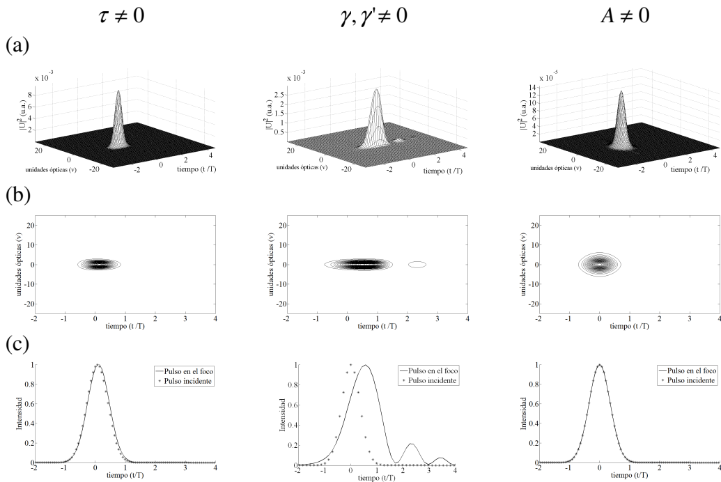
Figura 4.14 PTDT, tercer orden y aberración esférica para un doblete acromático, f= 18mm . Iluminación Gaussiana y un pulso incidente de 10fs
