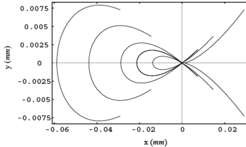
Figura 2.12 Frente del pulso cerca del foco para 810nm .
