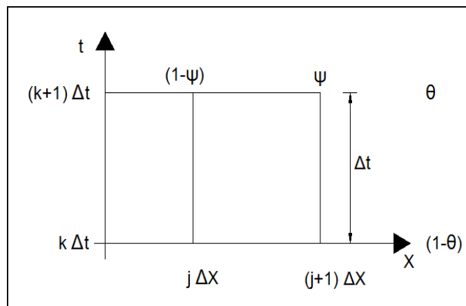
Figura 3.1 Esquema de diferencias finitas
