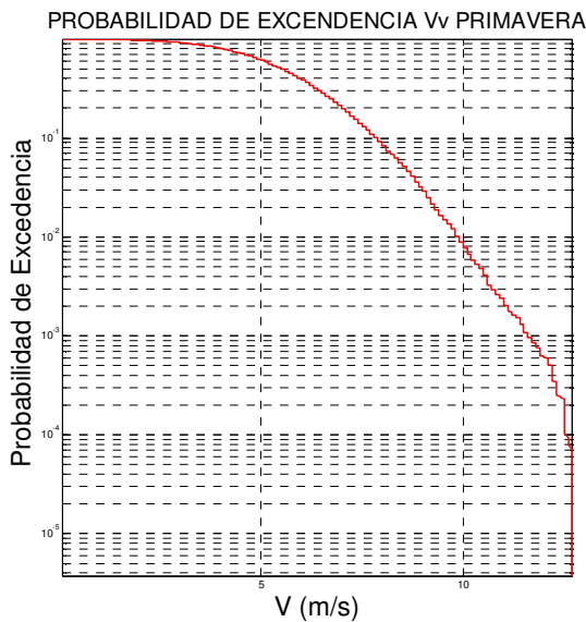
Figura A 125 Probabilidad de Excedencia Primavera
