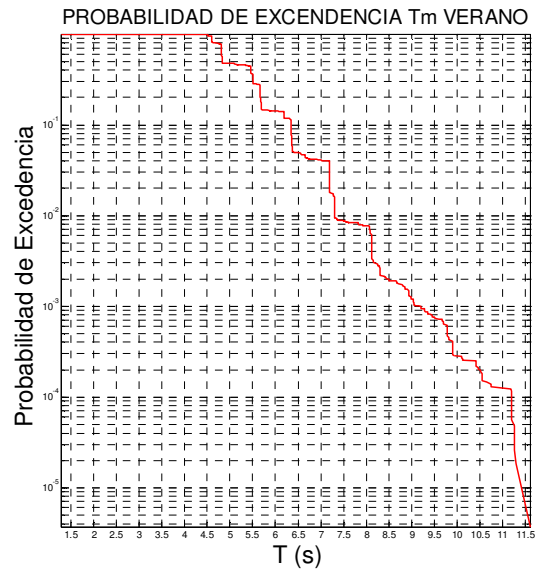
Figura A 116 Probabilidad de Excedencia Verano
