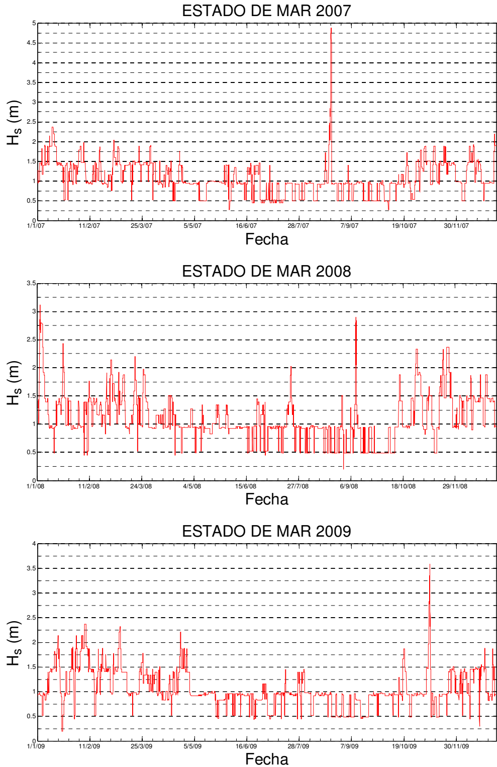
Figura A 55 Estados de mar 2007-2009
