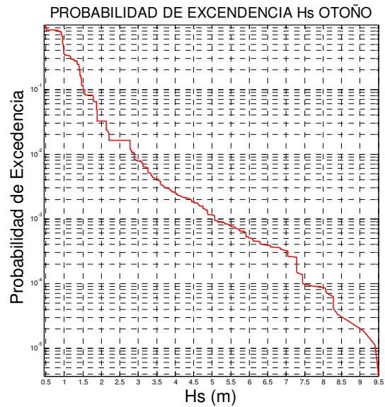
Figura A 7 Probabilidad de Excedencia Otoño
