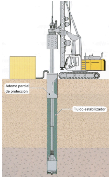
Fig. 43 Esquema de perforación con ademe metálico parcial (brocal) y fluido estabilizador. (Hudelmaier and Küfner 2009)
