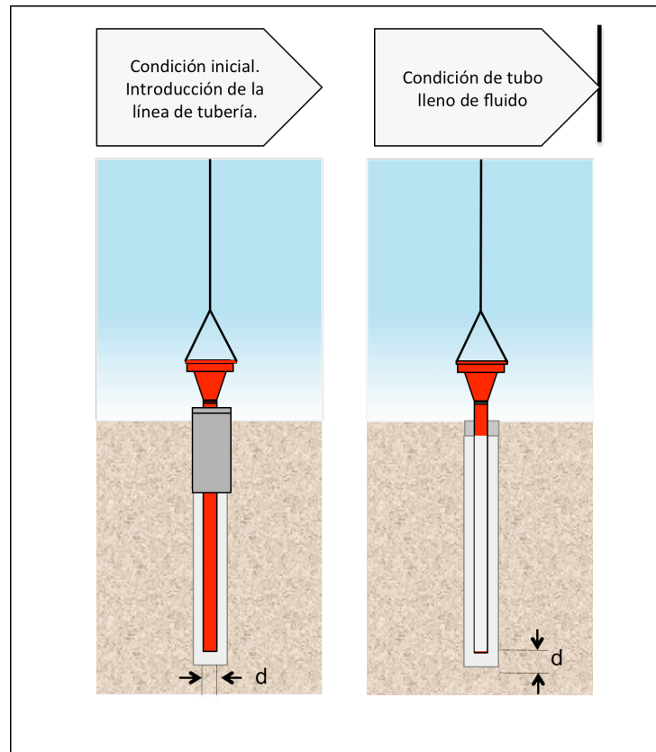
Fig. 70. Procedimiento de colado con tubería Tremie
