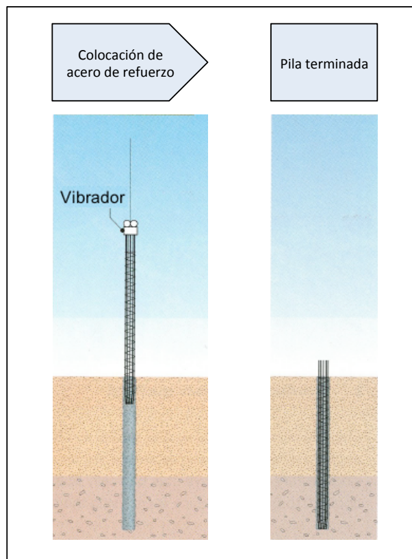
Fig. 54. Colocación de acero de refuerzo
