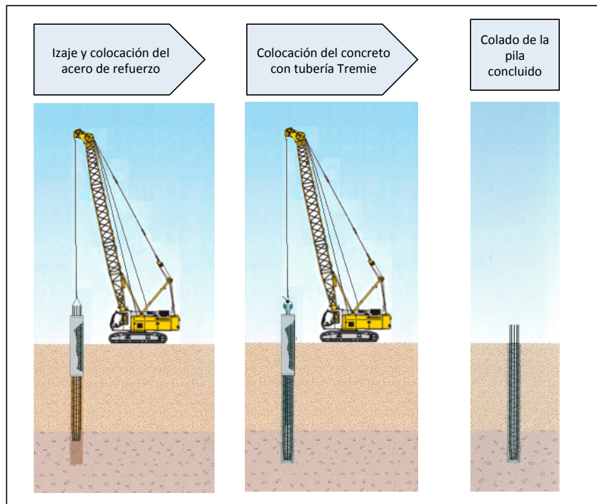
Fig. 42. Izaje de acero de refuerzo y colado de pila
