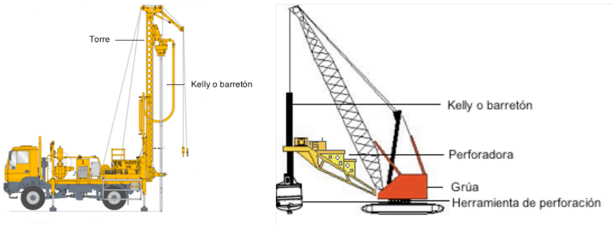
Fig. 4. Izquierda: Perforadora rotatoria con sistema de kelly montada sobre camión (Spiradrill); Derecha: Perforadora rotatoria con sistema de kelly montada en grúa
