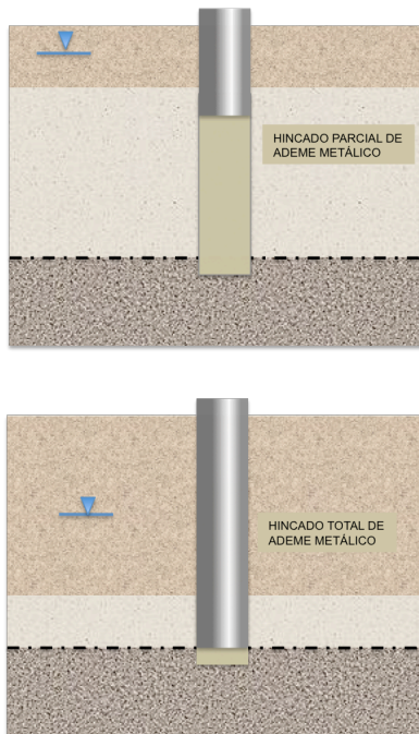
Fig. 24. Empleo de ademe metálico. Arriba: ademe parcial. Abajo: ademe en la totalidad de la longitud de la perforación
