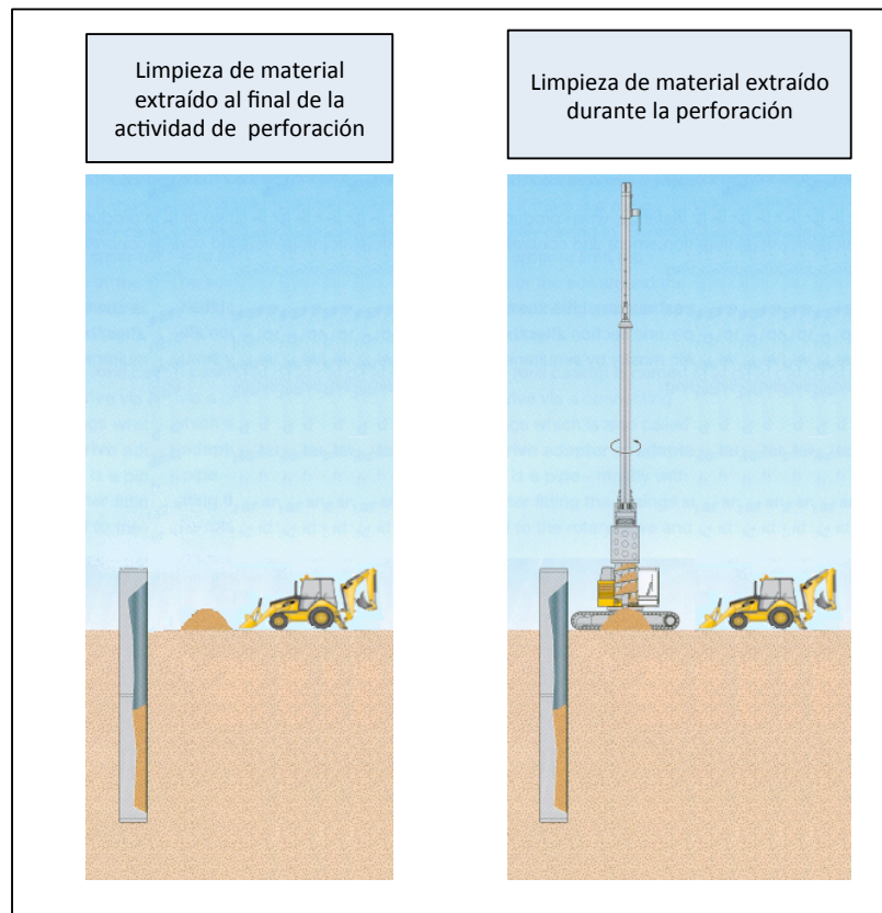
Fig. 29. Procedimiento constructivo. Retiro de material producto de excavación
