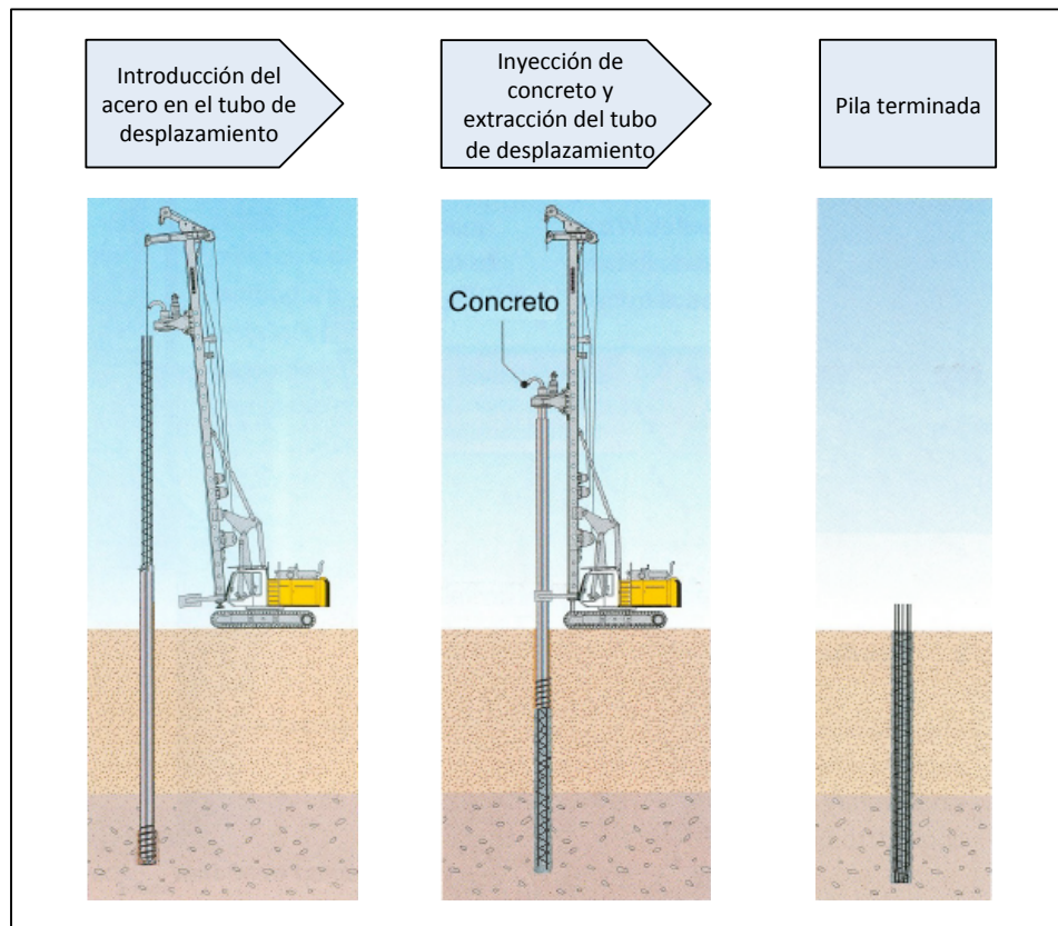
Fig. 60. Colocación de acero de refuerzo e inyección de concreto o mortero
