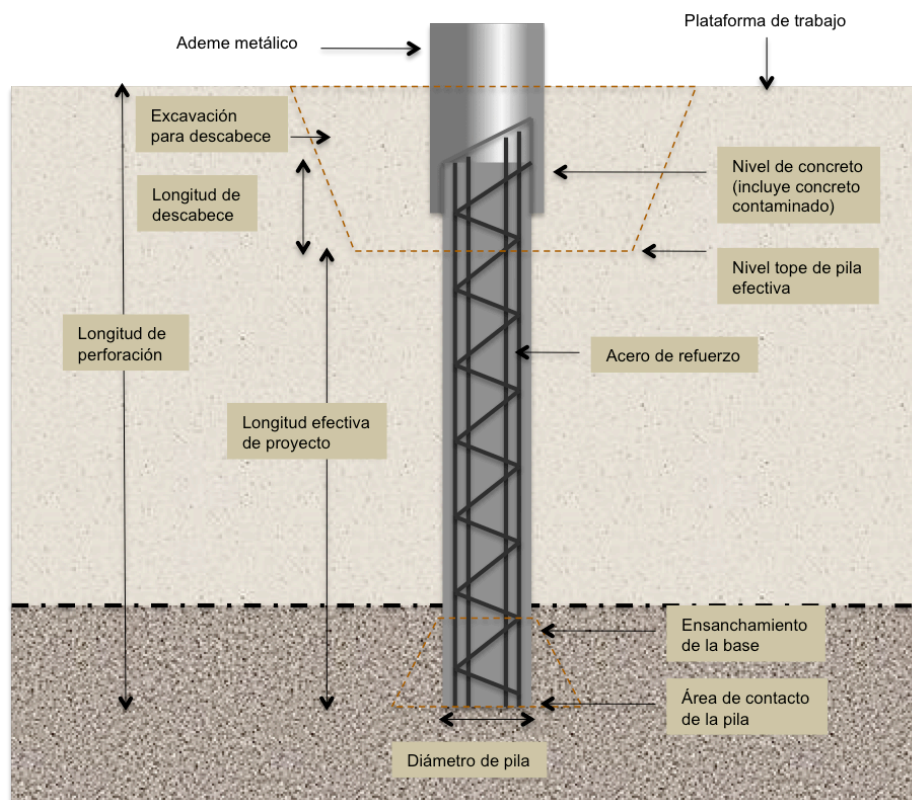
Fig. 23. Parte que componen a una pila de cimentación
