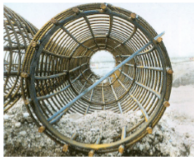
Fig. 66. Barra metálica auxiliar para vibrado del armado. (Hudelmaier and Küfner 2009)
