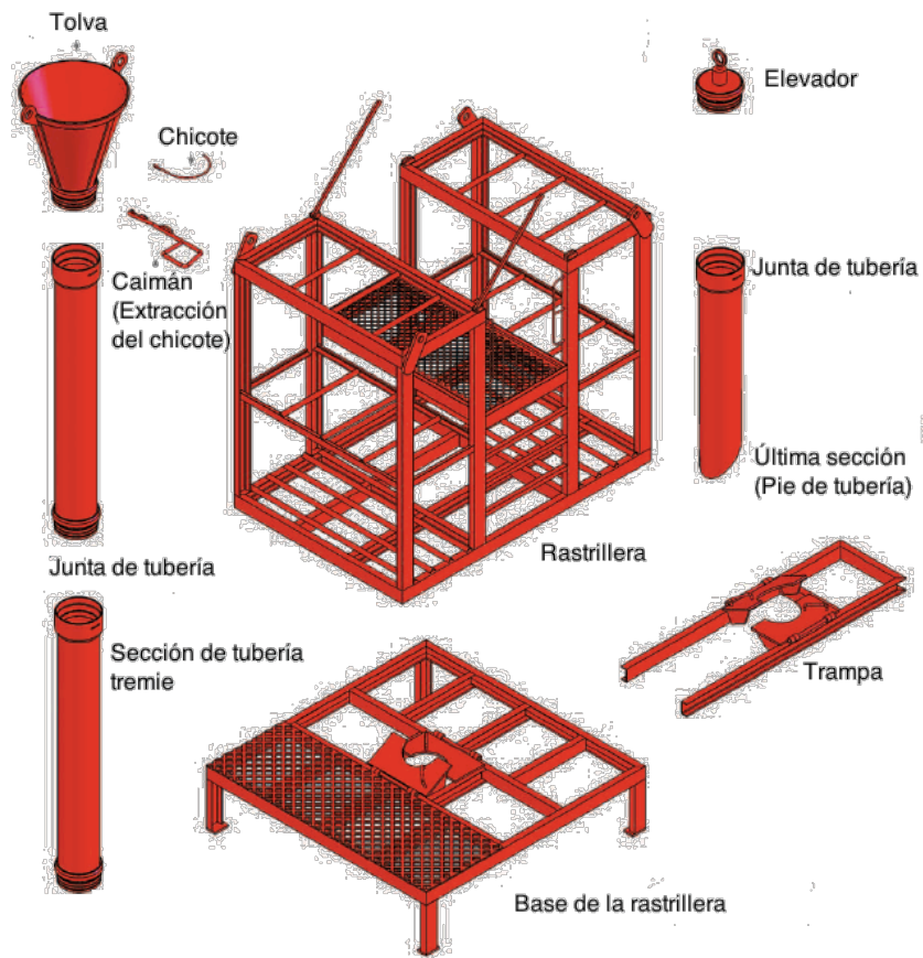
Fig. 69. Tubería Tremie (SPIT&T)
