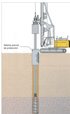
Fig. 40. Perforación con ademe metálico parcial (brocal)
