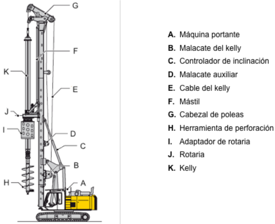
Fig. 3. Partes principales de perforadora rotatoria con sistema de kelly y máquina base propia (Hudelmaier and Küfner 2009)
