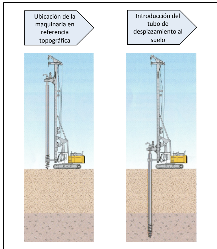
Fig. 59. Desplazamiento total de suelo
