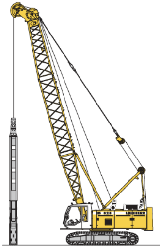
Fig. 10. Grúa de pluma rígida (LIEBHERR)
