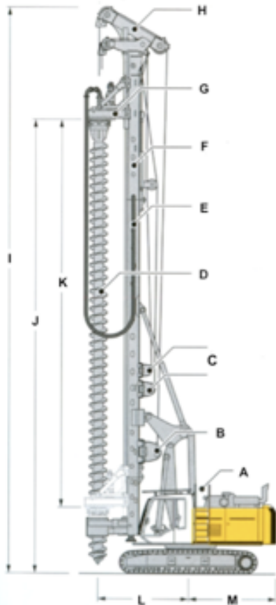
Fig. 6. Partes principales de perforadora rotatoria con hélice continua (Hudelmaier and Küfner 2009)
