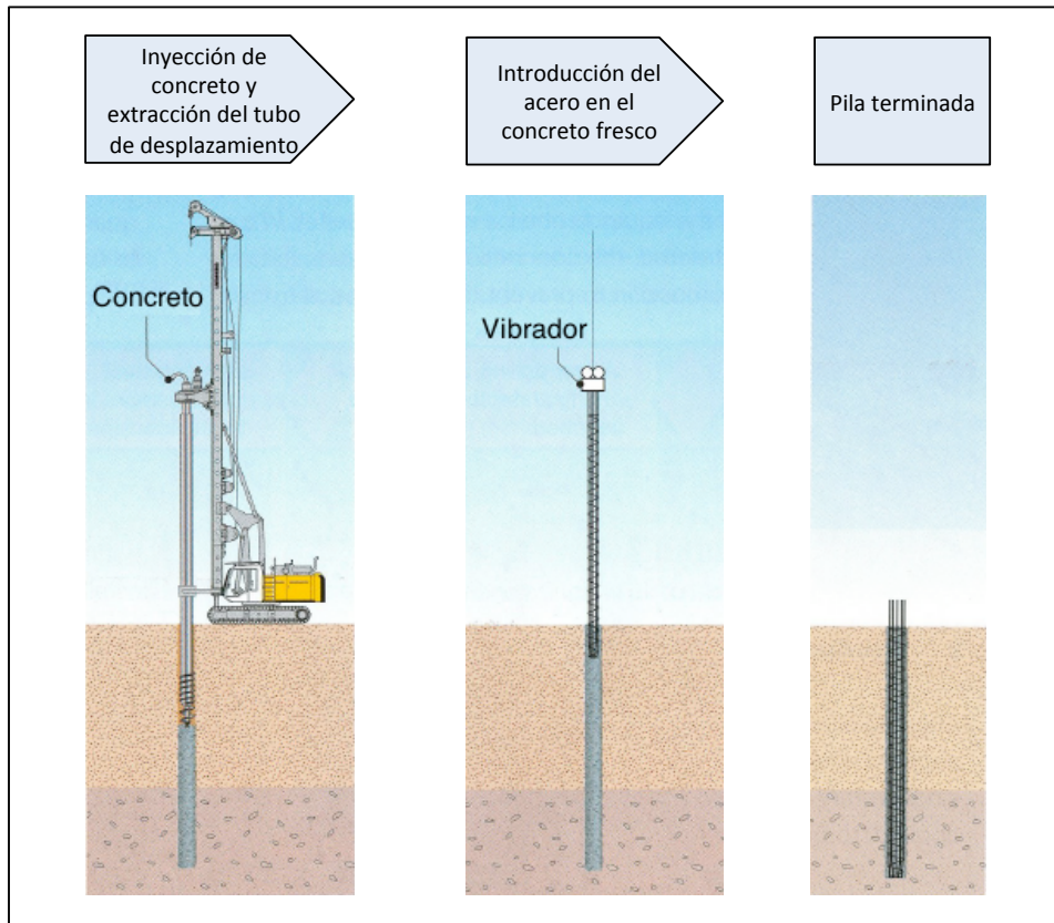
Fig. 61. Inyección de concreto o mortero y colocación de acero de refuerzo
