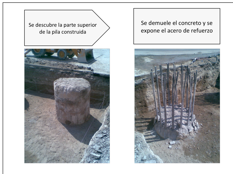
Fig. 75. Descabece de pila de cimentación
