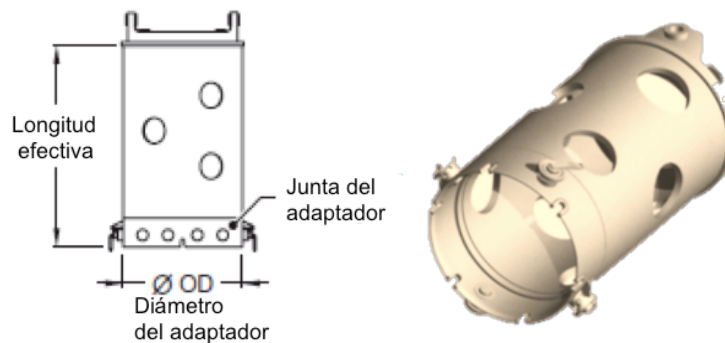
Fig. 14. Adaptador para ademes
