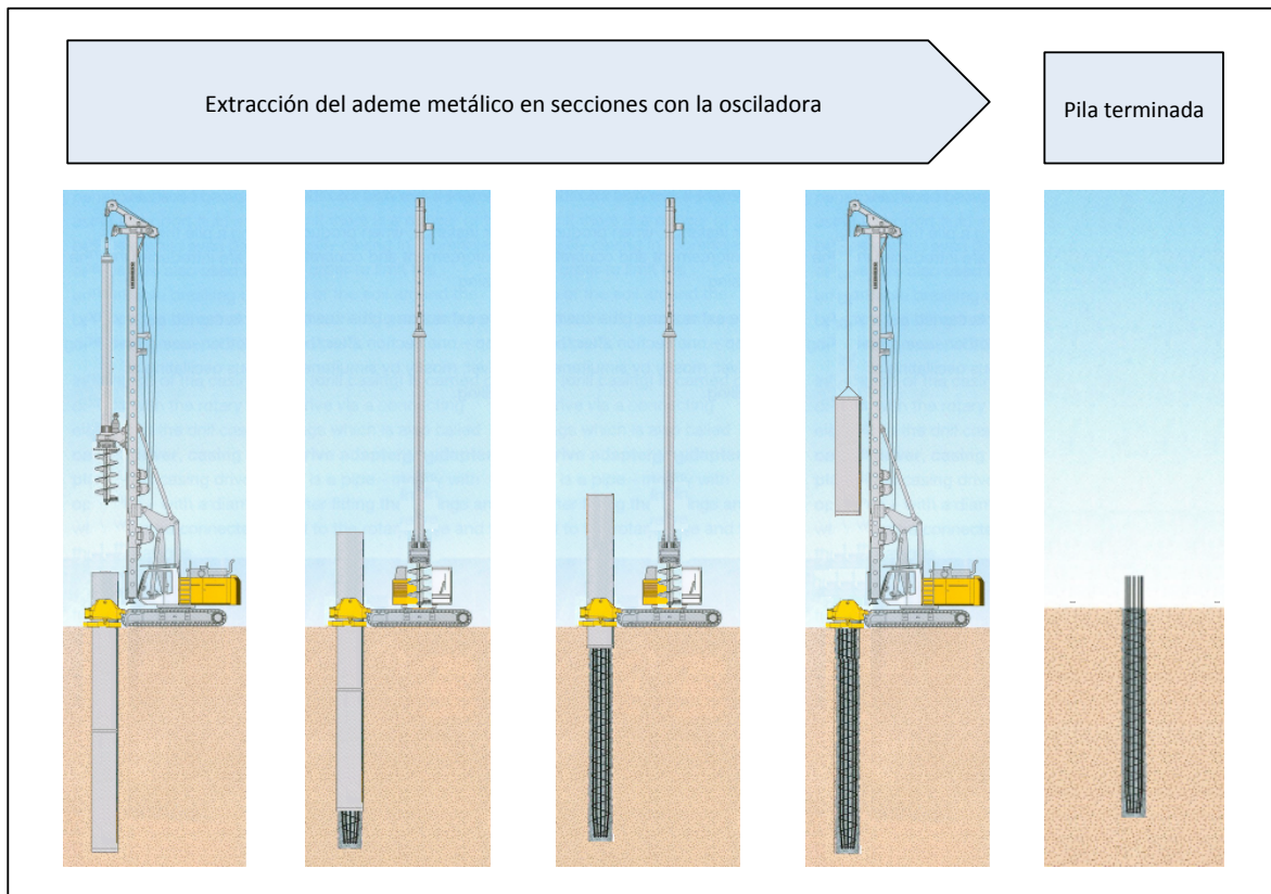
Fig. 36. Procedimiento constructivo. Extracción de secciones de ademe metálico con osciladora
