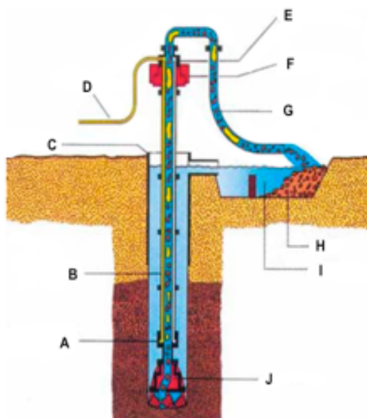
Fig. 7. Partes de perforadora de circulación inversa (Paniagua Z. and Paredes n.d.)
