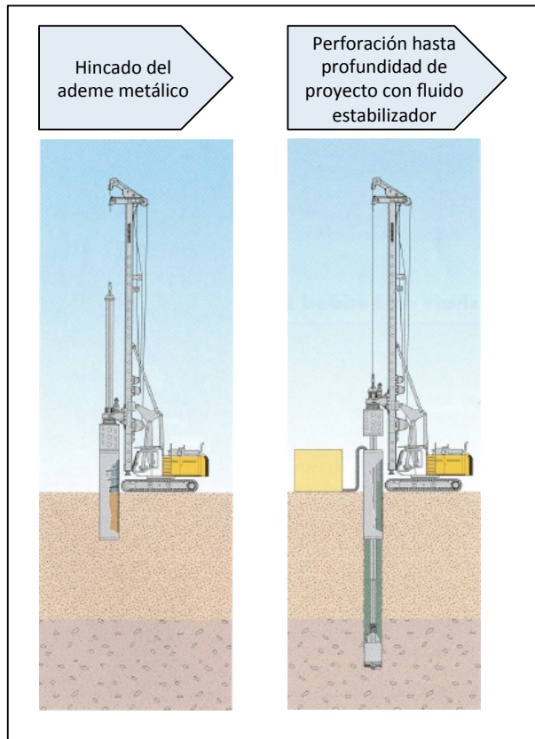
Fig. 44. Perforación con ademe metálico parcial y fluido estabilizador
