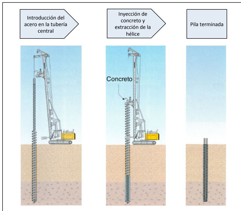
Fig. 56. Colocación del acero de refuerzo, extracción de hélice con material e inyección del concreto o mortero
