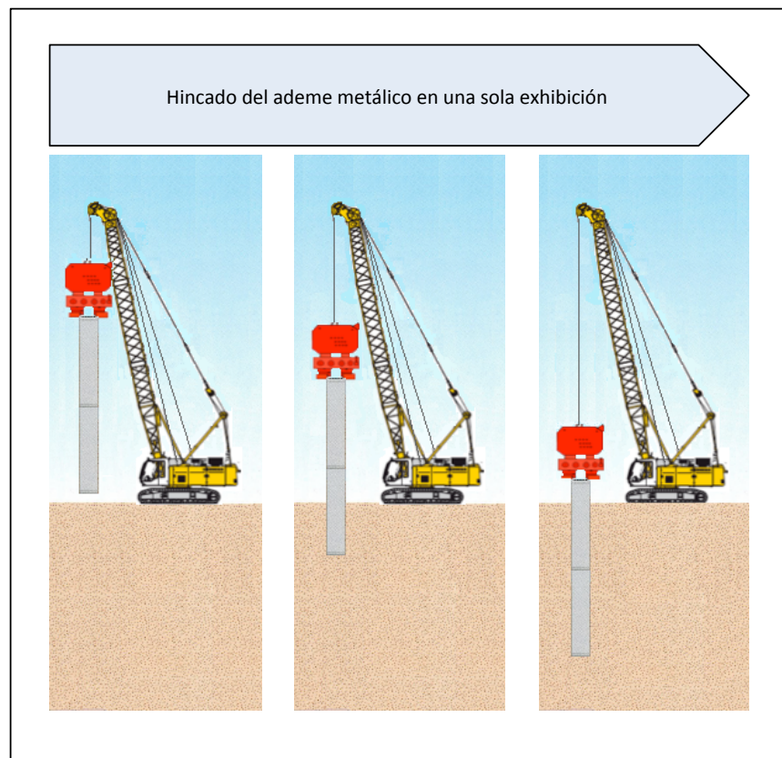
Fig. 39. Hincado de ademe metálico en una sola exhibición
