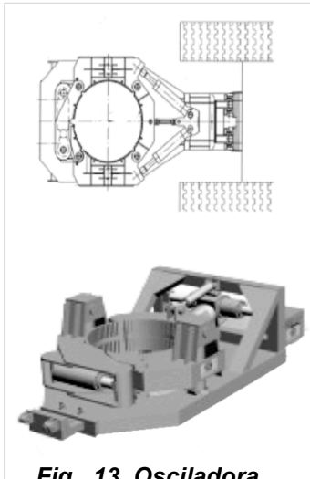
Fig. 13. Osciladora (LIEBHERR)
