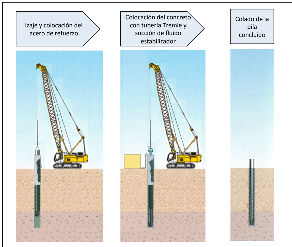
Fig. 46. Colcoación del acero de refuerzo y colado de pila
