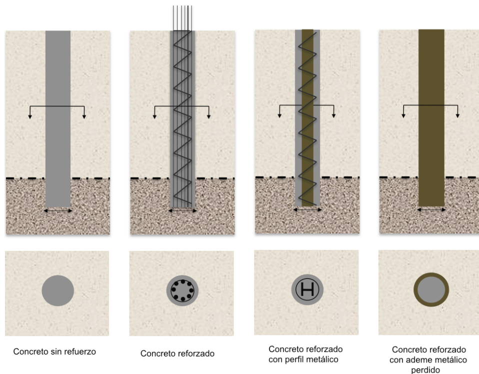
Fig. 63. Tipos de refuerzo en pilas de cimentación
