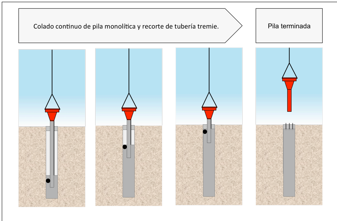
Fig. 72. Procedimiento de colado con tubería Tremie
