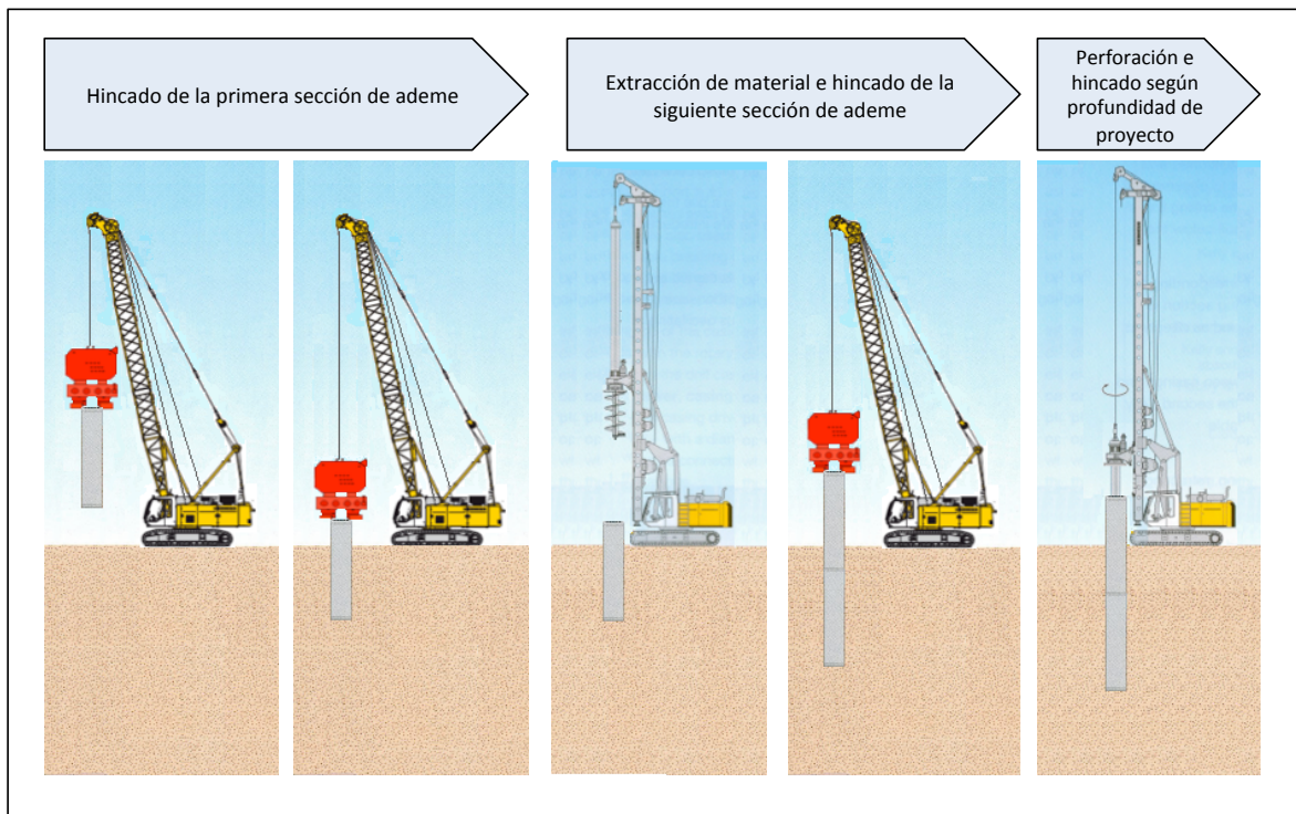
Fig. 38. Procedimiento constructivo. Hincado de ademe metálico en secciones
