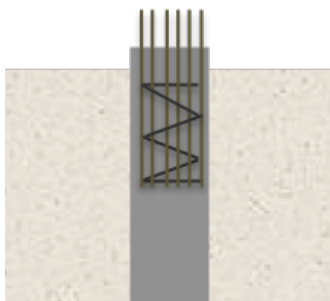
Fig. 64. Refuerzo de ligadura estructural
