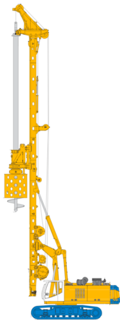
Fig. 2. Perforadora rotatoria con sistema de kelly (BAUER)
