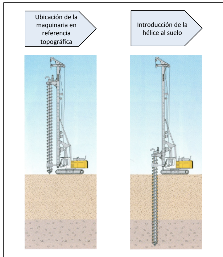
Fig. 55. Perforación desplazamiento de suelo
