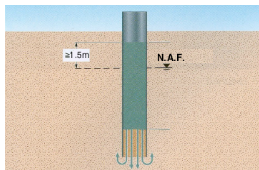
Fig. 45. Esquema de condición de nivel de fluido estabilizador
