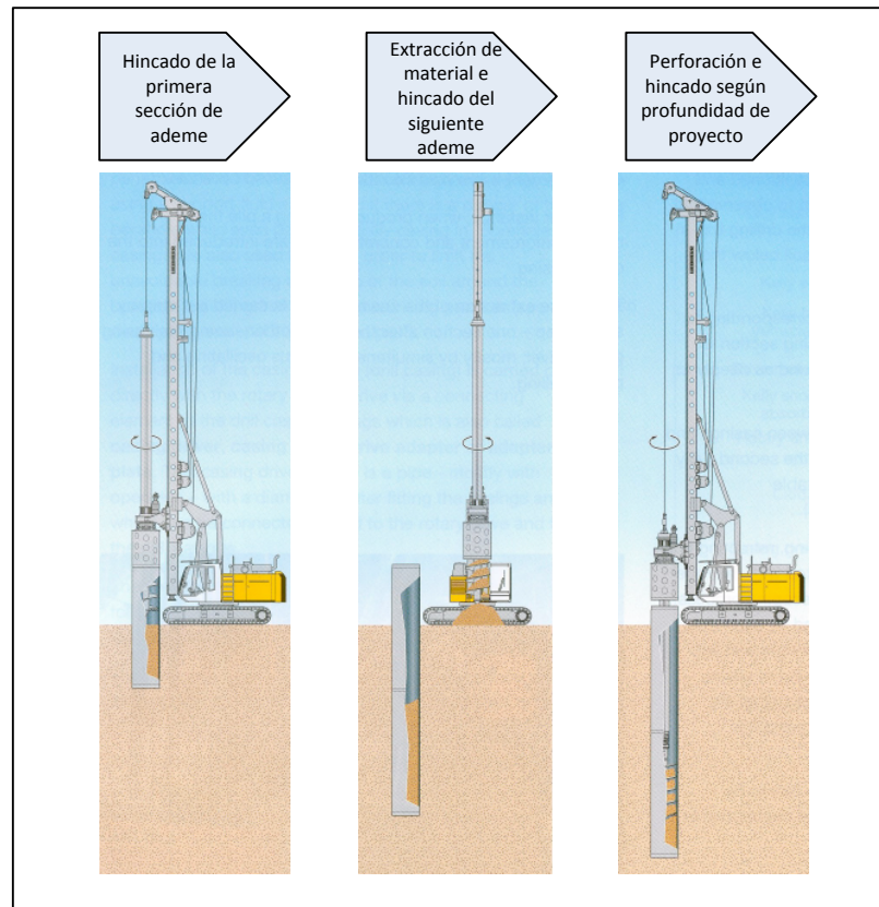
Fig. 27. Procedimiento constructivo, perforación e hincado de ademes
