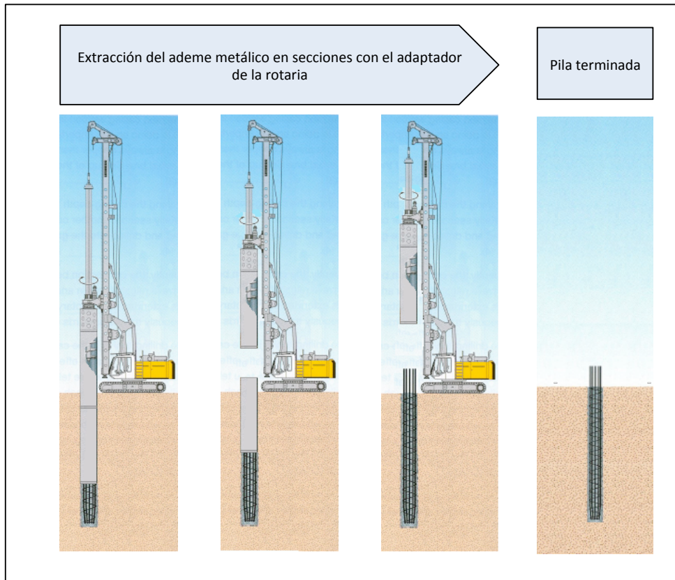
Fig. 31. Procedimiento constructivo. Extracción de ademes metálicos
