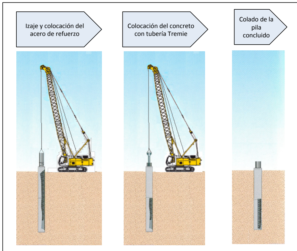
Fig. 30. Procedimiento constructivo. Izaje y colado de pila
