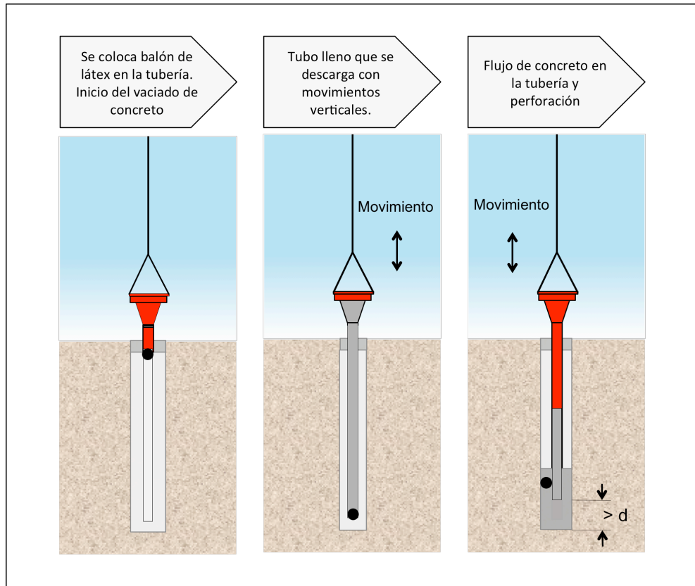
Fig. 71. Procedimiento de colado con tubería Tremie
