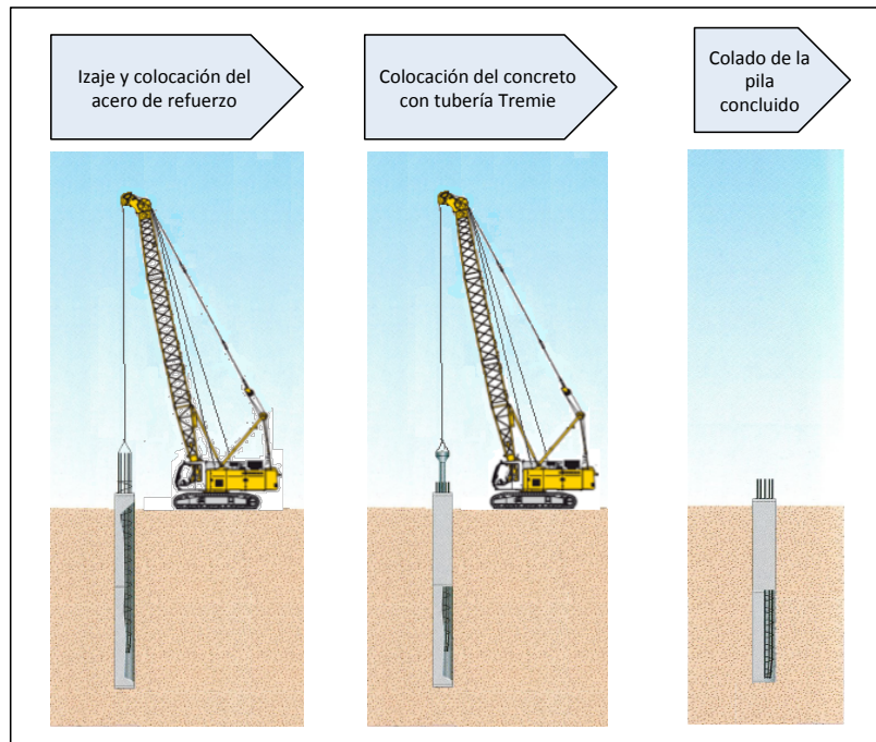
Fig. 35. Procedimiento constructivo. Izaje de acero de refuerzo y colado de pila
