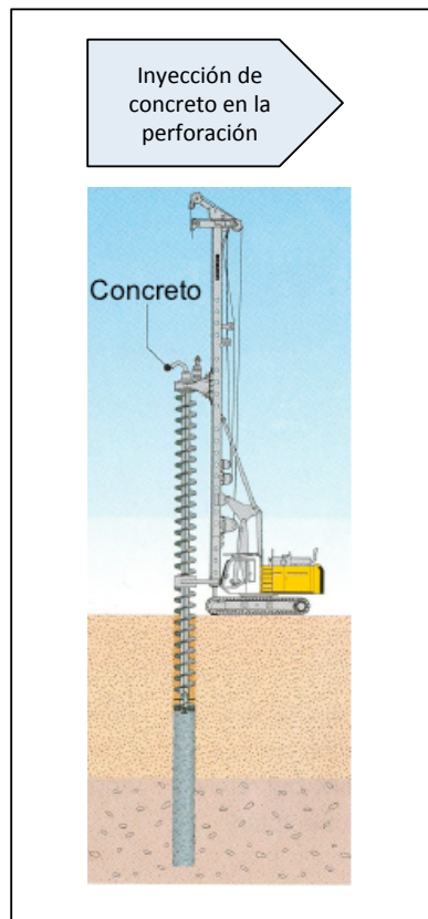
Fig. 53. Extracción e inyección de concreto o mortero
