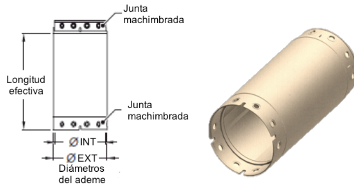
Fig. 21. Ademe metálico
