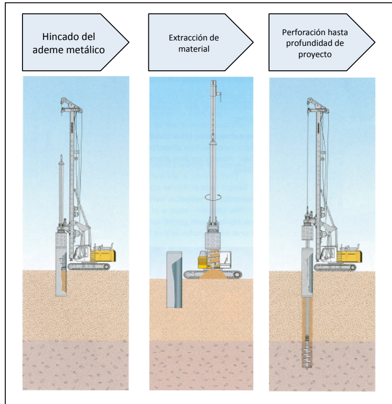
Fig. 41. Procedimiento constructivo perforación con ademe metálico parcial sin fluido estabilizador
