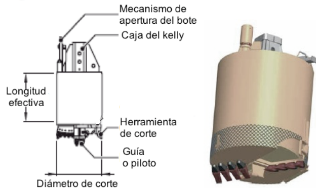
Fig. 17. Bote de perforación
