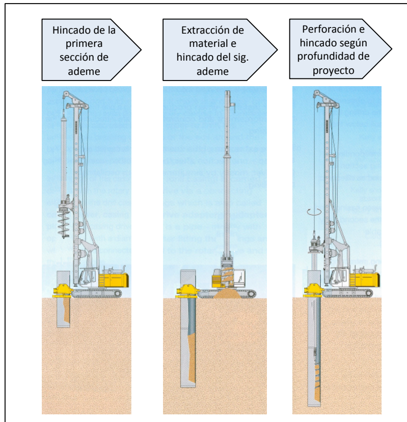
Fig. 34. Procedimiento constructivo, extracción de material e hincado de ademes con osciladora
