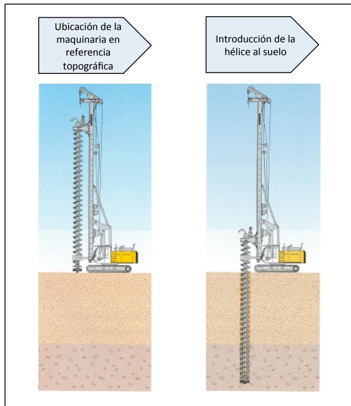
Fig. 52. Perforación con hélice continua
