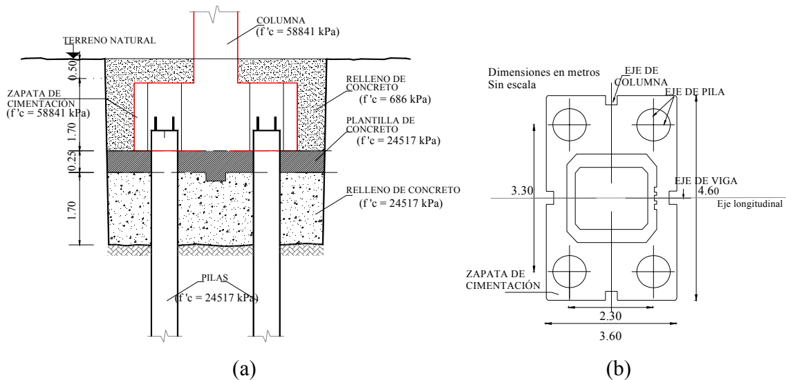
Figura 2.3 Esquema de la cimentación (a) elevación (b) planta
