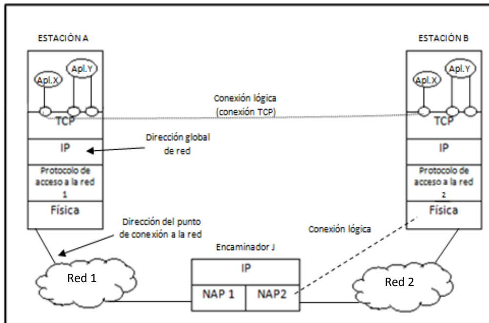
Figura 1. 8 Funcionamiento de TCP/IP (2.9).
