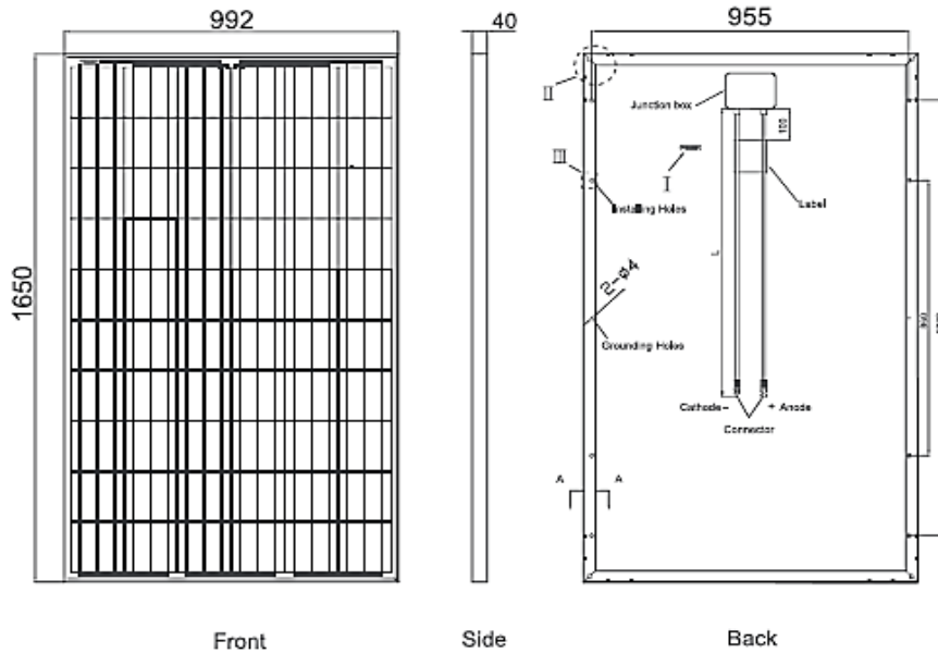
Figura 46. Dimensiones del panel del módulo JKM50P.
