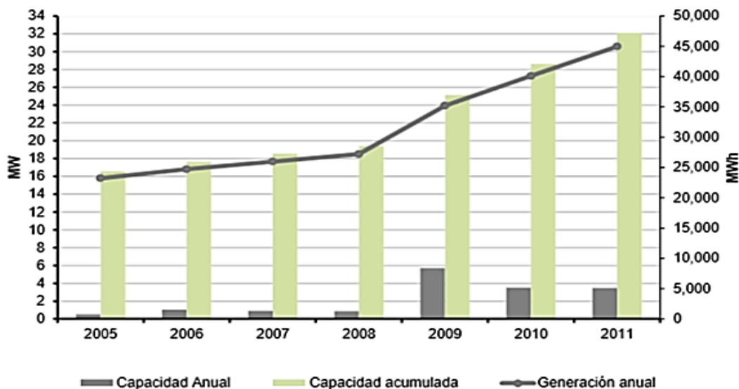
Figura 32: Evolución de la capacidad instalada y generación de electricidad con sistemas FV en México.
