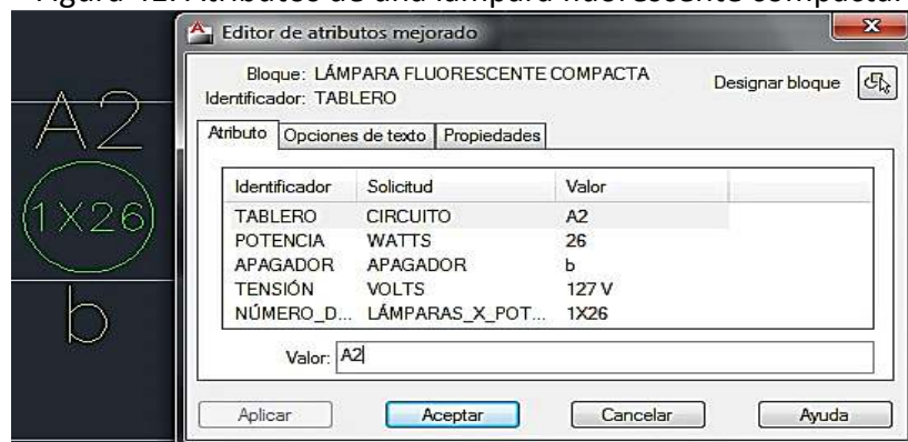
Figura 41. Atributos de una lámpara fluorescente compacta.
