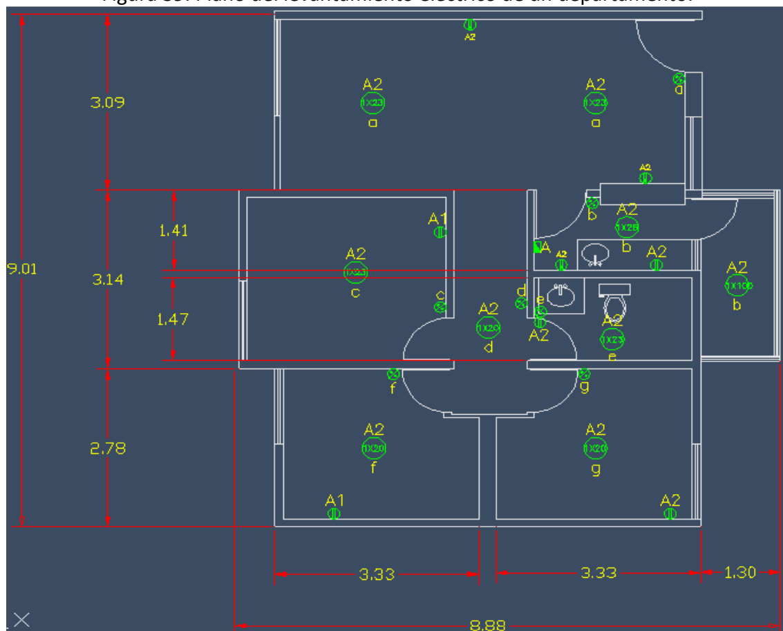
Figura 39. Plano del levantamiento eléctrico de un departamento.
