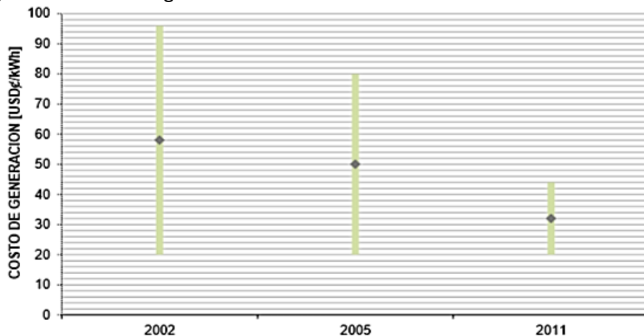
Figura 31: Costos de generación con sistemas FV a nivel mundial 2002 – 2011.
