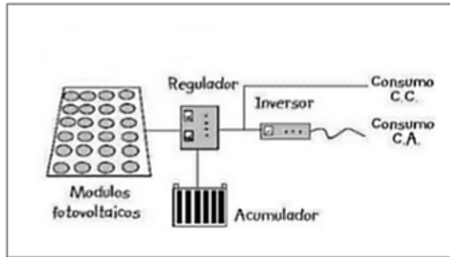
Figura 27: Sistema FV aislado.
