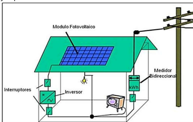
Figura 28: Ejemplo de sistema FV interconectado a la red eléctrica en una vivienda.
