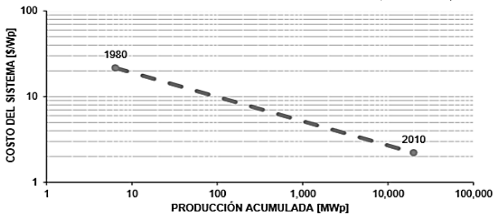
Figura 30: Desarrollo del costo de los módulos FV, 1980 – 2010 (curva de aprendizaje).
