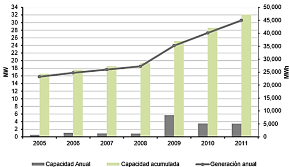
Figura 23. Evolución de la capacidad instalada y generación de electricidad con sistemas FV en México.
