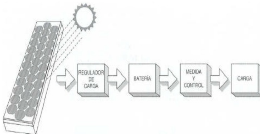
Figura 3.6. Diagrama de una instalación solar fotovoltaica. 1
