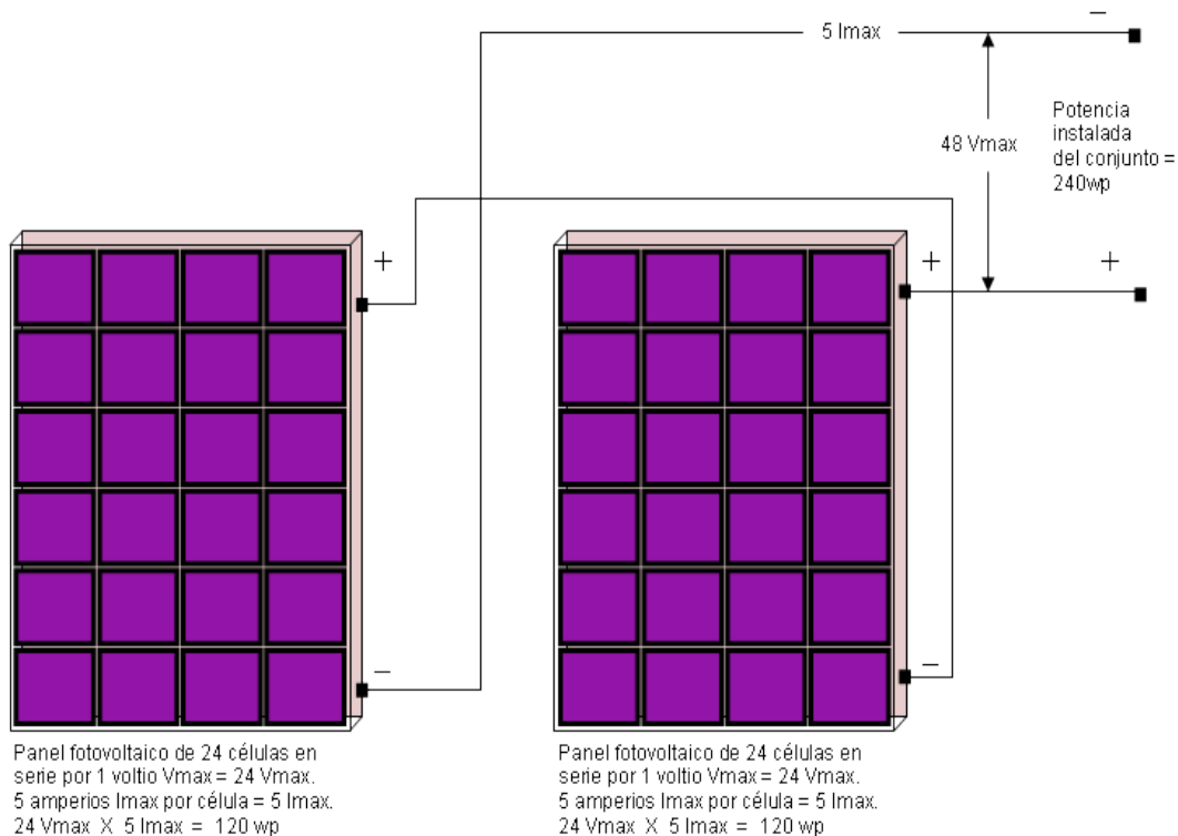
Figura 1.11. Ejemplo de conexión de paneles en serie. 1
