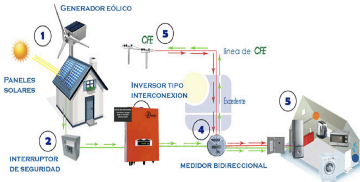
Figura 1.3. Sistema híbrido con entrega de excedente a la red de CFE. 1
