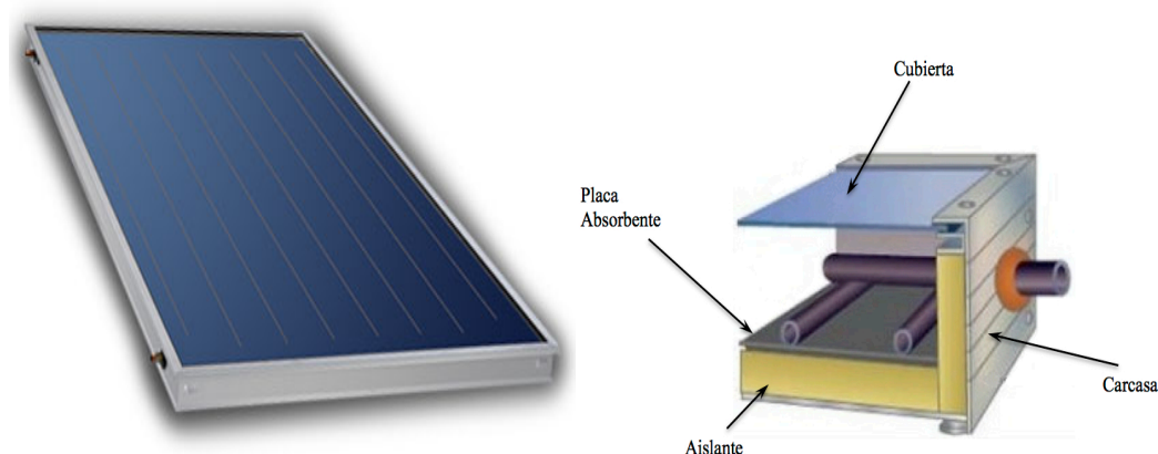
Figura 2.2. Colector solar plano y sus componentes. 1
