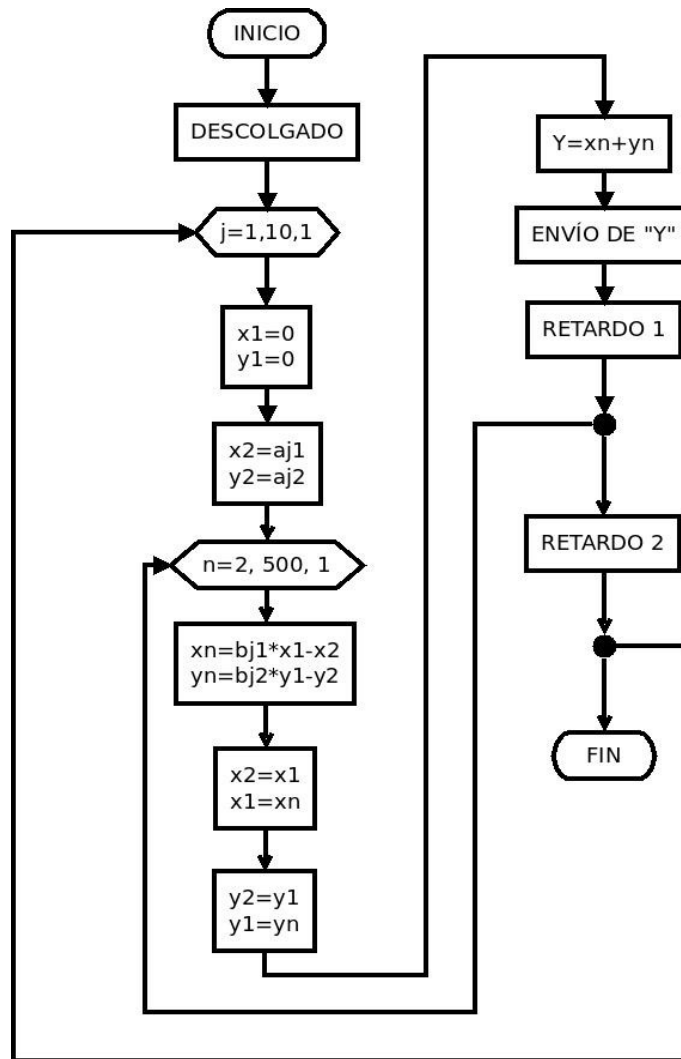
Figura 4.12: Diagrama de flujo de la generación de tonos DTMF.
