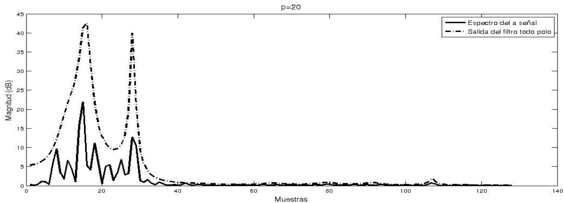
Figura 2.16: Espectro de la señal y salida del filtro todo polo p=20 .
