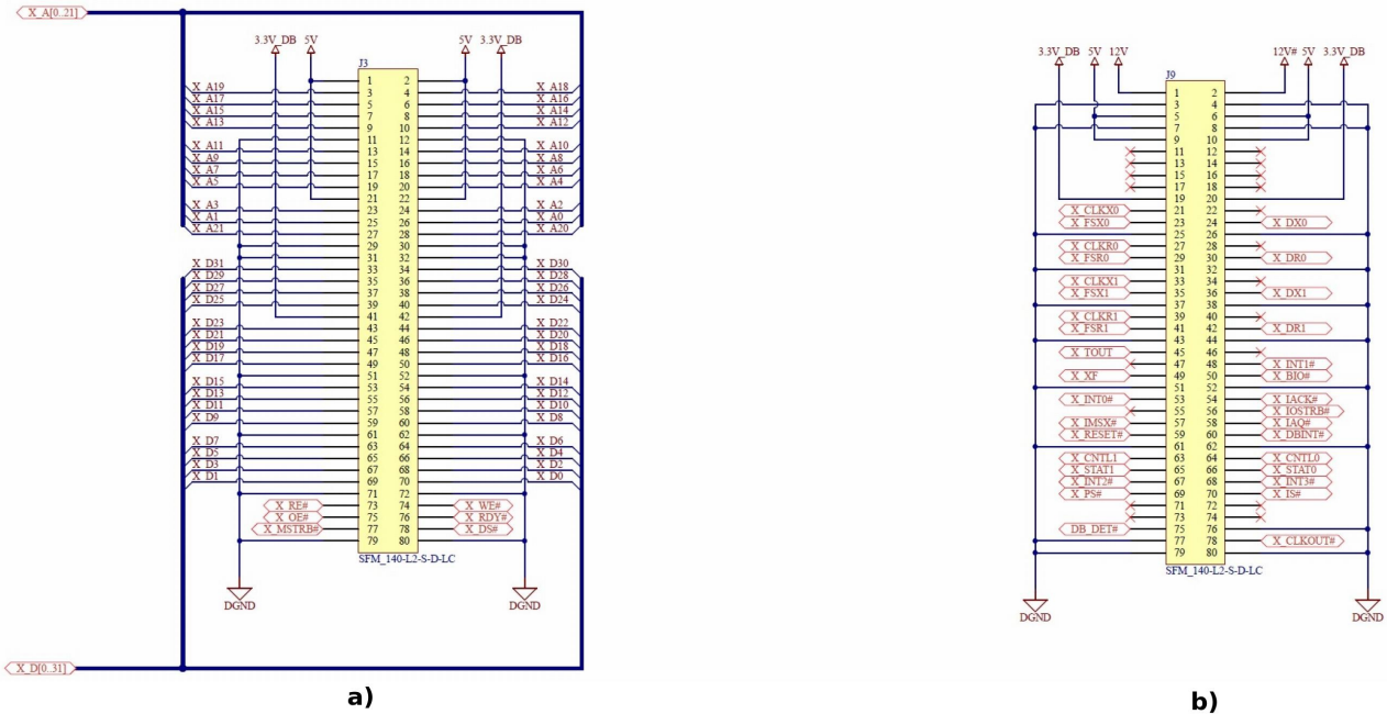
Figura 4.9: Interfaz de expansión de memoria y periféricos.
