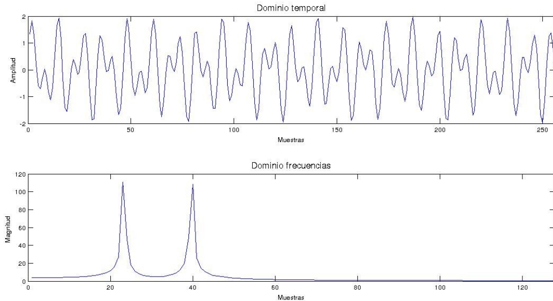
Figura 3.10: Ejemplo de una señal DTMF en el dominio temporal y frecuencial.
