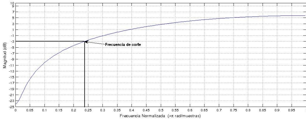
Figura 2.8: Filtro de preénfasis.
