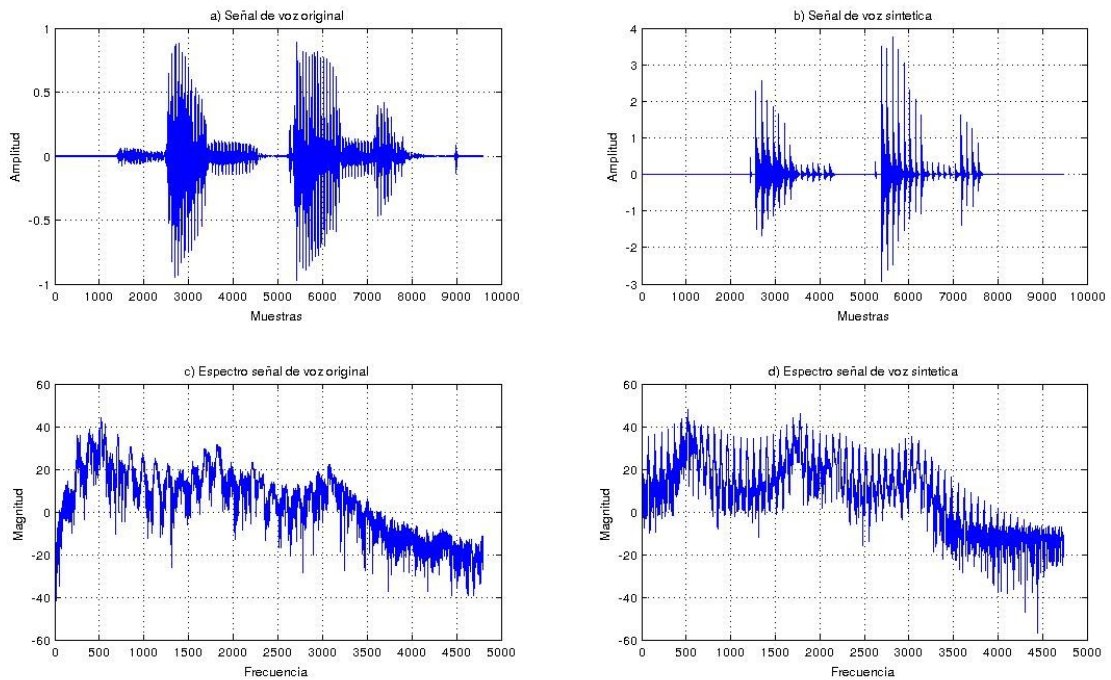
Figura 5.5: Señal a)Original, b)Sintética, c)Espectro original, d)Espectro sintética, N=128 , p=10 .
