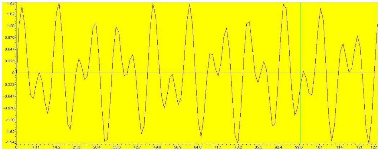
Figura 5.8: Tono DTMF correspondiente al número 1.
