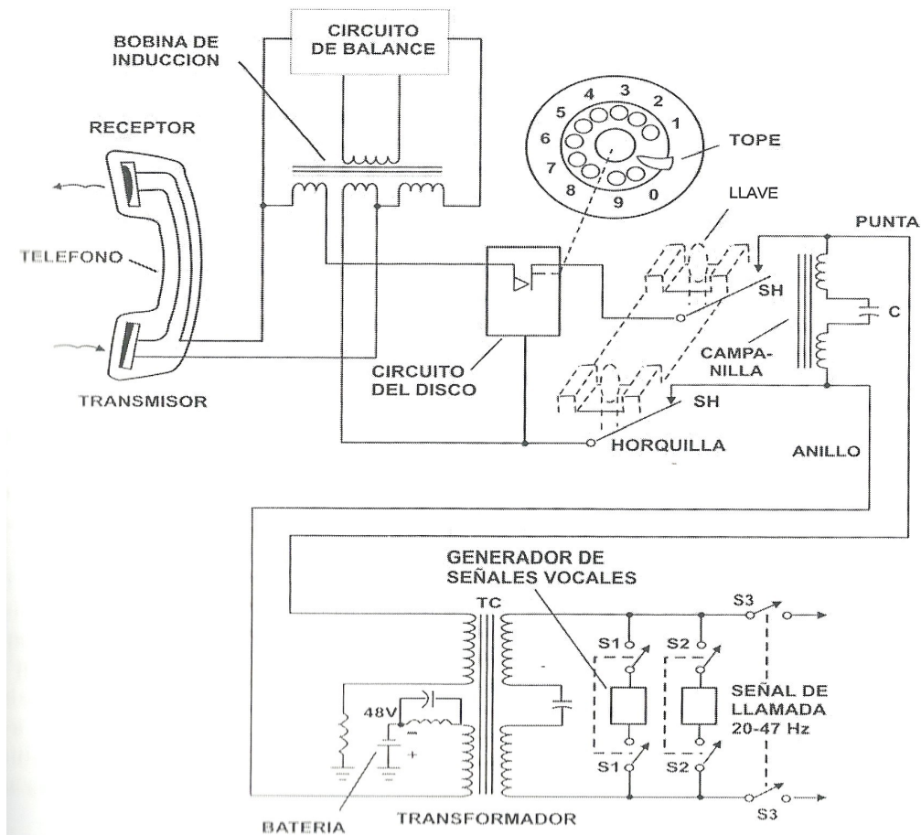
Figura 3.1: Circuito simplificado del aparato telefónico (analógico) [3].
