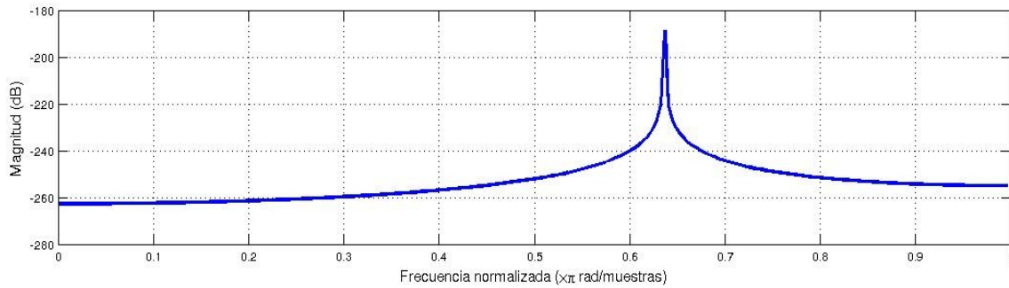
Figura 3.13: Respuesta en frecuencia del filtro IIR.
