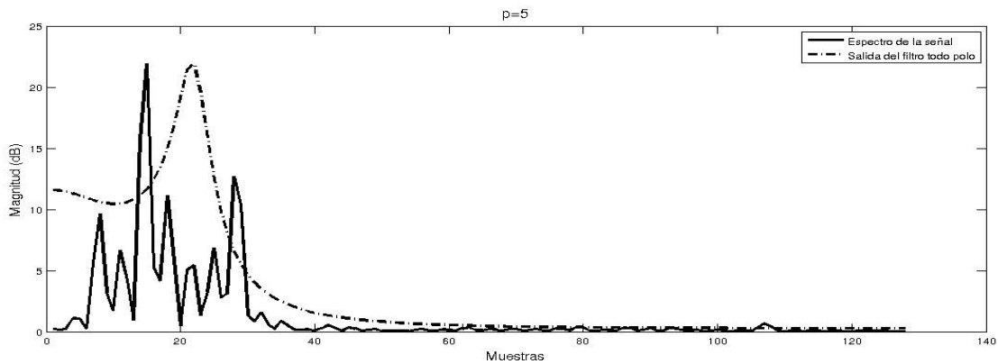
Figura 2.14: Espectro de la señal y salida del filtro todo polo p=5 .
