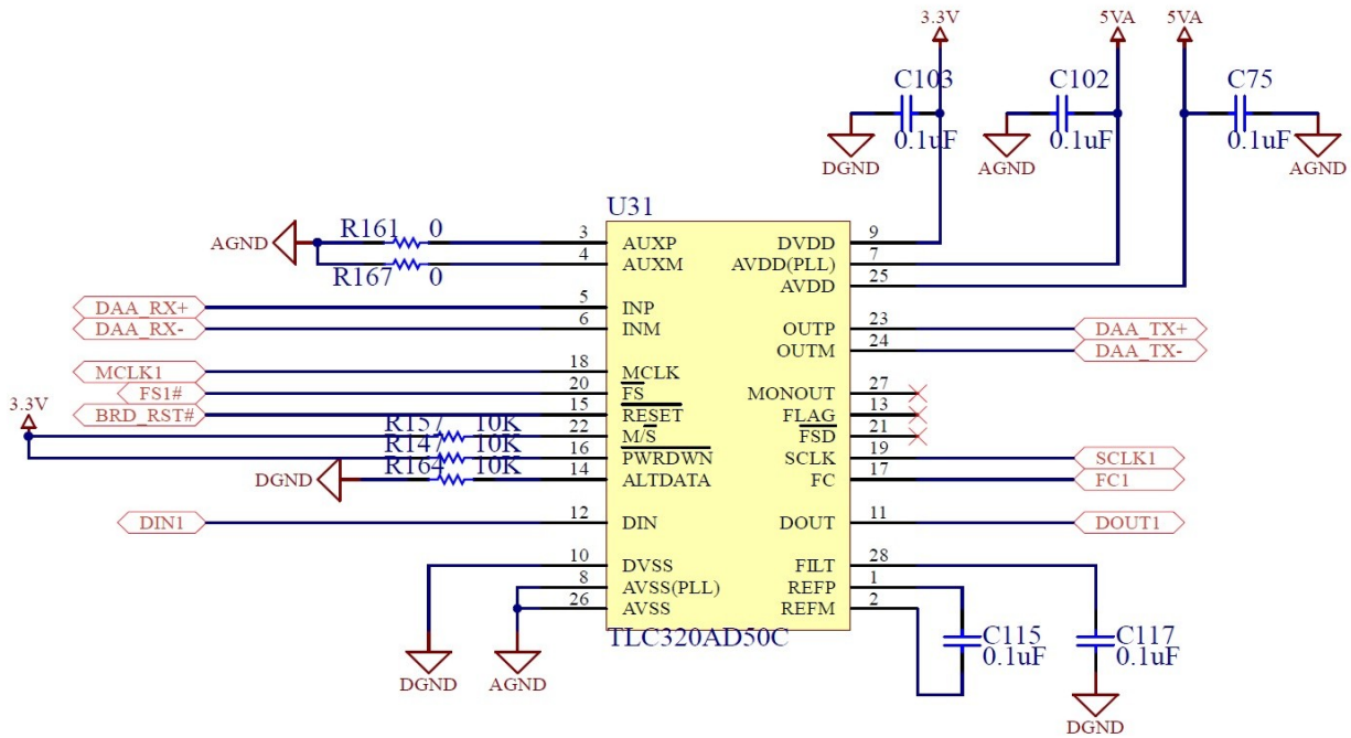
Figura 4.6: Códec para la interfaz DAA.
