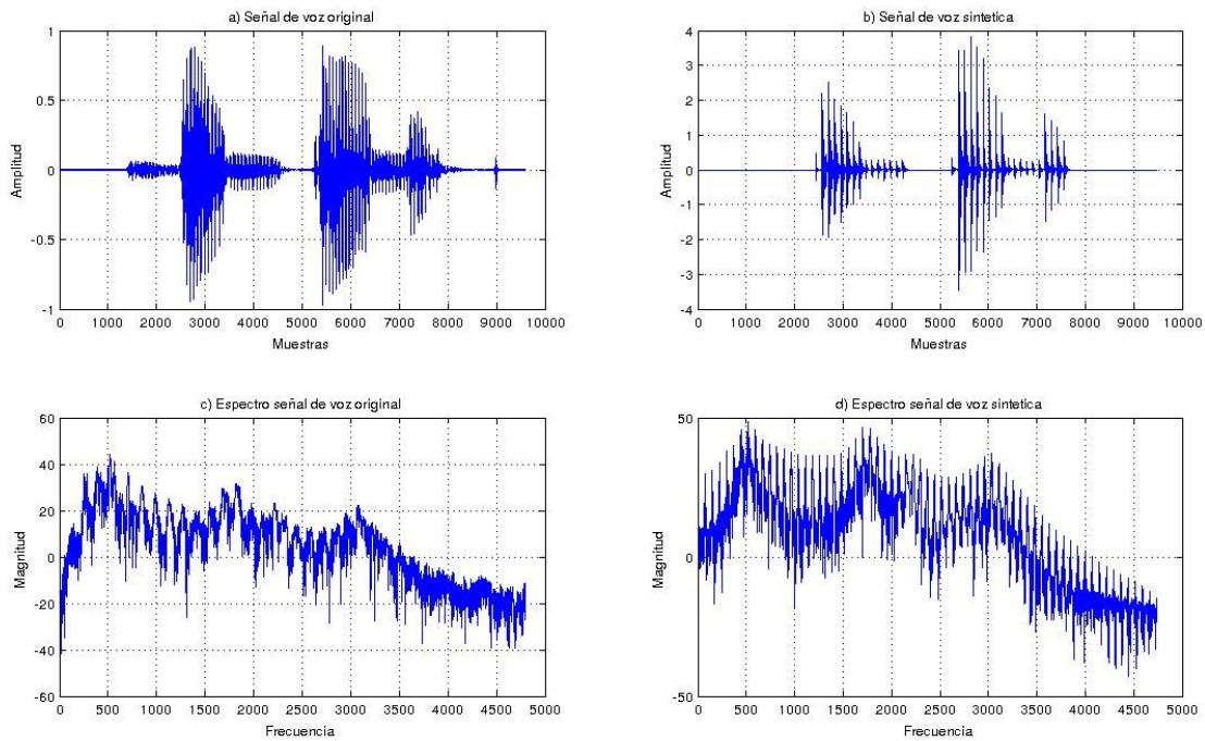
Figura 5.6: Señal a)Original, b)Sintética, c)Espectro original, d)Espectro sintética, N=128 , p=20 .
