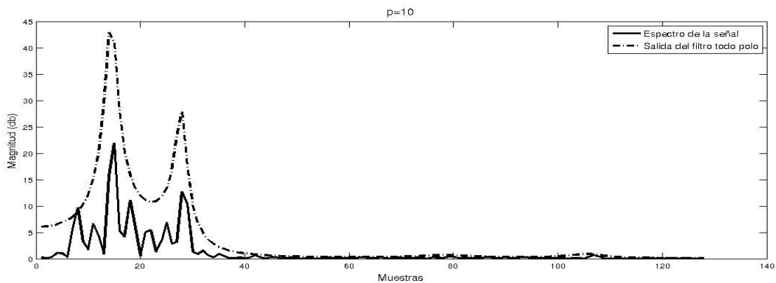
Figura 2.15: Espectro de la señal y salida del filtro todo polo p=10 .
