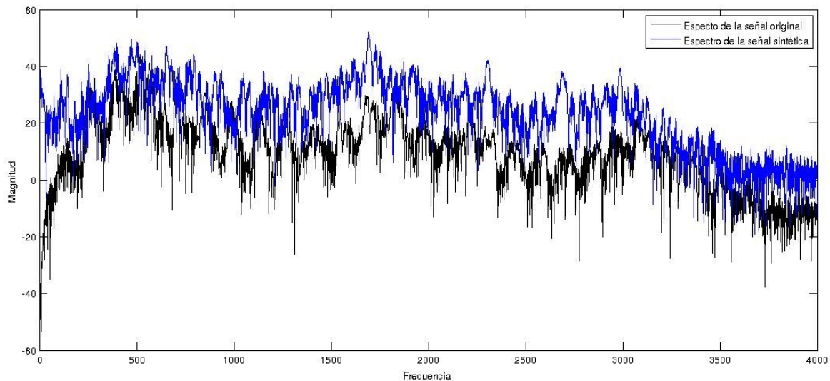
Figura 2.19: Espectro de una señal de voz original (negra) y sintética (azul).
