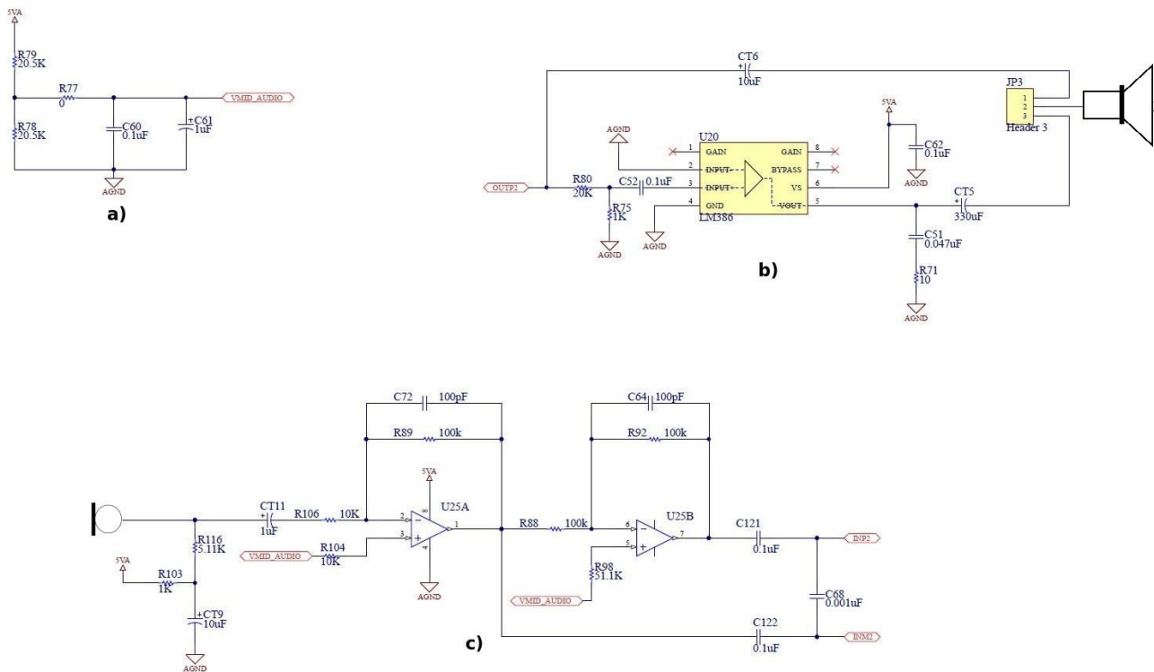
Figura 4.7: Circuito de micrófono y bocina.
