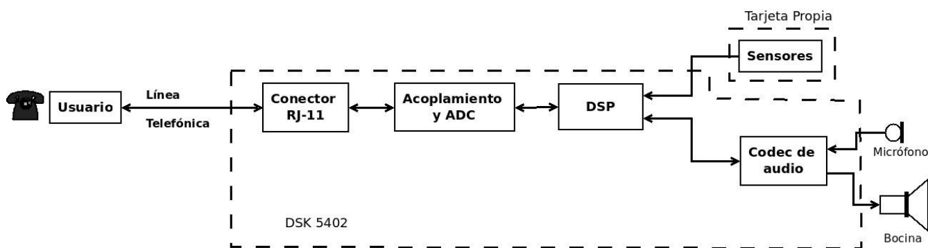
Figura 4.1: Diagrama de bloques del sistema.
