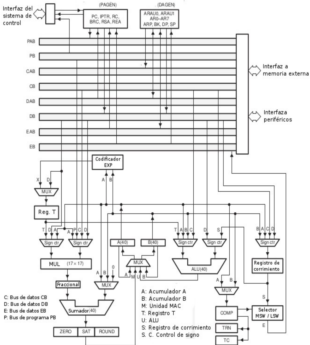
Figura 4.8: Diagrama a bloques del TMS320C5402 [17].
