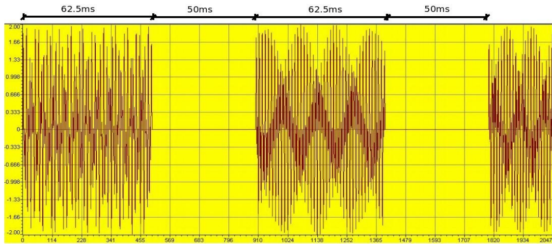
Figura 5.10: Ejemplo de varios tonos DTMF, correspondiente a los dígitos 1, 2 y 3.
