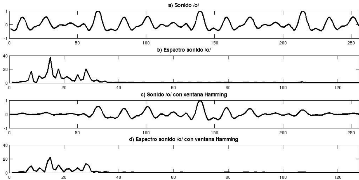
Figura 2.6: Segmento de voz aplicándole una ventana Hamming con N=256 .
