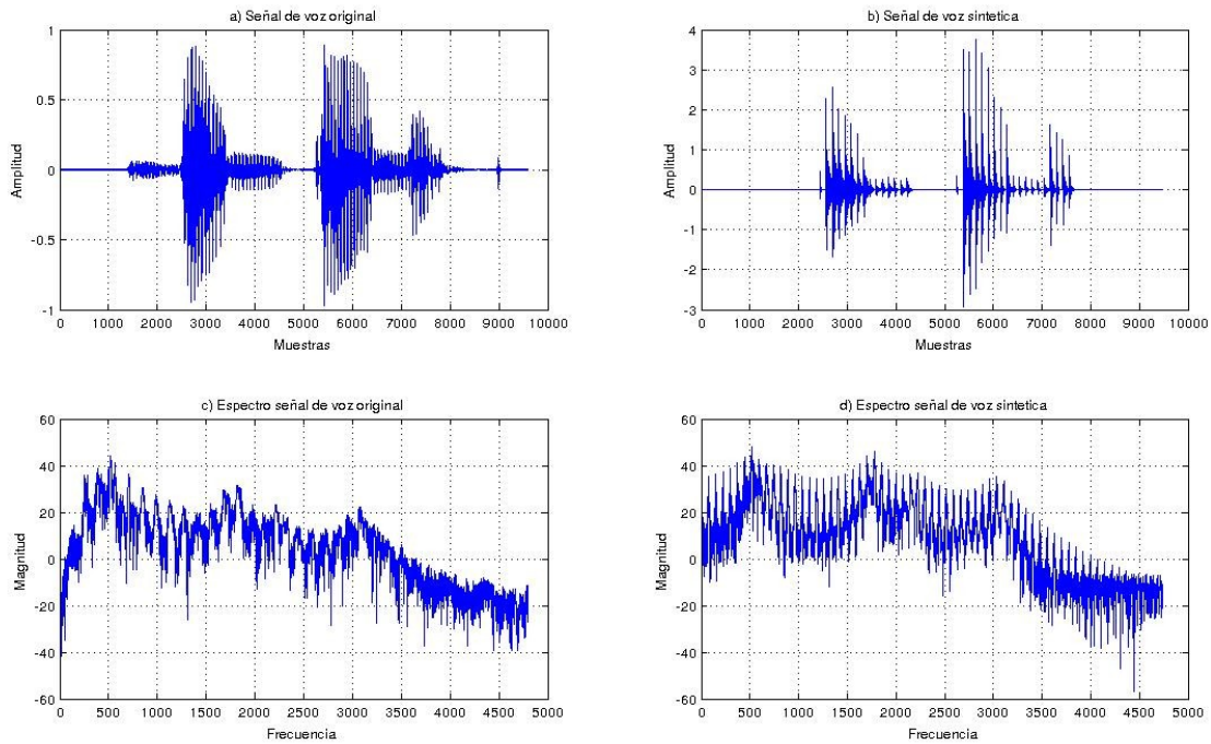
Figura 5.3: Señal a)Original, b)Sintética, c)Espectro original, d)Espectro sintética, N=128 , p=10 .
