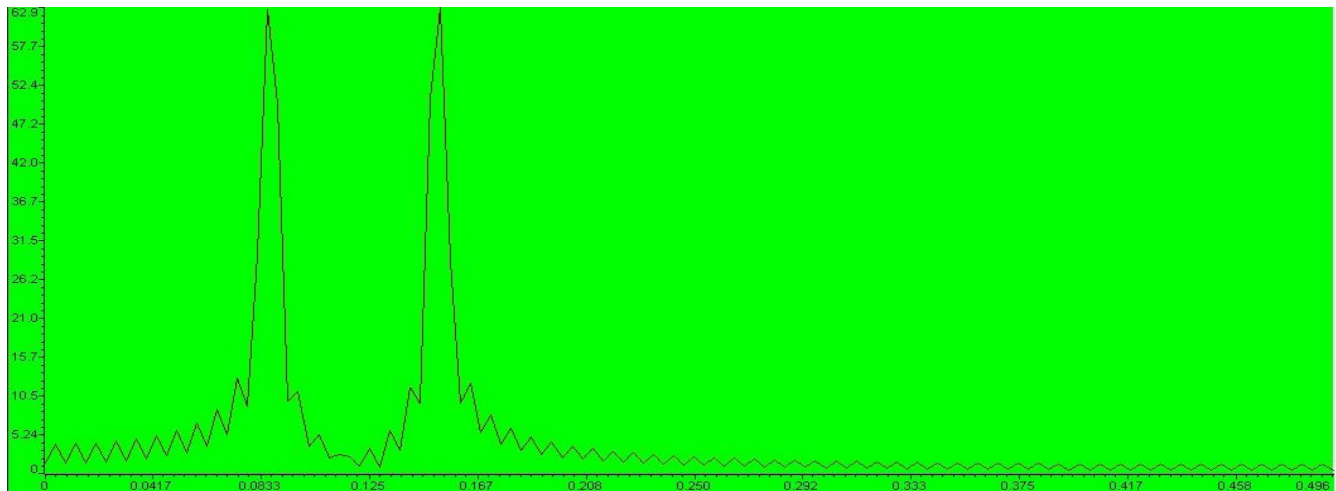
Figura 5.9: Espectro de tono DTMF correspondiente al número 1.
