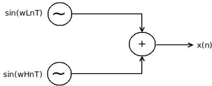
Figura 3.11: Diagrama de bloques de un generador DTMF
