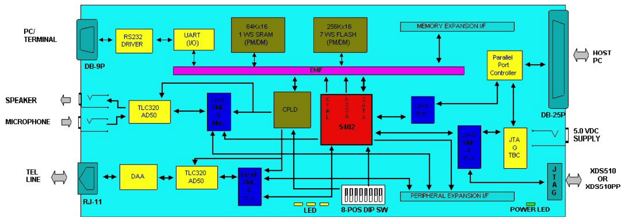
Figura 4.4: Sistema de desarrollo TMS320C5402 DSK [8].
