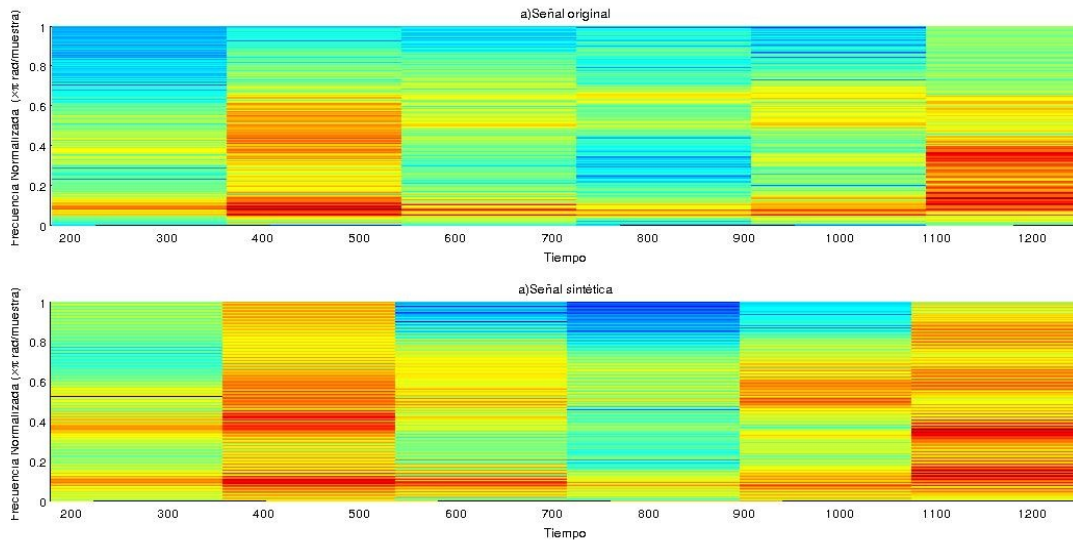
Figura 5.7: Espectrograma de la señal de voz "principal" a)Original, b)Sintética, N=128 , p=10 .
