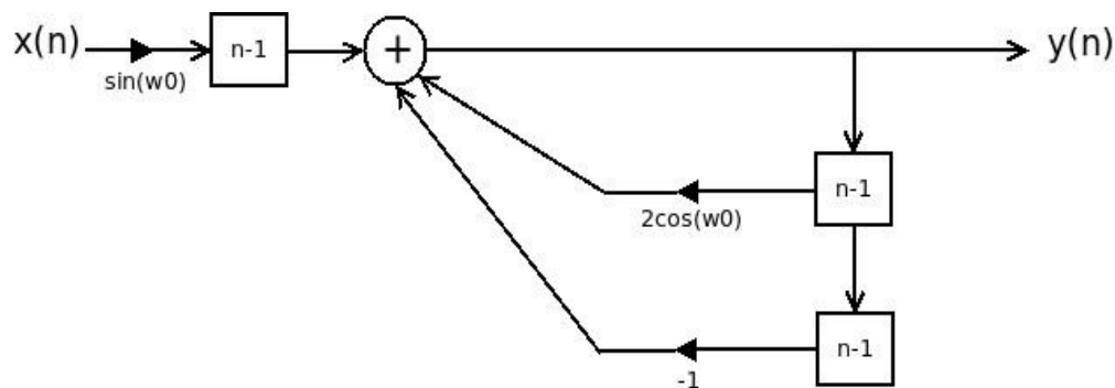
Figura 3.12: Filtro IIR para generar señales senoidales.
