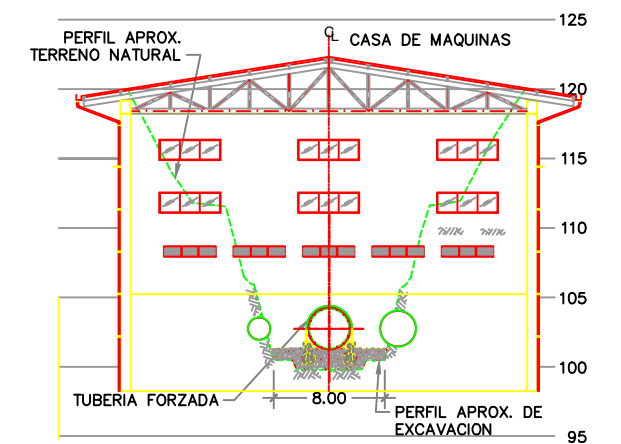
B - B
