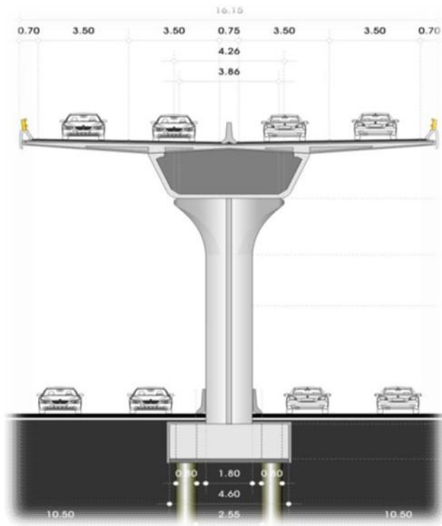
Ilustración 17. “Vista en corte de la superestructura del segundo piso de la Autopista Urbana Sur en dos carriles”
