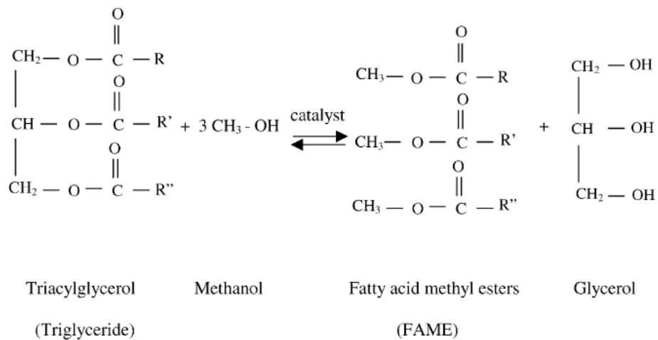
Figura 3.1 Representación esquemática del proceso de transesterificación. [16]
