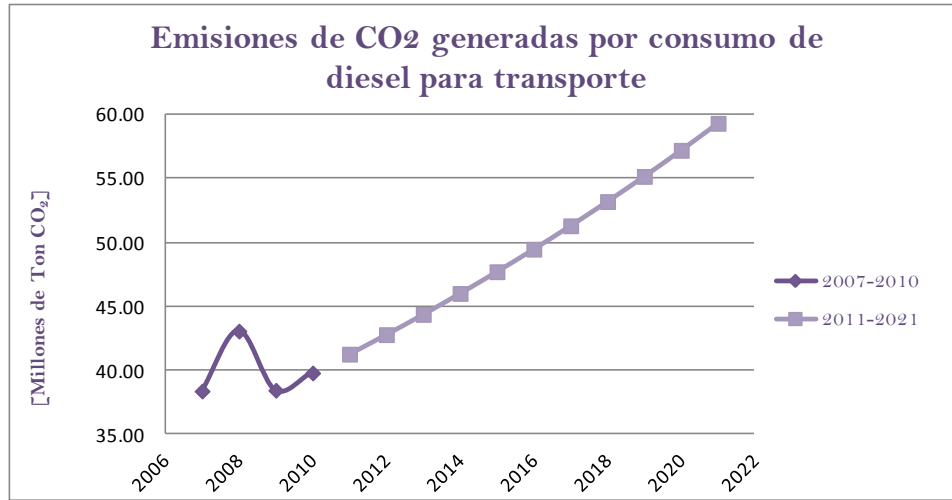
Figura 5.2 Tendencia en la generación de emisiones de CO 2 por consumo de diesel para transporte
