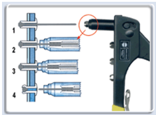
Figura 4.1 Instalación de un remache tipo pop
