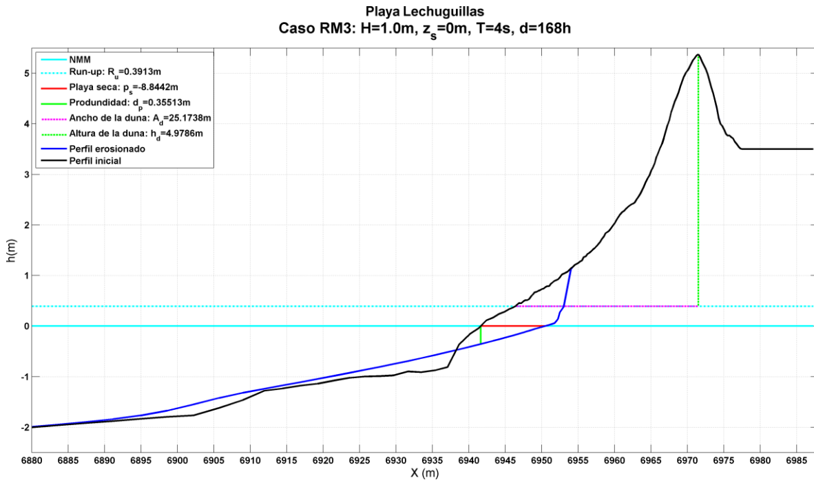
Figura V-10. Caso RM3. Recorrido de la línea de costa
