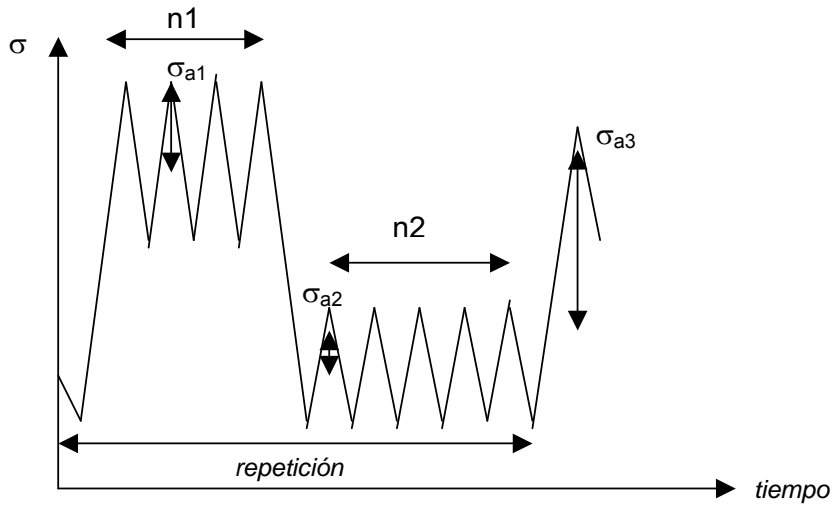
Figura 2.9. Cargas de amplitud variable
