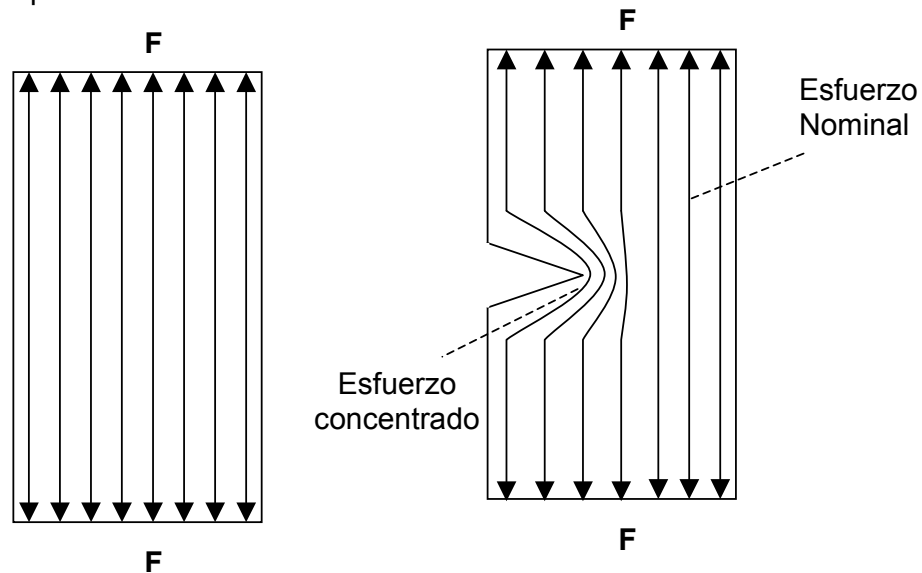
Figura 1.11 Efecto de un concentrador de esfuerzos en el flujo de carga
