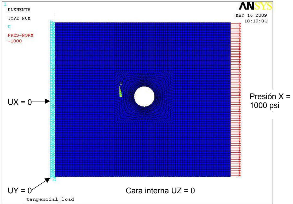
Figura 4.3 Carga Uniaxial
