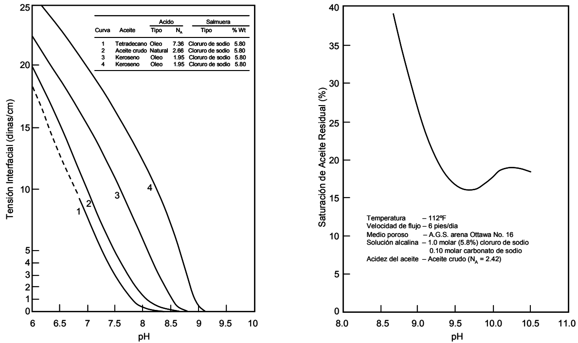
(a) Efecto del pH y salinidad sobre la tensión interfacial.
