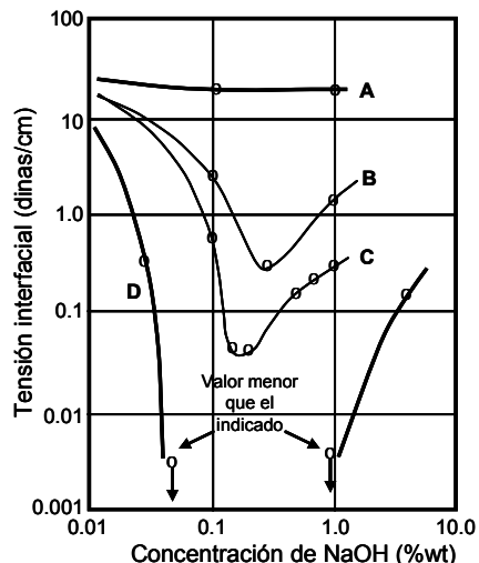
(b) Tensión interfacial vs concentración de álcali para cuatro diferentes crudos.
