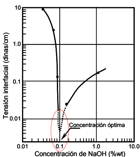
(a) Tensión interfacial vs concentración de álcali para un crudo de 12.2 °API.
