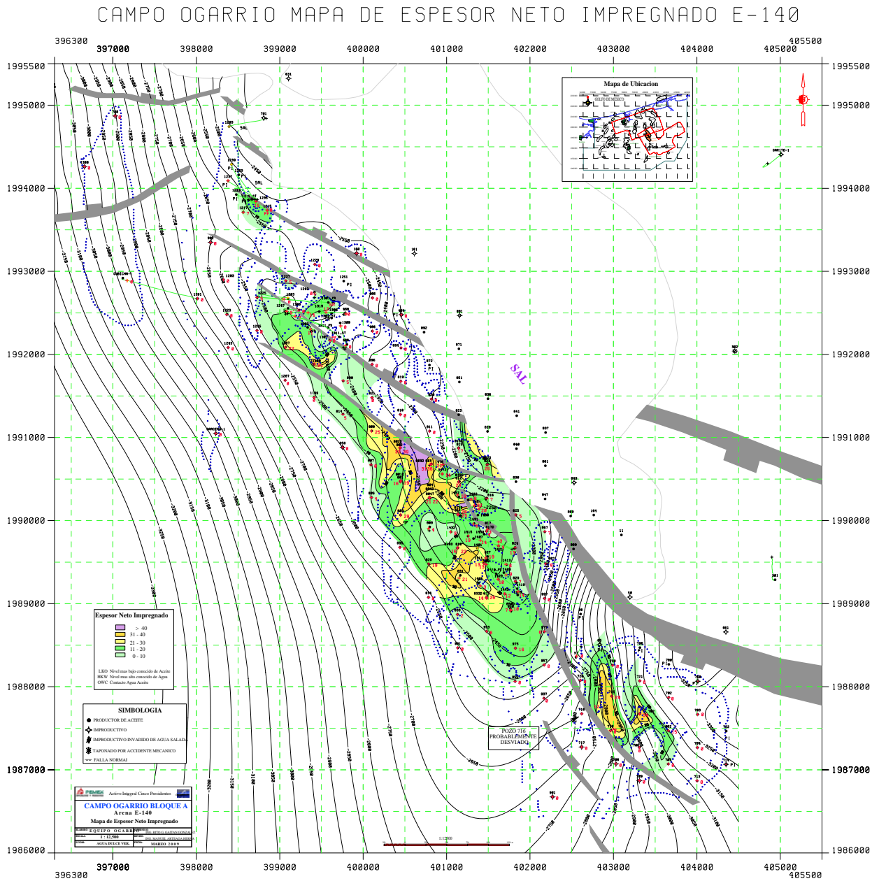
Figura A.4. Arena E_140, mapa de espesor neto impregnado Ogarrío Bloque A. 79
