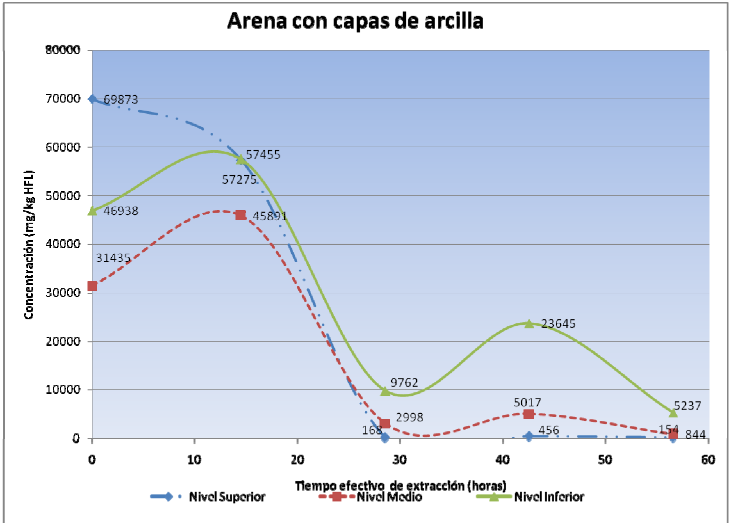
Fig. 5.2 Concentración vs el tiempo efectivo de tratamiento en la unidad experimental C1.
