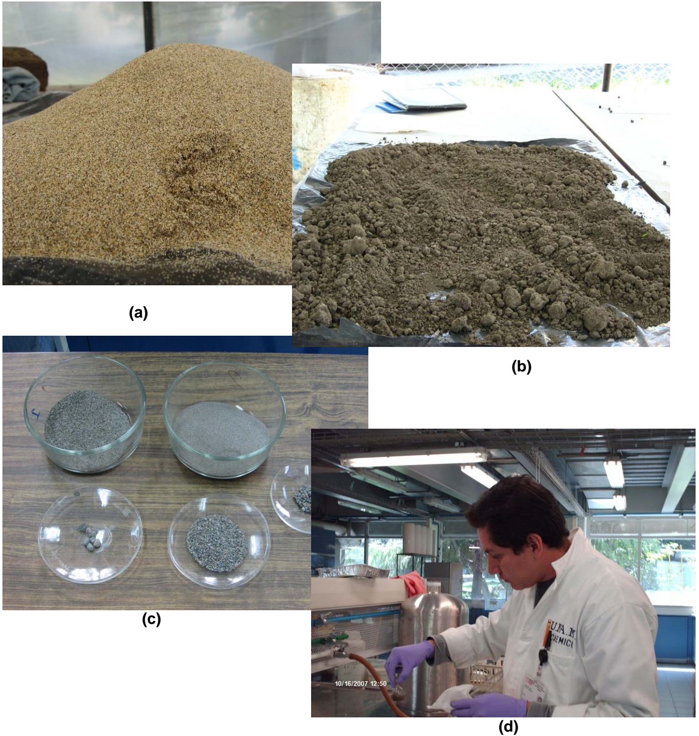
Fig. 4.14 Análisis de las propiedades del suelo. (a) suelo arenoso, (b) suelo arcilloso, (c) Análisis granulométrico y (d) determinación de densidad real.
