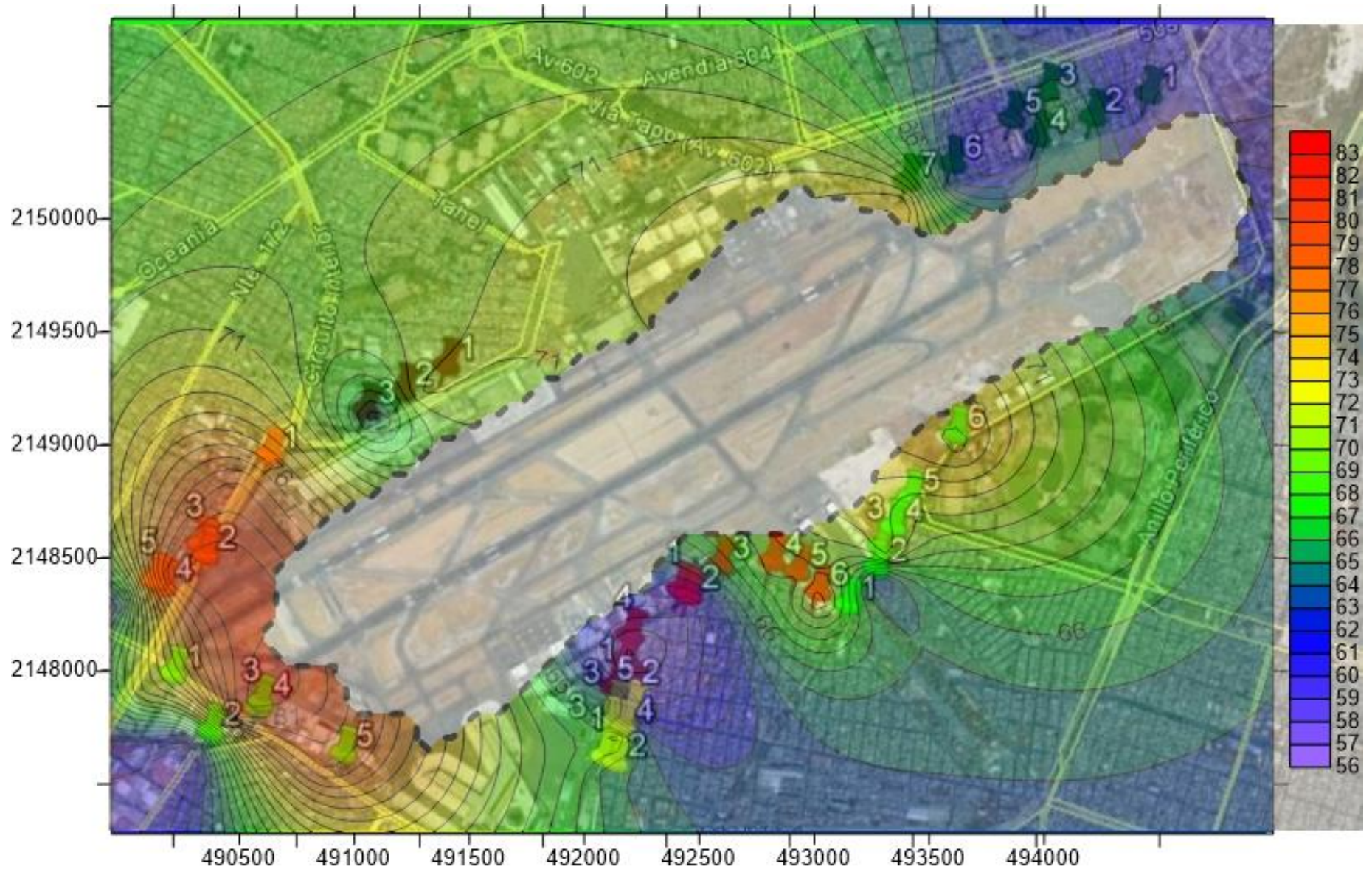
Figura 5.2 Mapa de ruido del N_{10} en los alrededores del AICM
