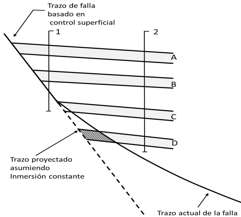
Fig. 4.1. Error en el mapeo volumétrico causado por la equivocada proyección de la falla.
