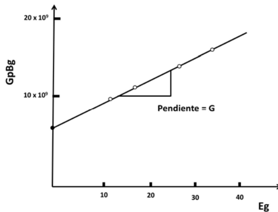
Fig. 3.7. Grafica de G_p B_g Vs. E_g . 15
