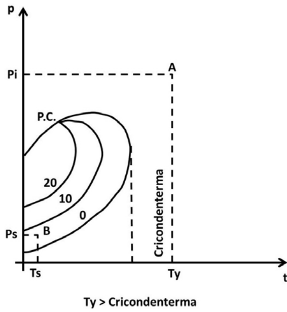
Fig. 1.7 Diagrama de fase de un yacimiento de gas húmedo. 2
