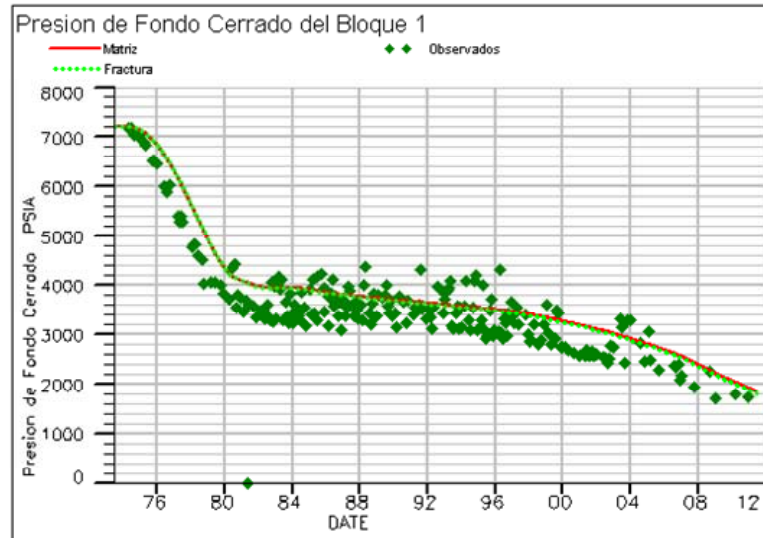
Fig. 4.3. Comportamiento de Presión del Modelo de Simulación.
