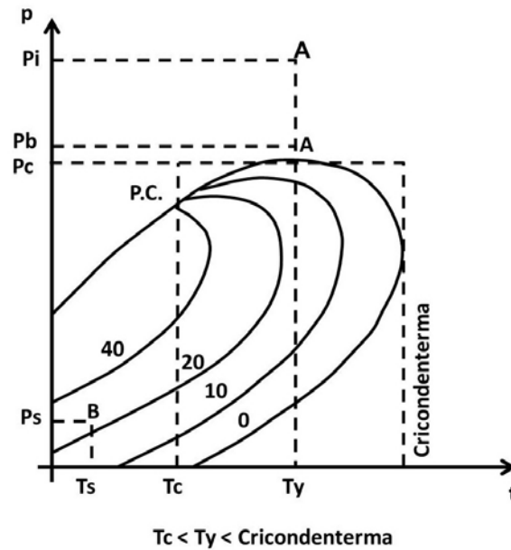
Fig. 1.6 Diagrama de fase de un yacimiento de gas y condensado. 2
