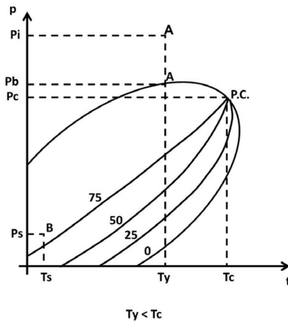
Fig. 1.4 Yacimiento de aceite y gas disuelto. 2
