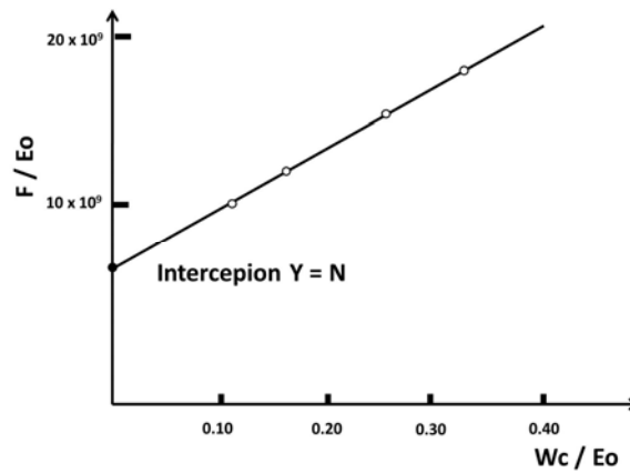
Fig. 3.6. Grafica F-E o Vs. W c - E o . 15
