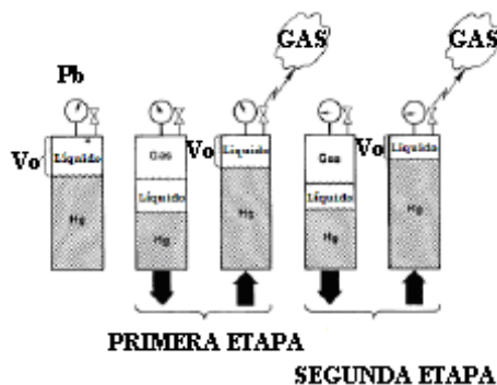
FIGURA 2.25 Liberación Diferencial
