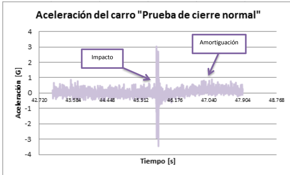
Fig. 8.20 Gráfica original de la aceleración del carro
