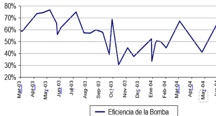
Figura 5.6 Eficiencia de la bomba de KL083.
