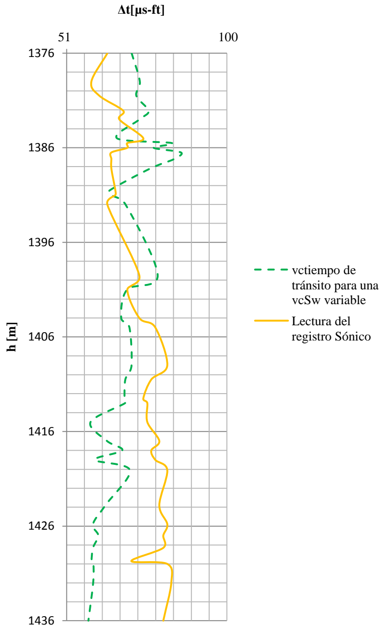
Figura 3.53. v_{c0} en términos del tiempo de tránsito al utilizar el registro sísmico de porosidad
