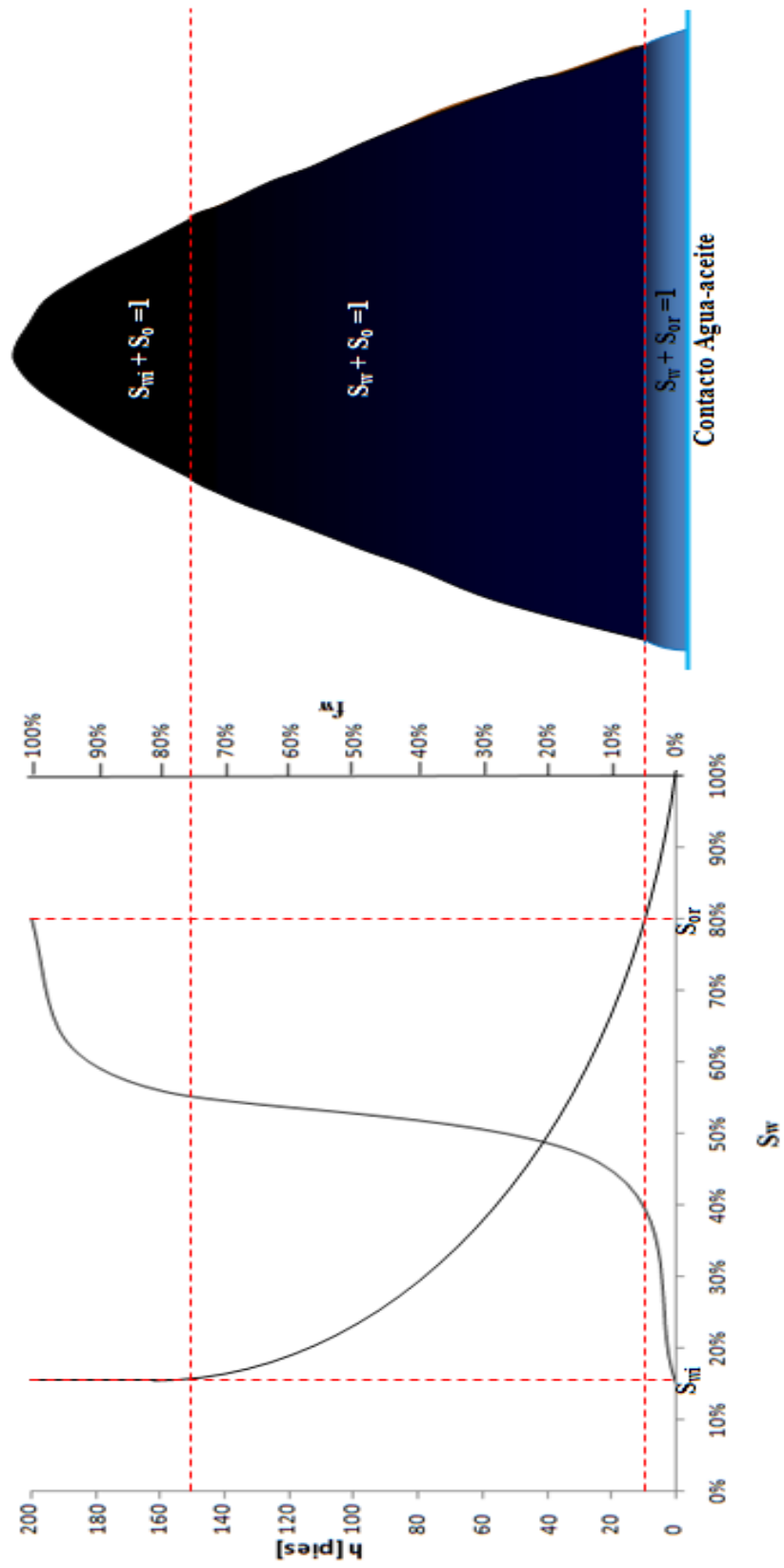
Figura 3.67. Distribución vertical de fluidos y flujo fraccional de agua en un yacimiento homogéneo
