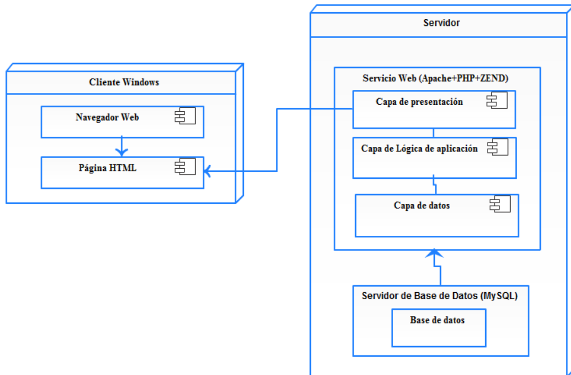
Figura 4.2 Arquitectura física del sistema de expedientes
