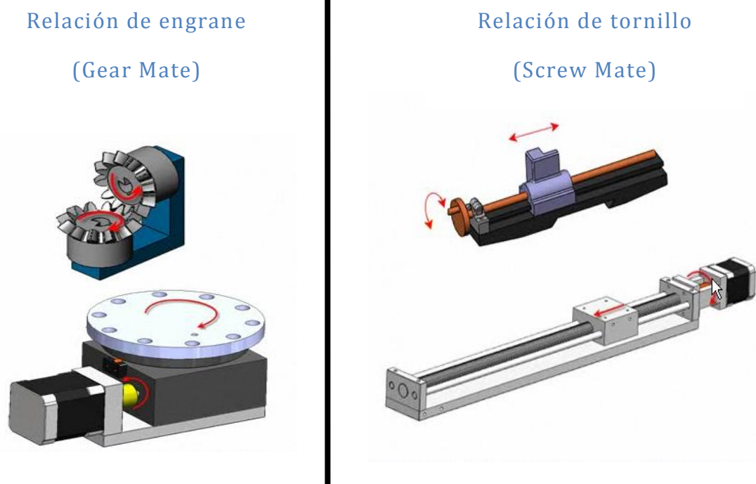
Figura 3.4 Relaciones mecánicas en un ensamblaje de CAD.
