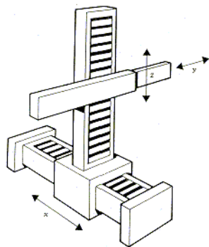
Figura 1.9 Robot Cartesiano
