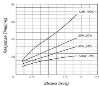
STROKE Vs RESPONSE TIME 行程 / 反應時間
