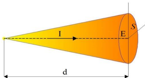
Figura 1.5 Relación entre la intensidad luminosa y la distancia hacia la superficie a iluminar
