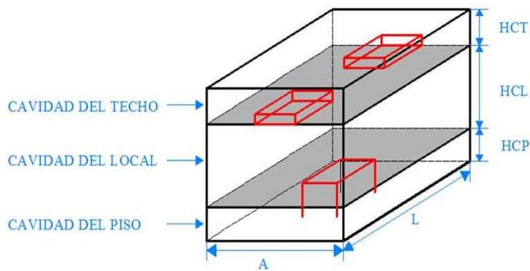
Figura 1.16 Cavidades y alturas de cavidad de un local
