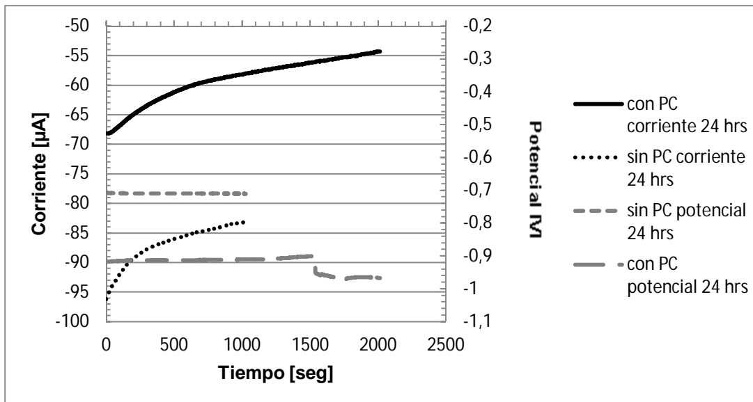
Gráfica 3.28. Serie de tiempo con y sin protección catódica. Primer día de pruebas. 25°C.
