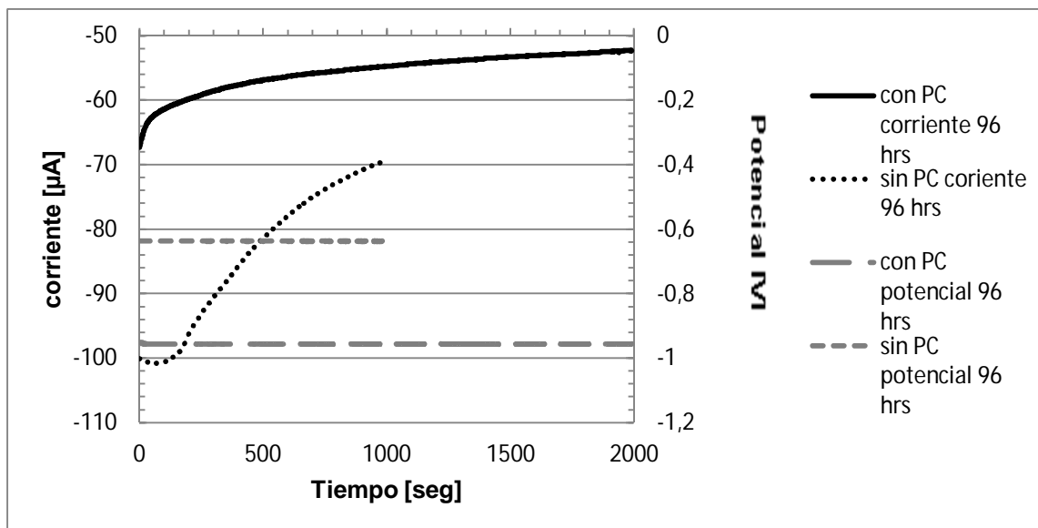
Gráfica 3.35, serie de tiempo con y sin protección catódica. Último día de pruebas. 25°C.
